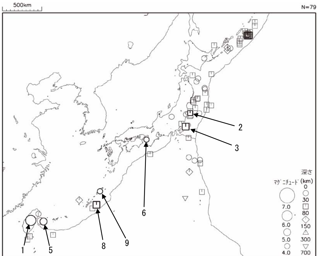
図 2 平成 25 年 6 月に発生した M4.0 以上の地震 (図中の番号は、「平成 25 年 6 月の主な地震活動」の表の番号に対応する主な地震)
