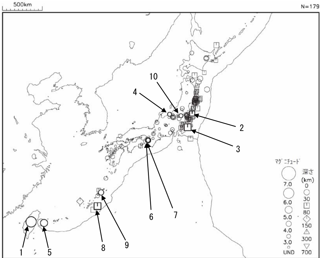
図 1 平成 25 年 6 月に震度 1 以上を観測した地震 (図中の番号は、「平成 25 年 6 月の主な地震活動」の表の番号に対応する主な地震)
