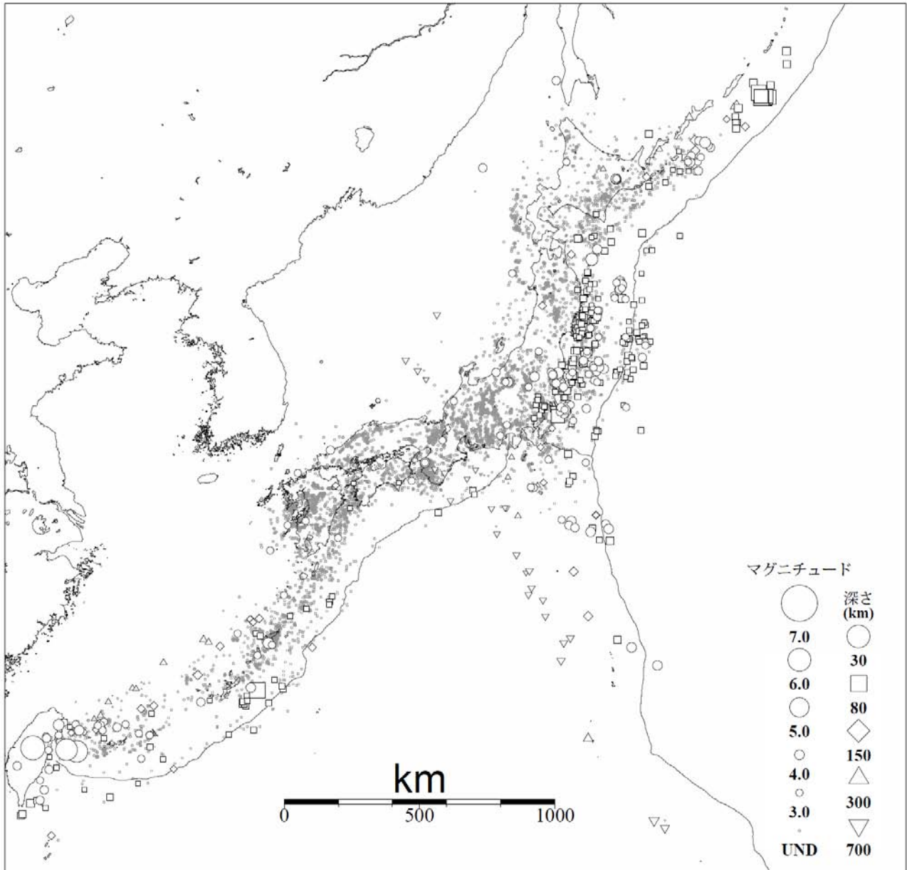
図3 気象庁が震源を決定した日本付近の平成 25 年 6 月の地震の震央分布 (M3.0 以上の地震については白抜きで示す)
