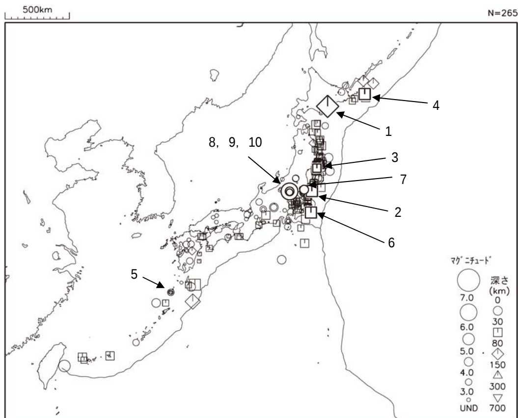
図 1 平成 25 年 2 月に震度 1 以上を観測した地震 (図中の番号は、「平成 25 年 2 月の主な地震活動」の表の番号に対応する主な地震)
