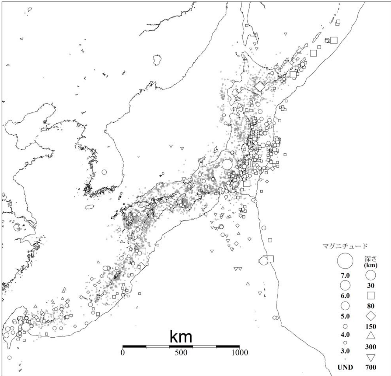
図3 気象庁が震源を決定した日本付近の平成25年2月の地震の震央分布 (M3.0以上の地震については白抜きで示す)
