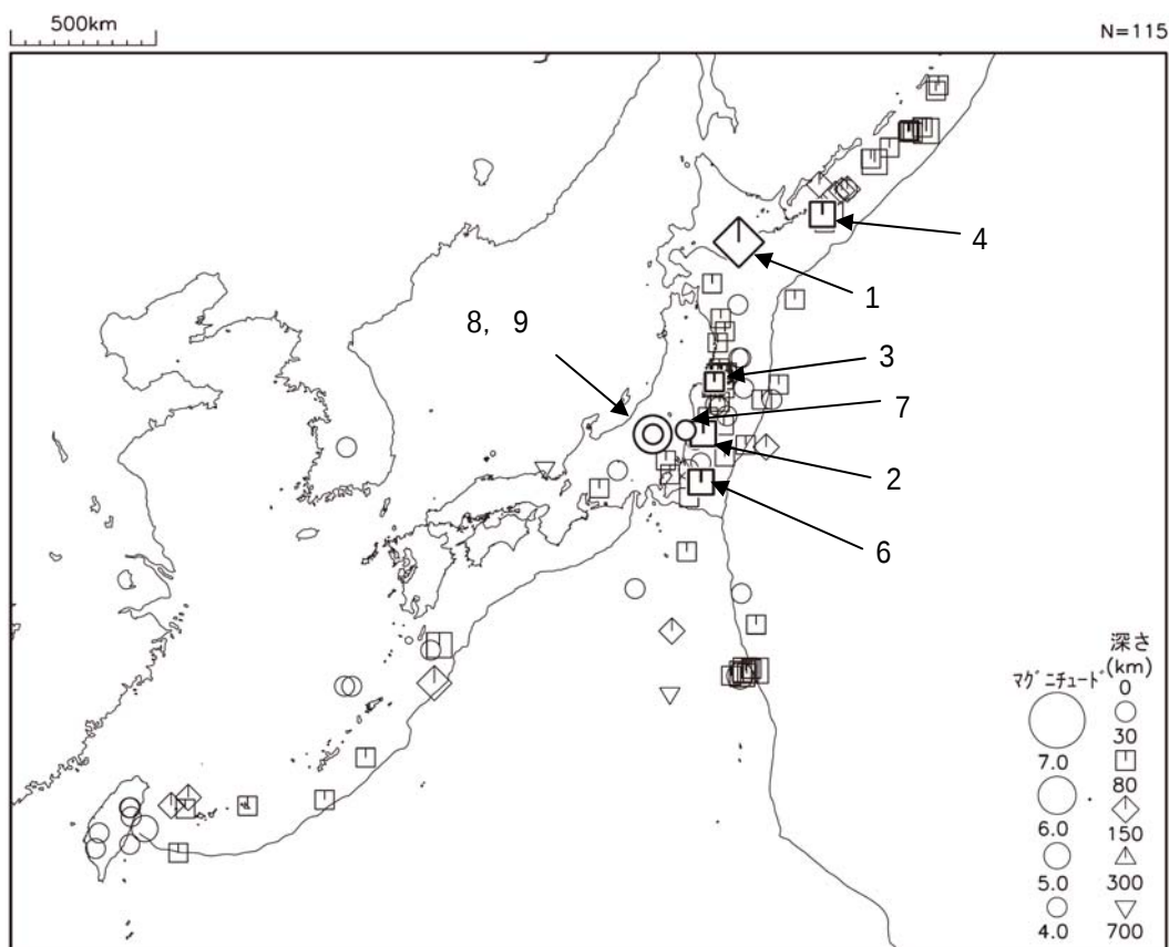
図 2 平成 25 年 2 月に発生した M4.0 以上の地震 (図中の番号は、「平成 25 年 2 月の主な地震活動」の表の番号に対応する主な地震)
