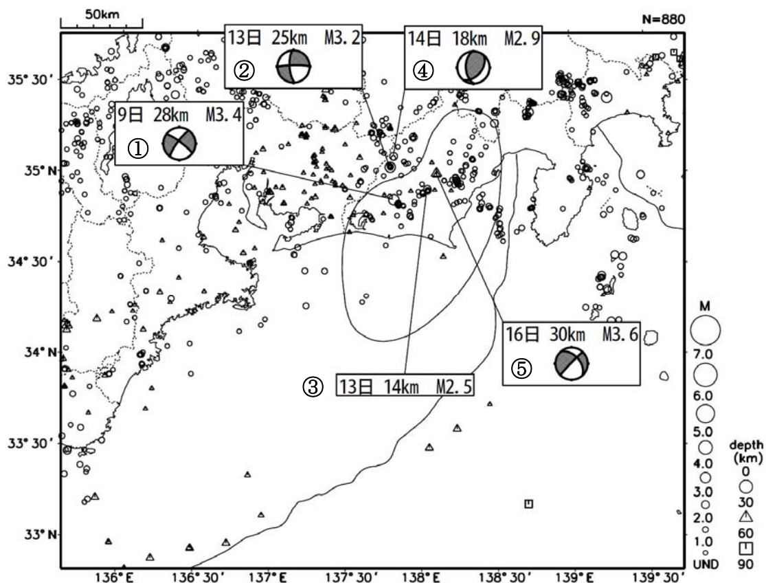
図1 震央分布図(2012年9月1日～30日:深さ0～90km、Mすべて。図中のナス型の領域は東海地震の想定震源域。)
