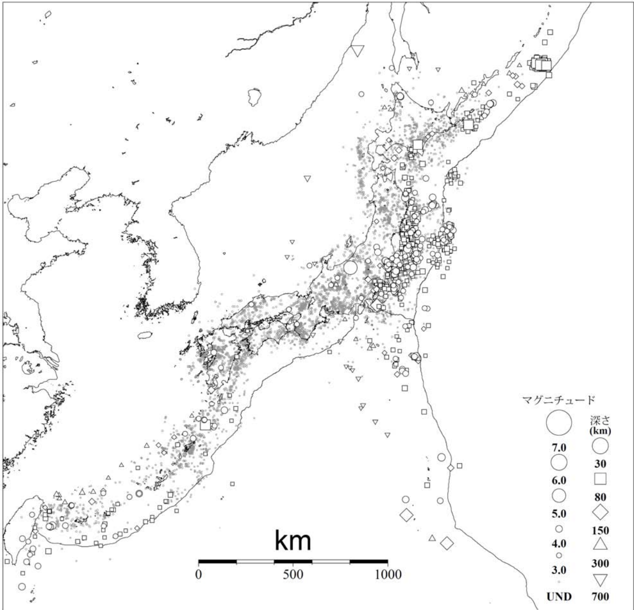
図3 気象庁が震源を決定した日本付近の平成24年7月の地震の震央分布 (M3.0以上の地震については白抜きで示す)
