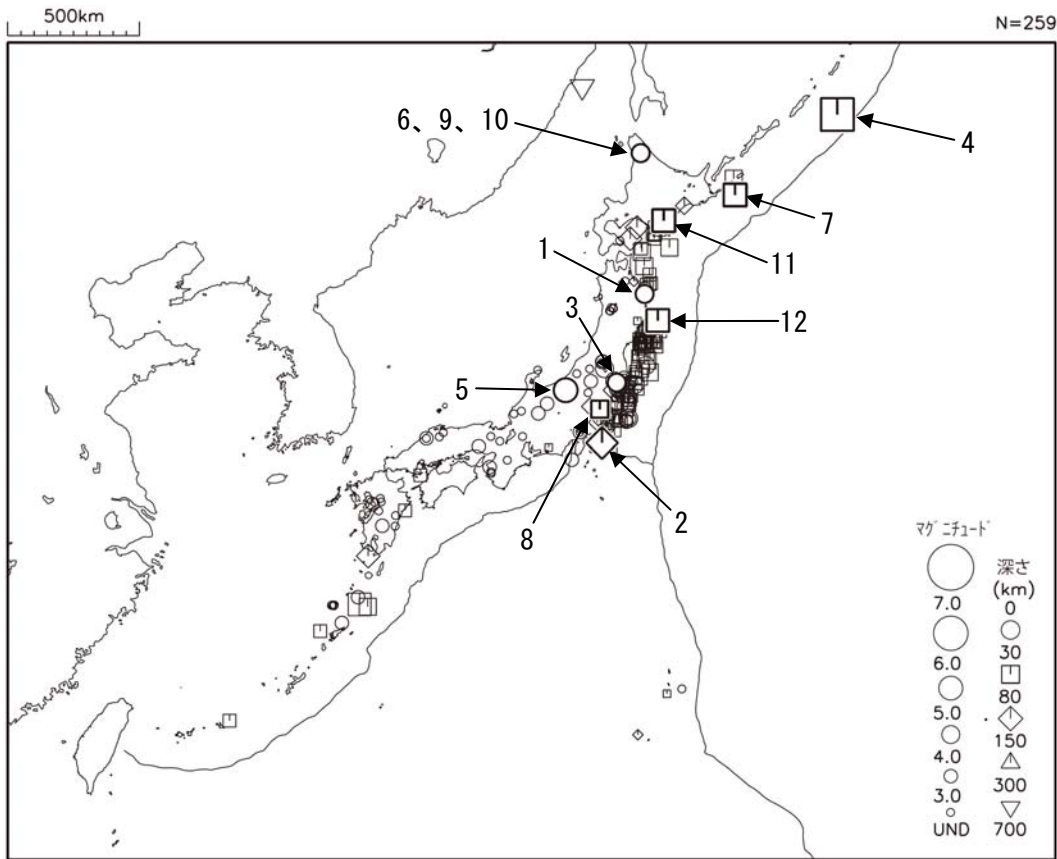
図 1 平成 24 年 7 月に震度 1 以上を観測した地震 (図中の番号は、「平成 24 年 7 月の主な地震活動」の表の番号に対応する主な地震)
