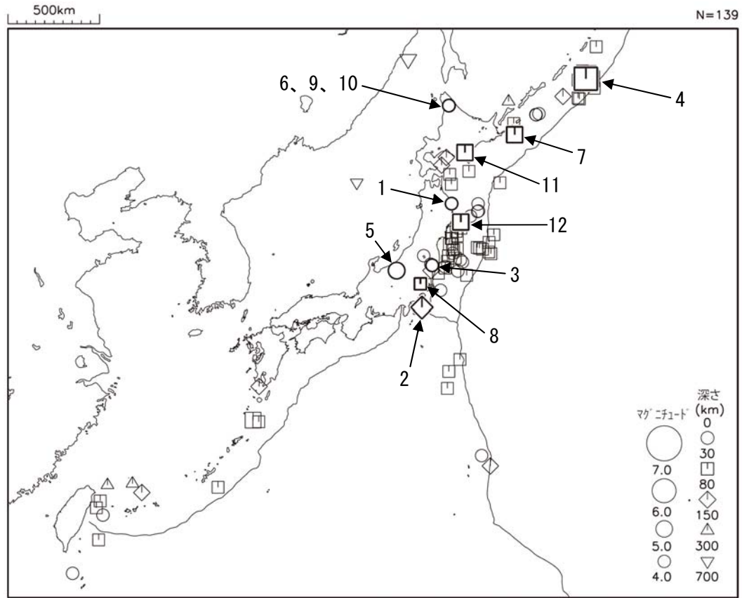
図 2 平成 24 年 7 月に発生した M4.0 以上の地震 (図中の番号は、「平成 24 年 7 月の主な地震活動」の表の番号に対応する主な地震)
