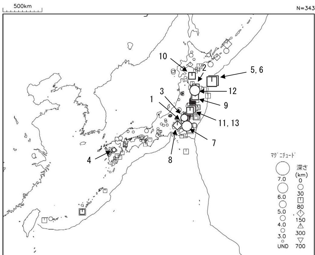
図 1 平成 24 年 3 月に震度 1 以上を観測した地震 (図中の番号は、3 ページの表の番号に対応する主な地震)
