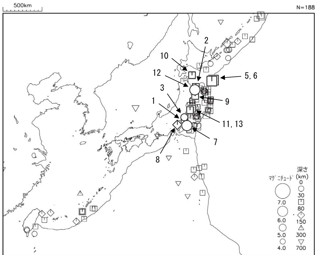
図 2 平成 24 年 3 月に発生した M4.0 以上の地震 (図中の番号は、3 ページの表の番号に対応する主な地震)
