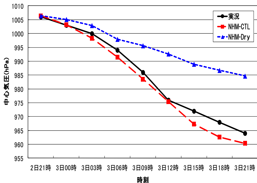
低気圧の中心気圧の時系列
