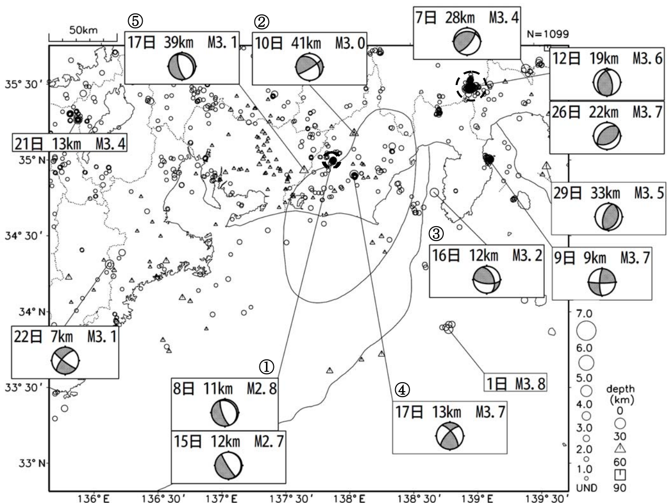
図1 震央分布図(2012年2月1日～29日:深さ0～90km、Mすべて。図中のナス型の領域は東海地震の想定震源域。)
