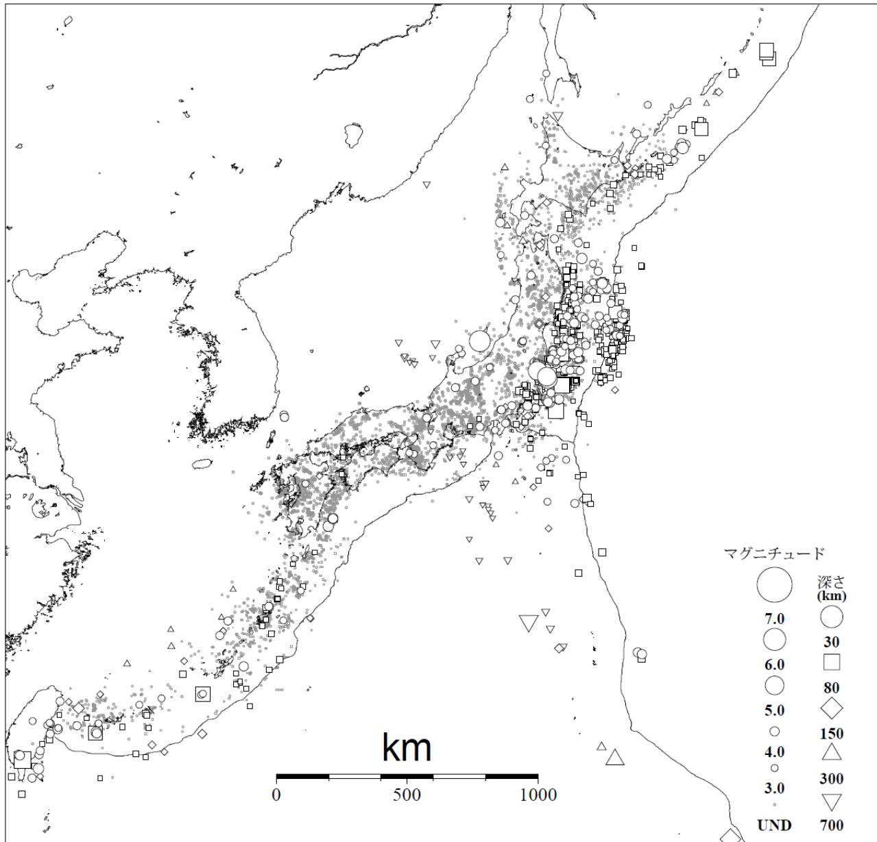
図3 気象庁が震源を決定した日本付近の平成24年2月の地震の震央分布 (M3.0以上の地震については白抜きで示す)
