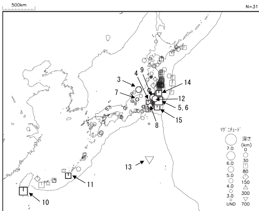
図 1 平成 24 年 2 月に震度 1 以上を観測した地震 (図中の番号は、3 ページの表の番号に対応する主な地震)
