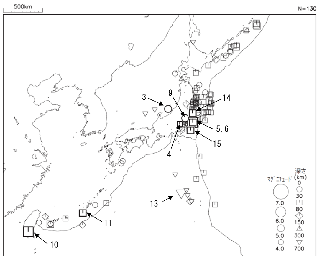
図 2 平成 24 年 2 月に発生した M4.0 以上の地震 (図中の番号は、3 ページの表の番号に対応する主な地震)
