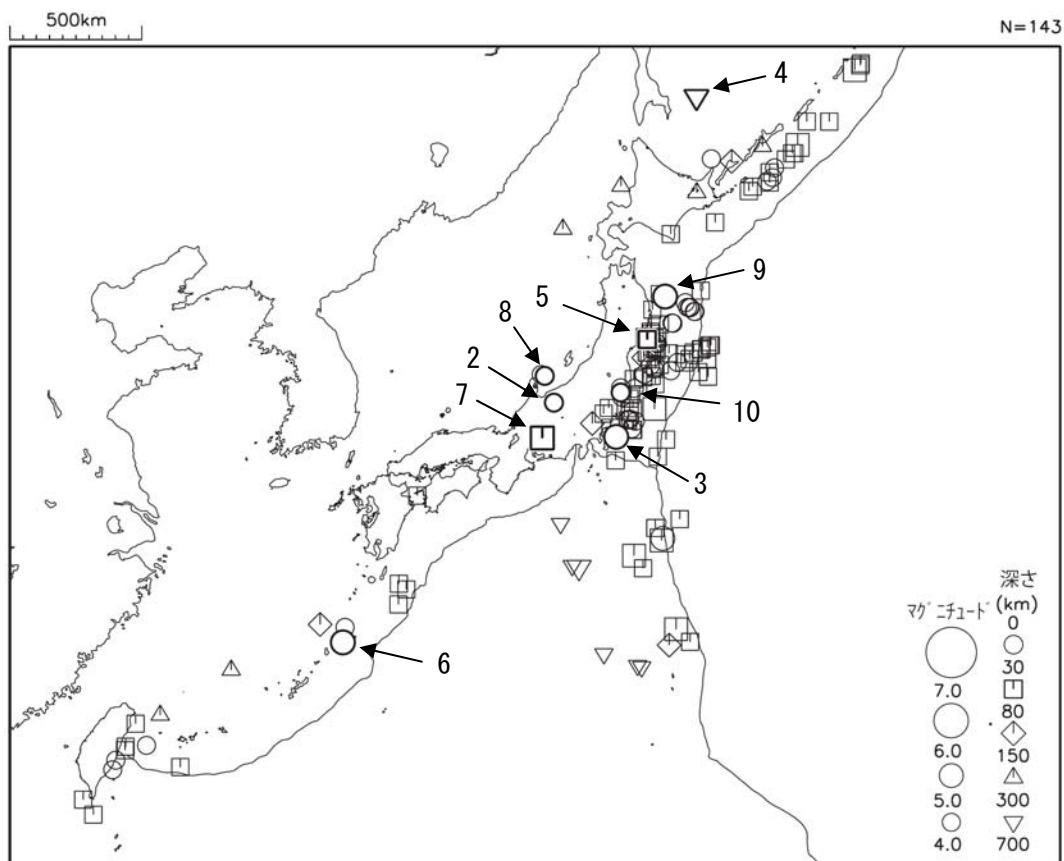
図 2 平成 23 年 12 月に発生した M4.0 以上の地震 (図中の番号は、3 ページの表の番号に対応する主な地震)
