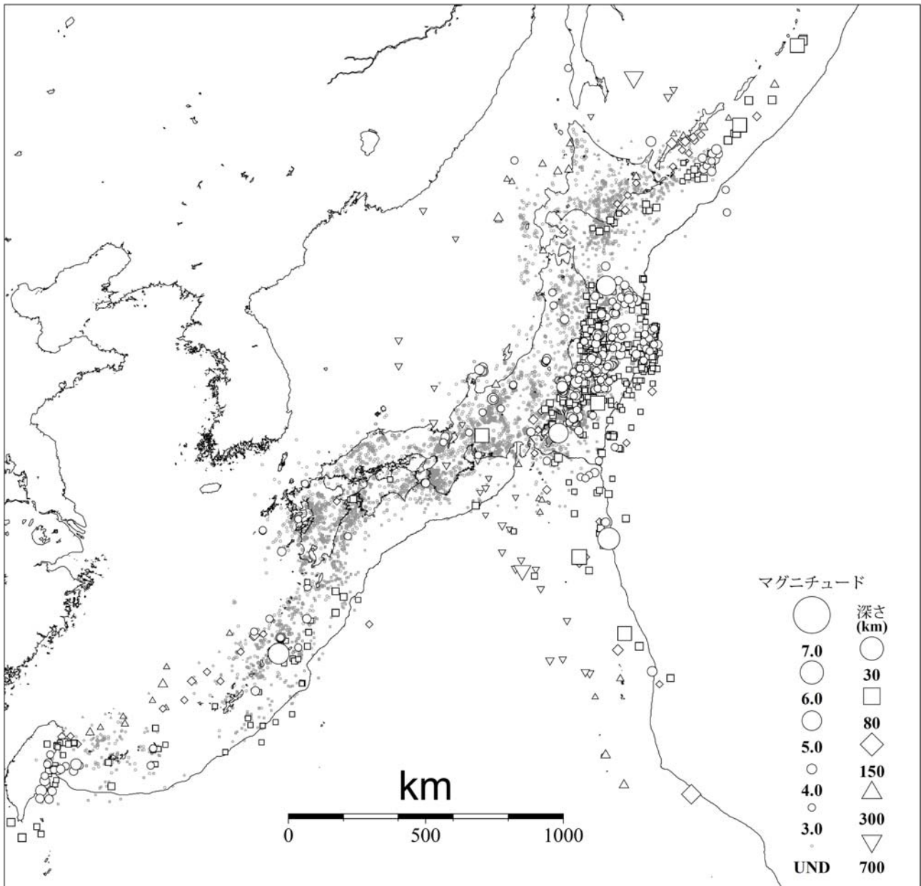
図3 気象庁が震源を決定した日本付近の平成23年12月の地震の震央分布 (M3.0以上の地震については白抜きで示す)
