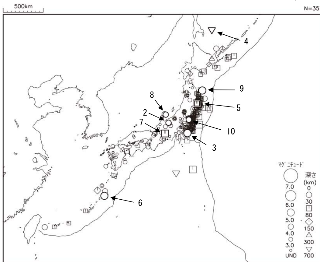
図 1 平成 23 年 12 月に震度 1 以上を観測した地震 (図中の番号は、3 ページの表の番号に対応する主な地震)
