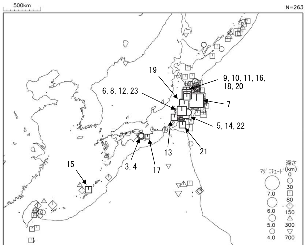
図2 平成23年7月に発生したM4.0以上の地震 (図中の番号は、4ページの表の番号に対応する主な地震)
