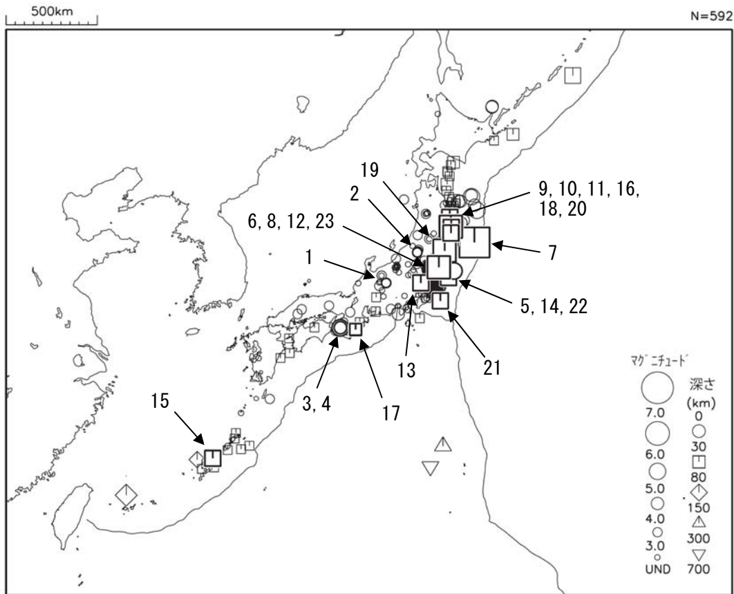
図1 平成23年7月に震度1以上を観測した地震 (図中の番号は、4ページの表の番号に対応する主な地震)
