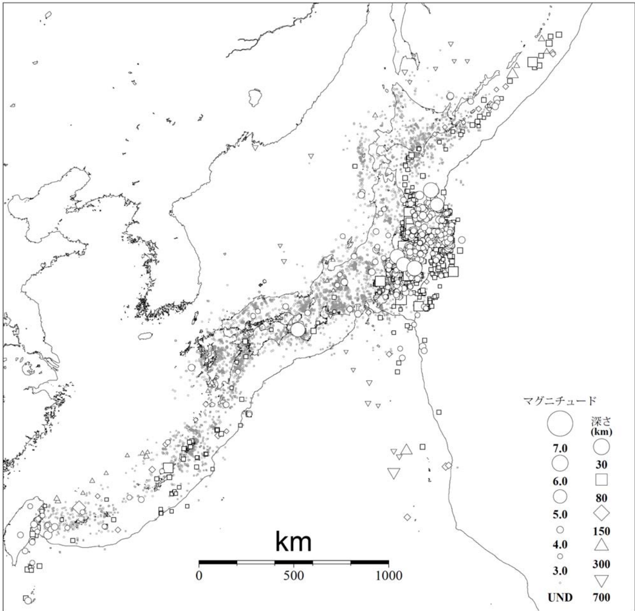
図3 気象庁が震源を決定した日本付近の平成23年7月の地震の震央分布 (M3.0以上の地震については白抜きで示す)
