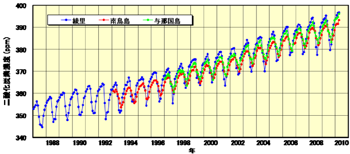
図：綾里、南鳥島および与那国島における大気中二酸化炭素月平均濃度の経年変化（ppm:百万分の一）
