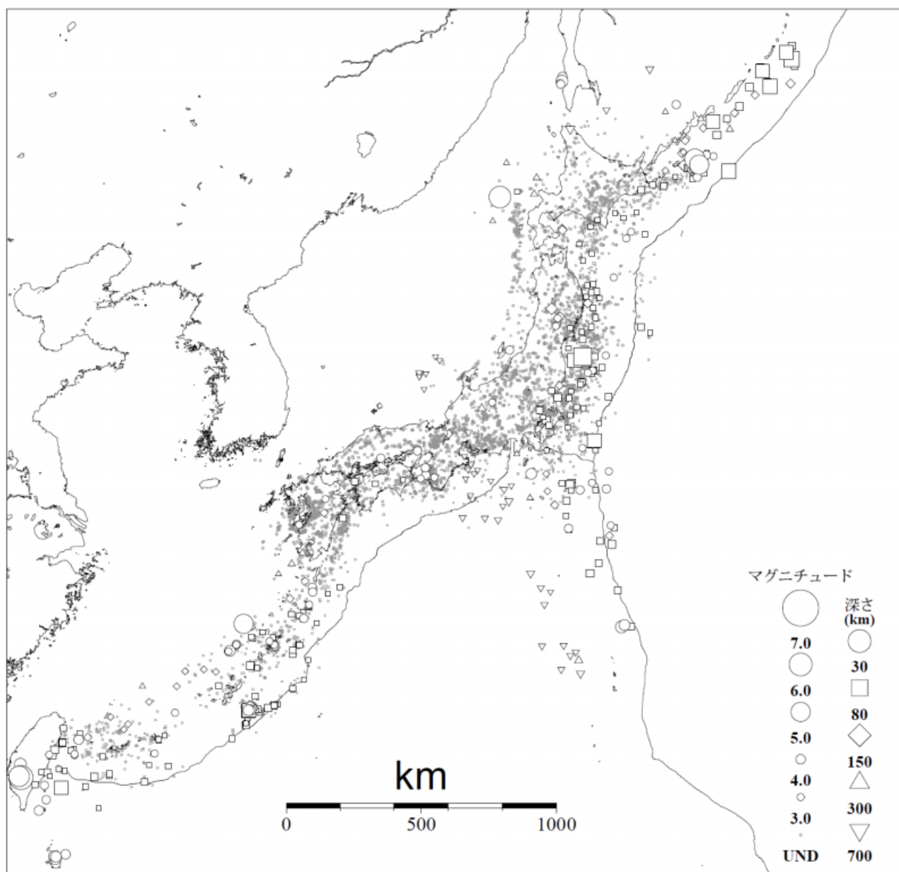
図3 気象庁が震源を決定した日本付近の平成22年3月の地震の震央分布 (M3.0以上の地震については白抜きで示す)
