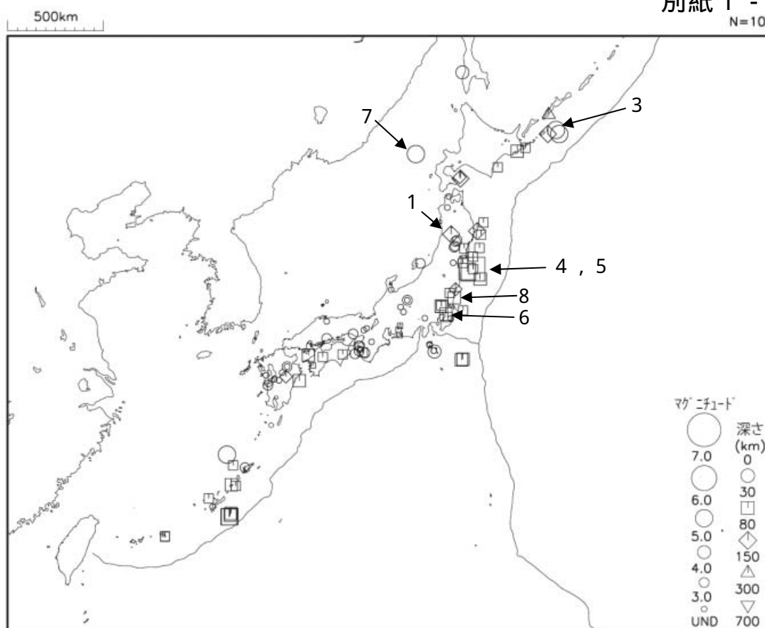
図1 平成 22 年 3 月に震度 1 以上を観測した地震 (図中の番号は、2 ページの表の番号に対応する地震)
