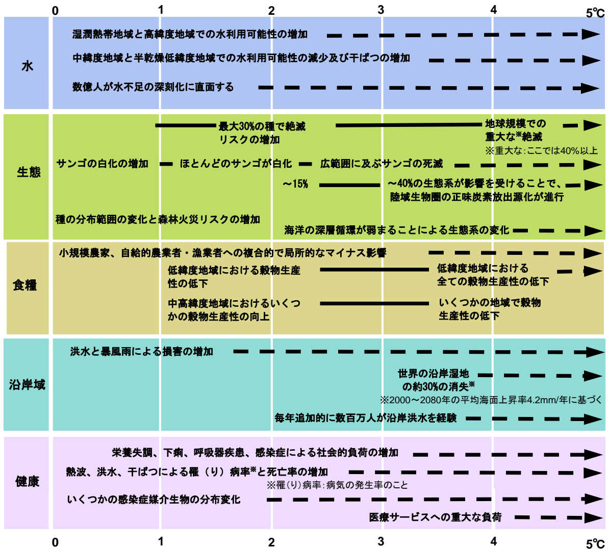
1980-1999年に対する世界年平均気温の変化
