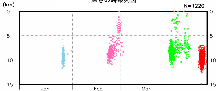
深さの時系列図
