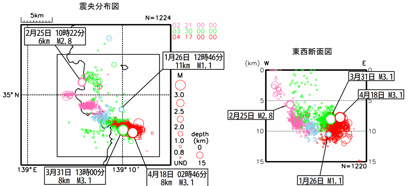
地震活動経過図、回数積算図
