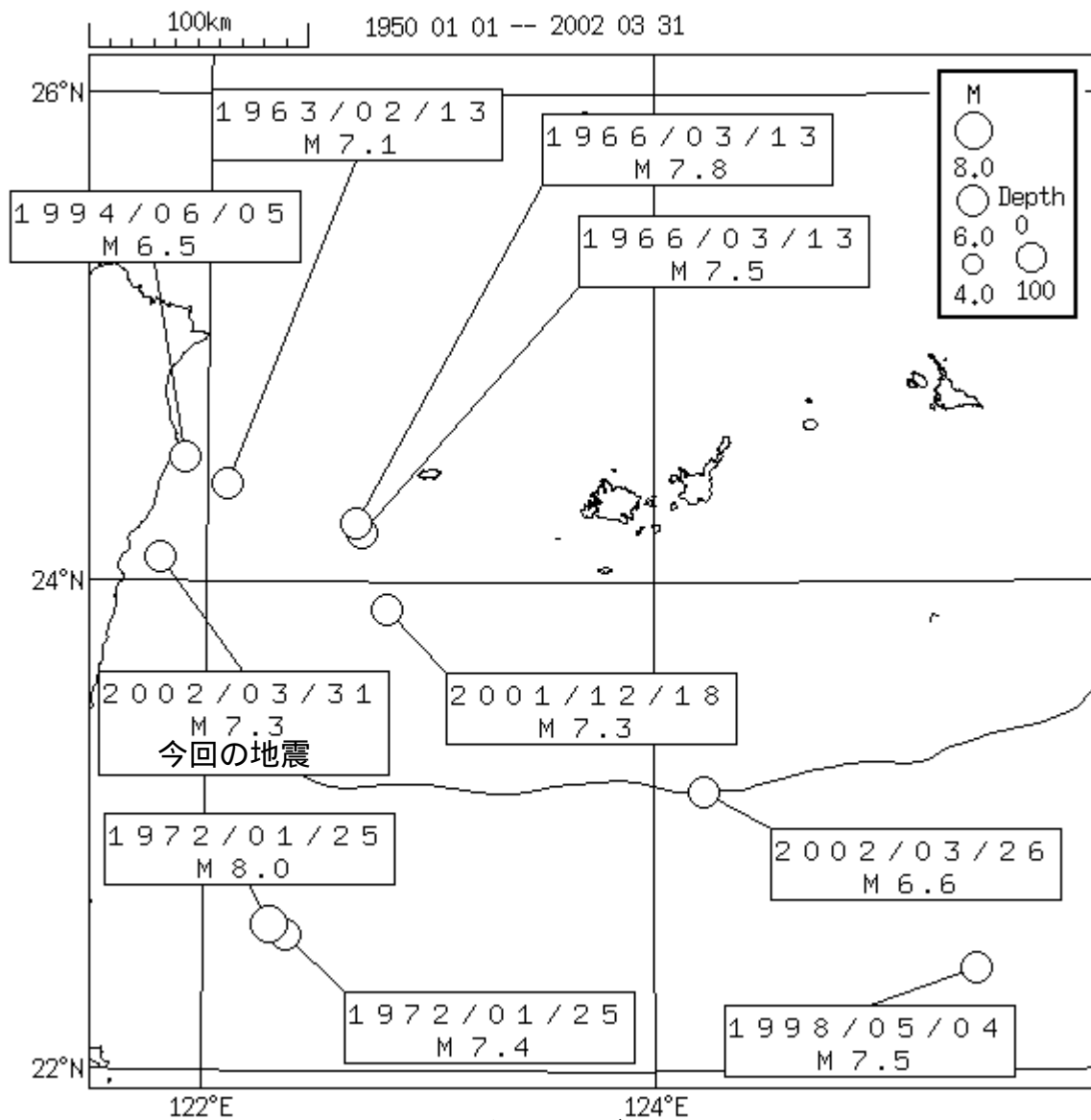
図 過去の津波を伴った地震 1900~2002年(宇津のデータによる)
