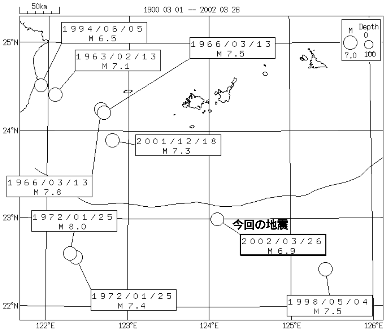
図 過去の津波を伴った地震 1900～2001年(宇津のデータによる)
