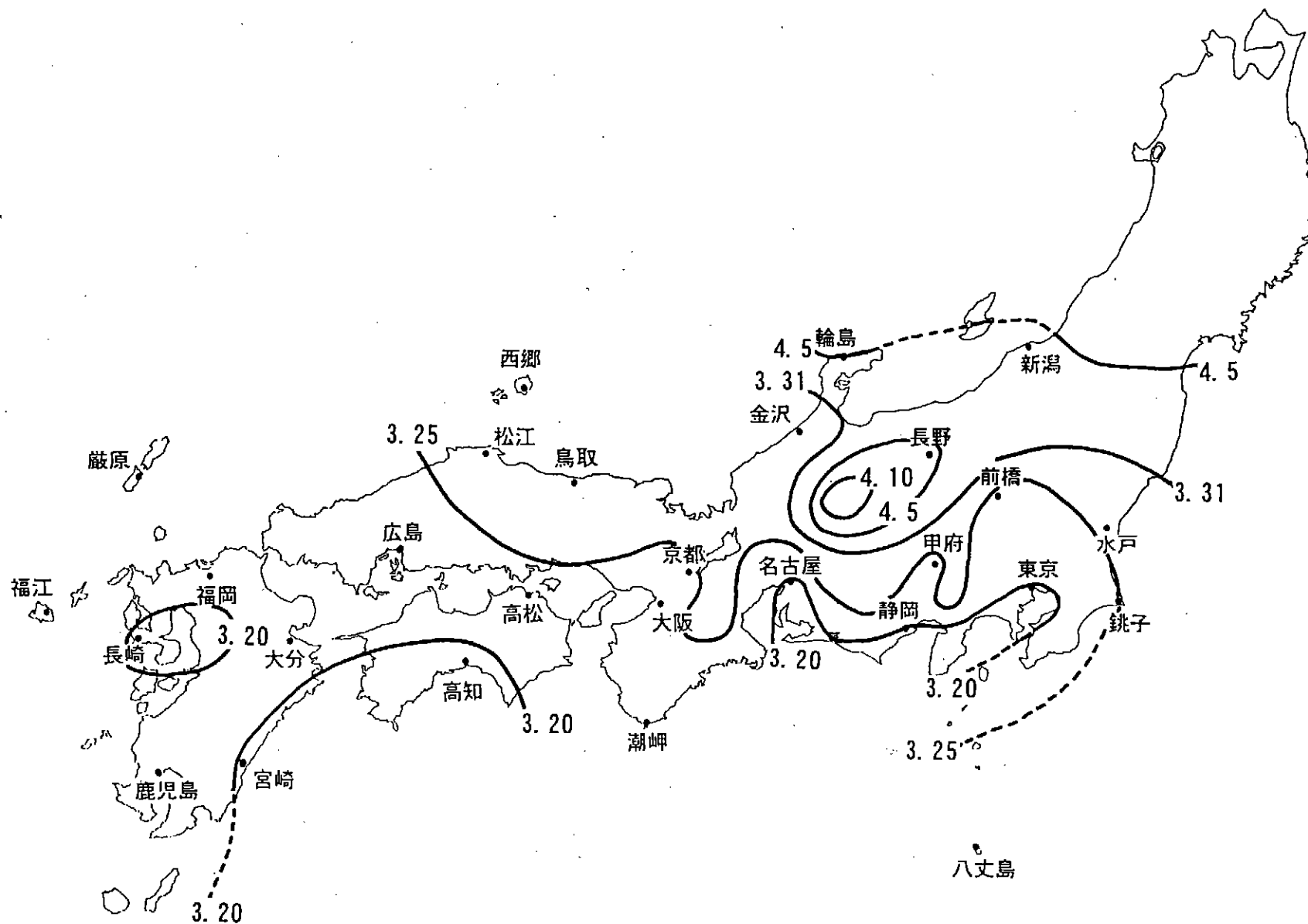
資料2 2002年さくらの開花予想の等期日線図 (東日本, 西日本)
