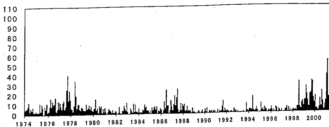
図2 吾妻山月別地震回数(1974.01.01~2001.05.14、S-P2秒以下)
