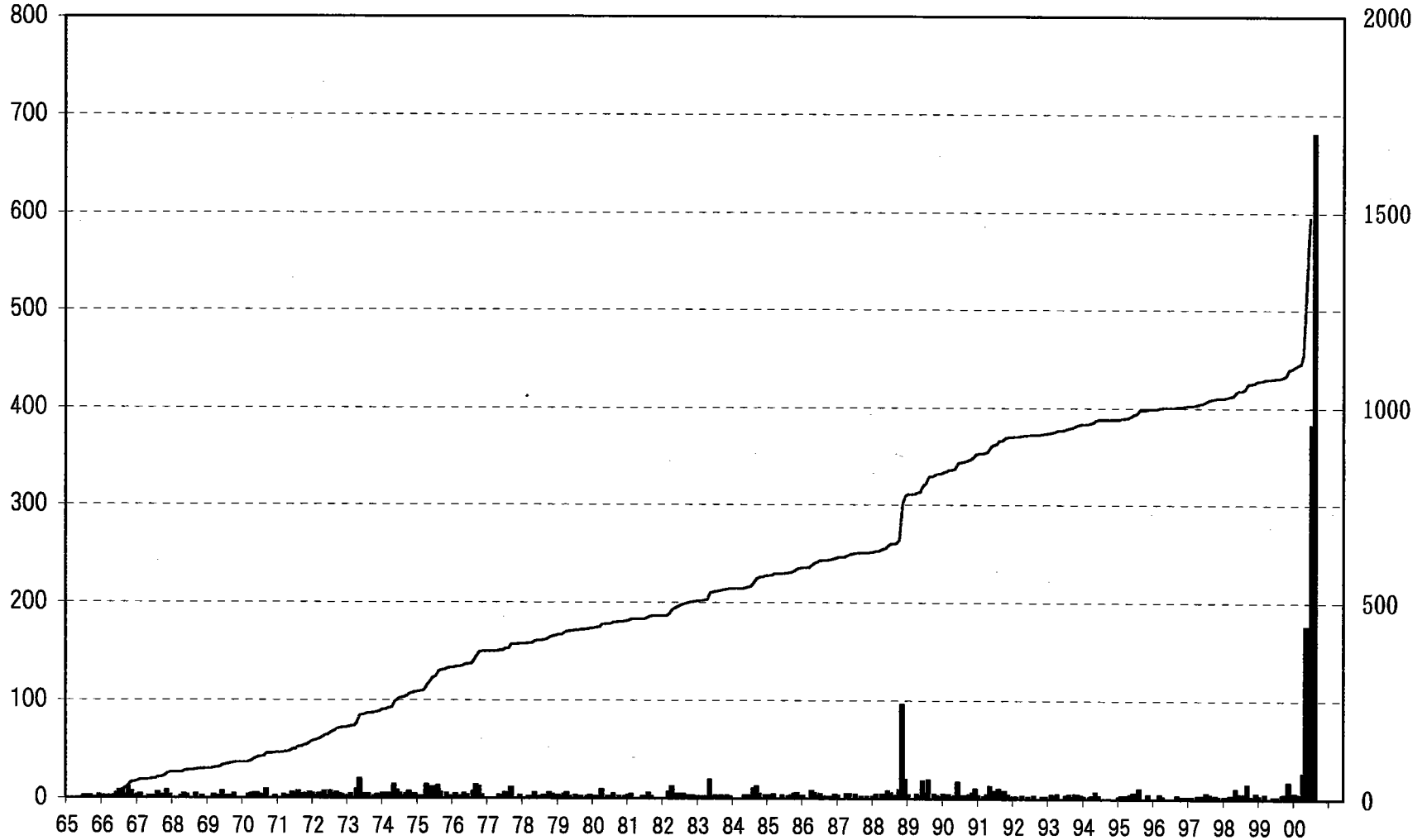
磐梯山で観測した月別地震回数 (1965-2000年)
