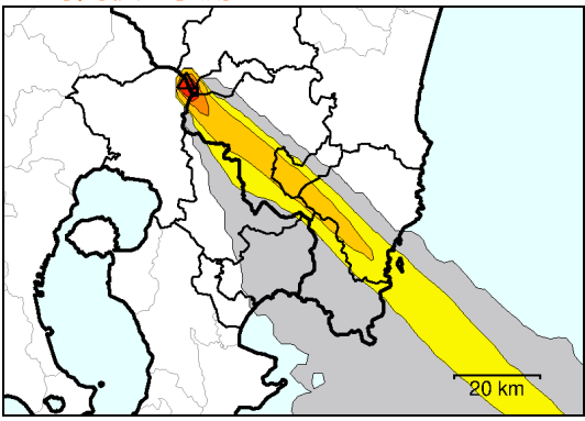
6時間後の予測
