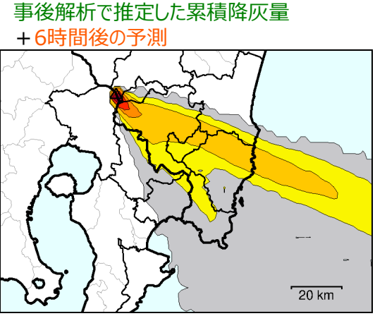
累積降灰量を発表基準とした場合
