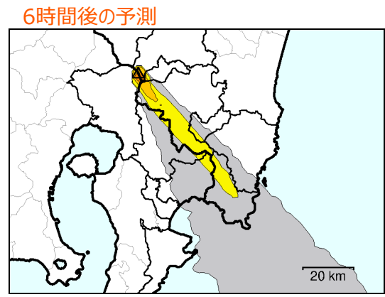
予測降灰量を発表基準とした場合
