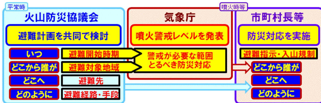
図 14 火山防災協議会、噴火警戒レベル、避難計画の関係(活動火山対策特別措置法に基づき気象庁にて作成)
