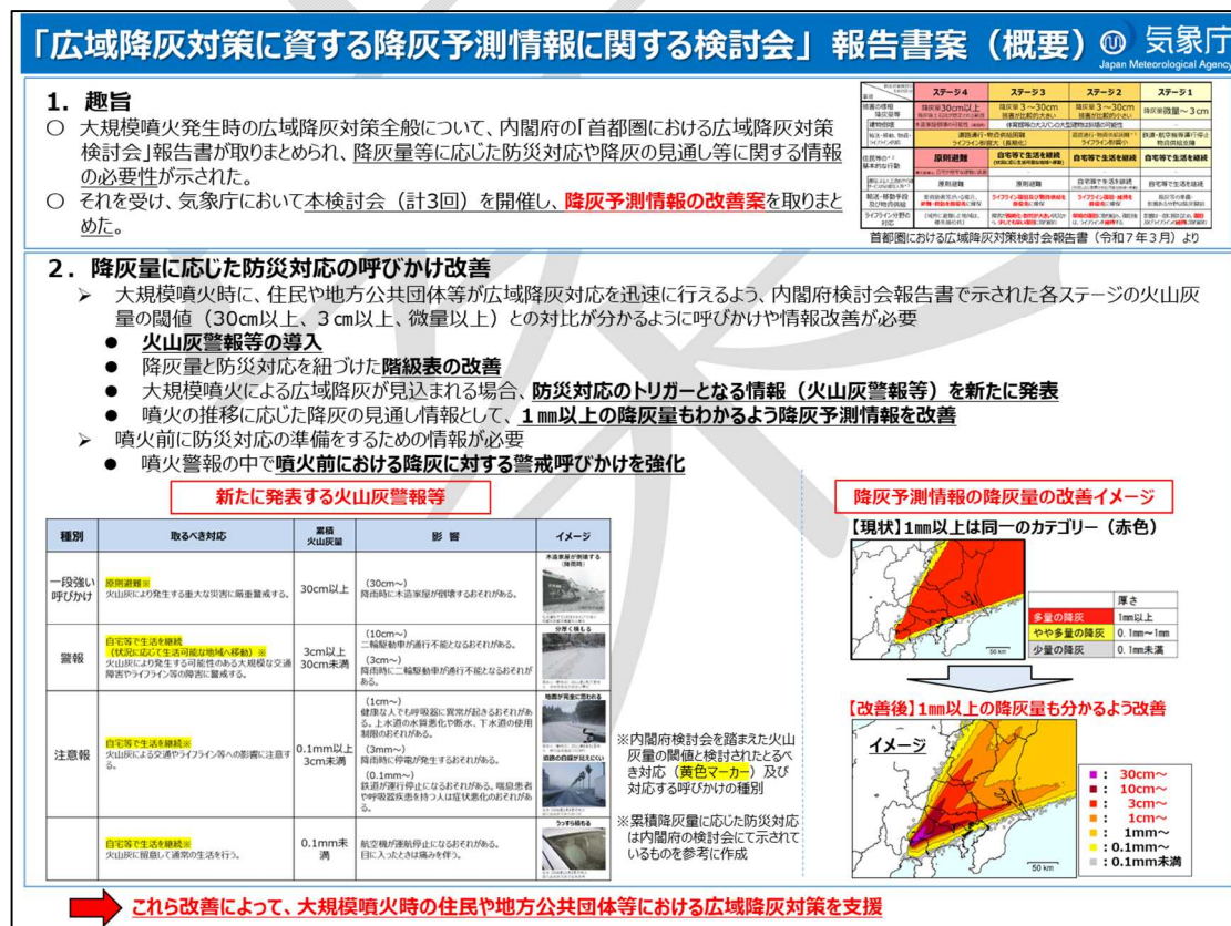
図 17 気象庁検討会報告書案の概要
