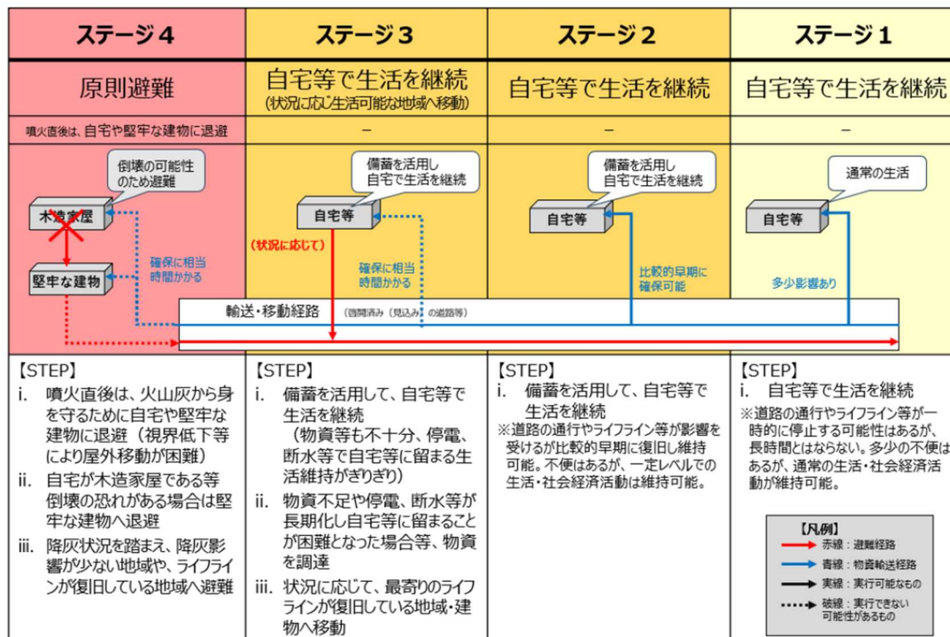
図 10 被害の様相に応じた対応手順の概要 内閣府検討会報告書(令和7年3月)
