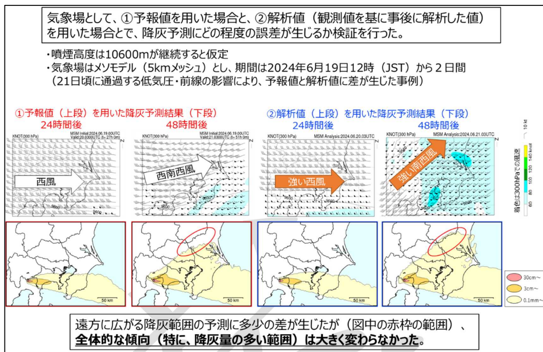
図7 気象データの違いによる降灰予報の誤差
