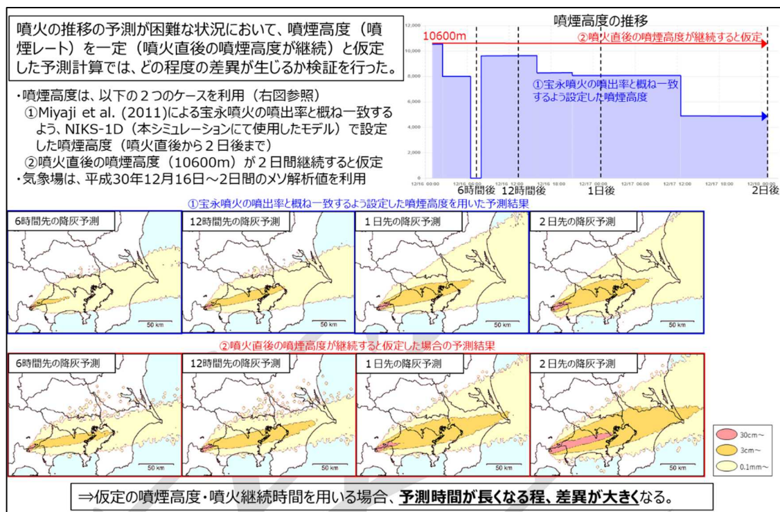
図6 6 大規模噴火における噴煙量（噴煙高度・噴火継続時間の設定の違いによる差異）
