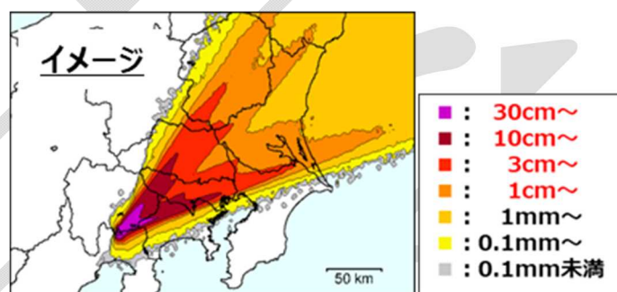
図 16 大規模噴火発生時の噴火の推移に応じた降灰の見通しの情報のイメージ
