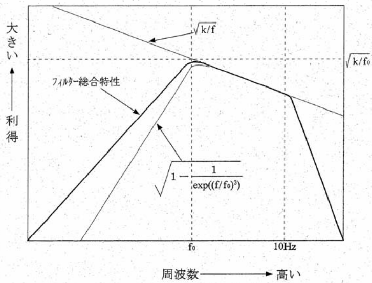
図1 フィルターの総合特性（両対数スケール）
