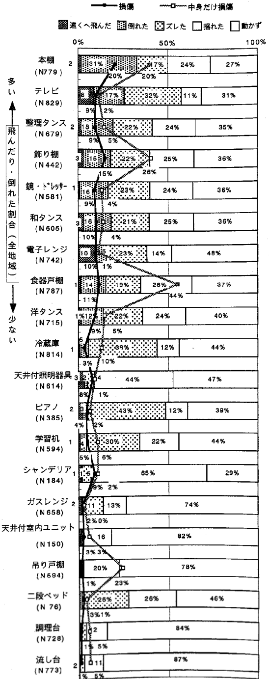
図 7-2 家具・設備機器の移動と被害
