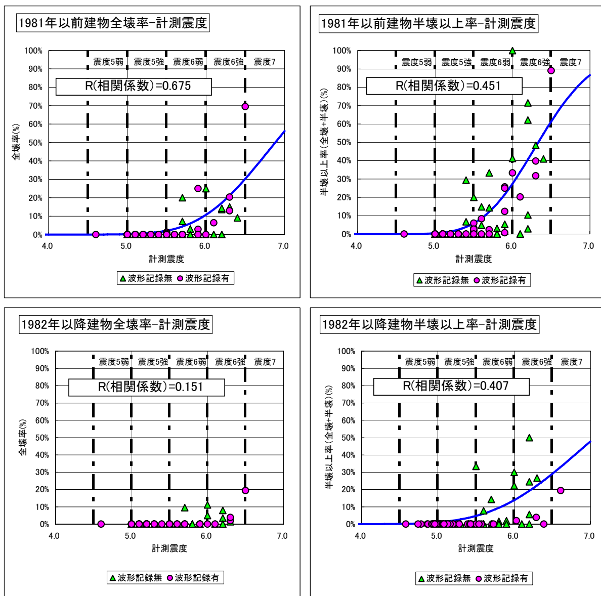
図 木造被害率(罹災証明データ)と計測震度の関係 (波形データ有+無)
