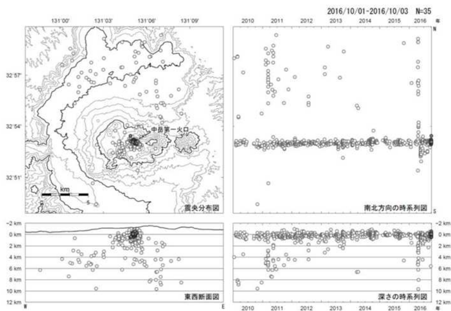
図 2 阿蘇山 震源分布図（2010 年 1 月 1 日～2016 年 10 月 3 日）
