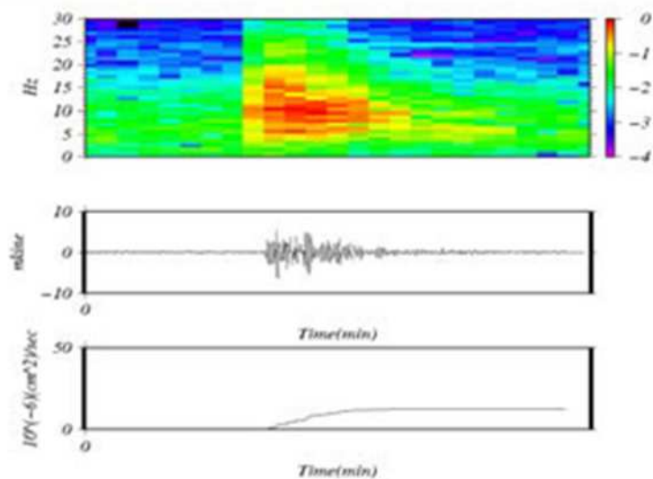
図3 阿蘇山 A型地震の発生状況 2016年10月3日06時~07時(横軸2分)
