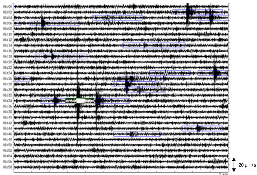
図3 阿蘇山 A型地震の発生状況 2016年10月3日06時~07時(横軸2分)
