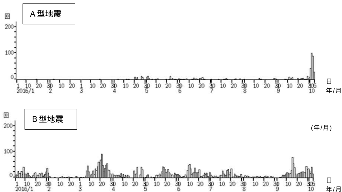
図 1 阿蘇山 日別地震回数（2016 年 1 月 1 日～10 月 3 日）
