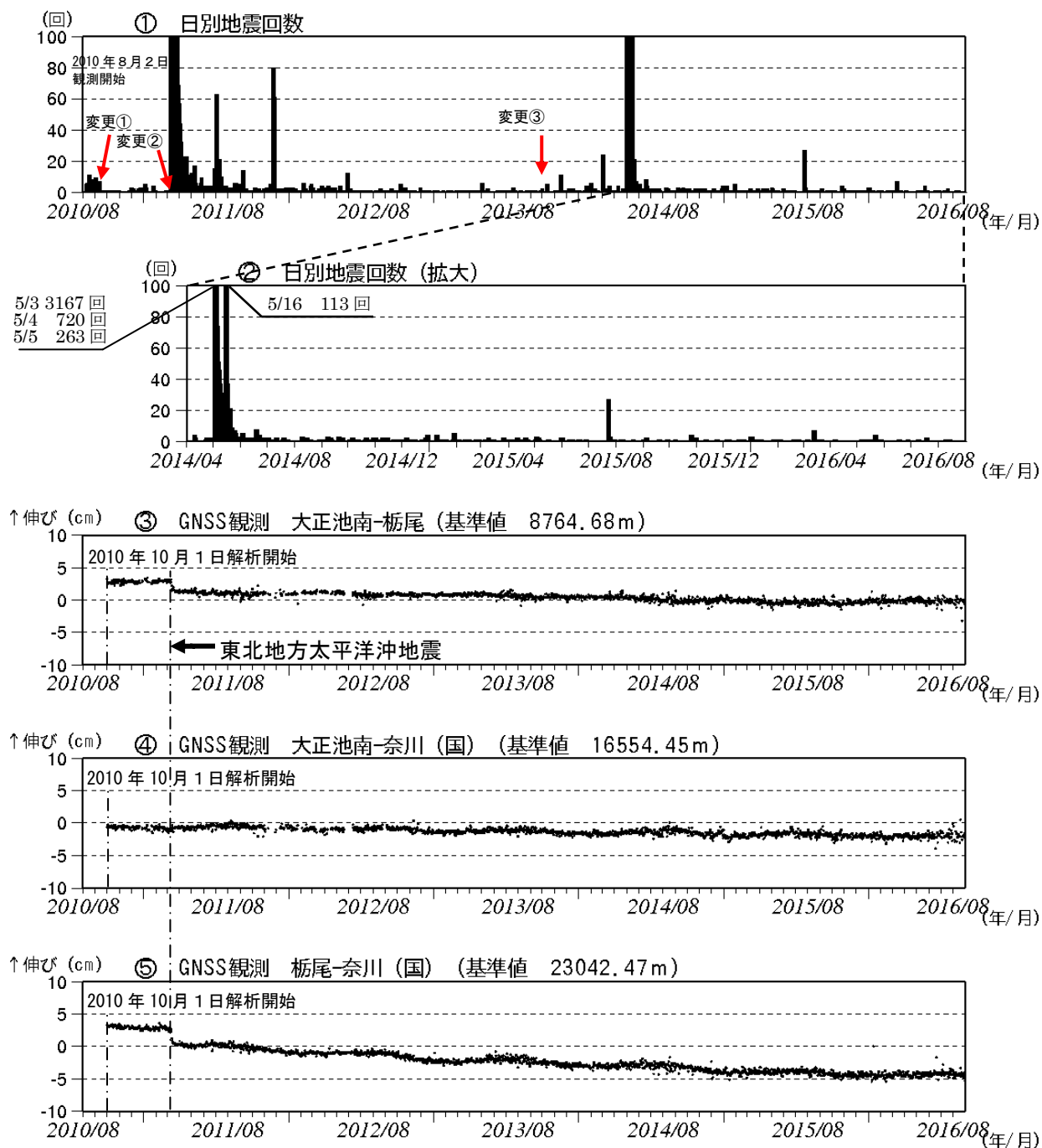
図 8 焼岳 火山活動経過図 (2010 年 8 月 2 日～2016 年 8 月 31 日)
