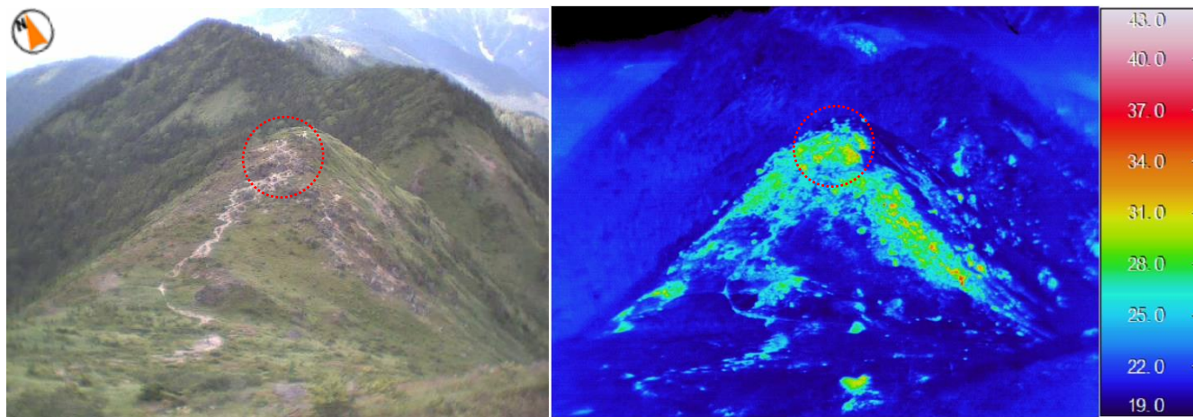
図 6 焼岳 焼岳展望台南斜面周辺の地表面温度分布
