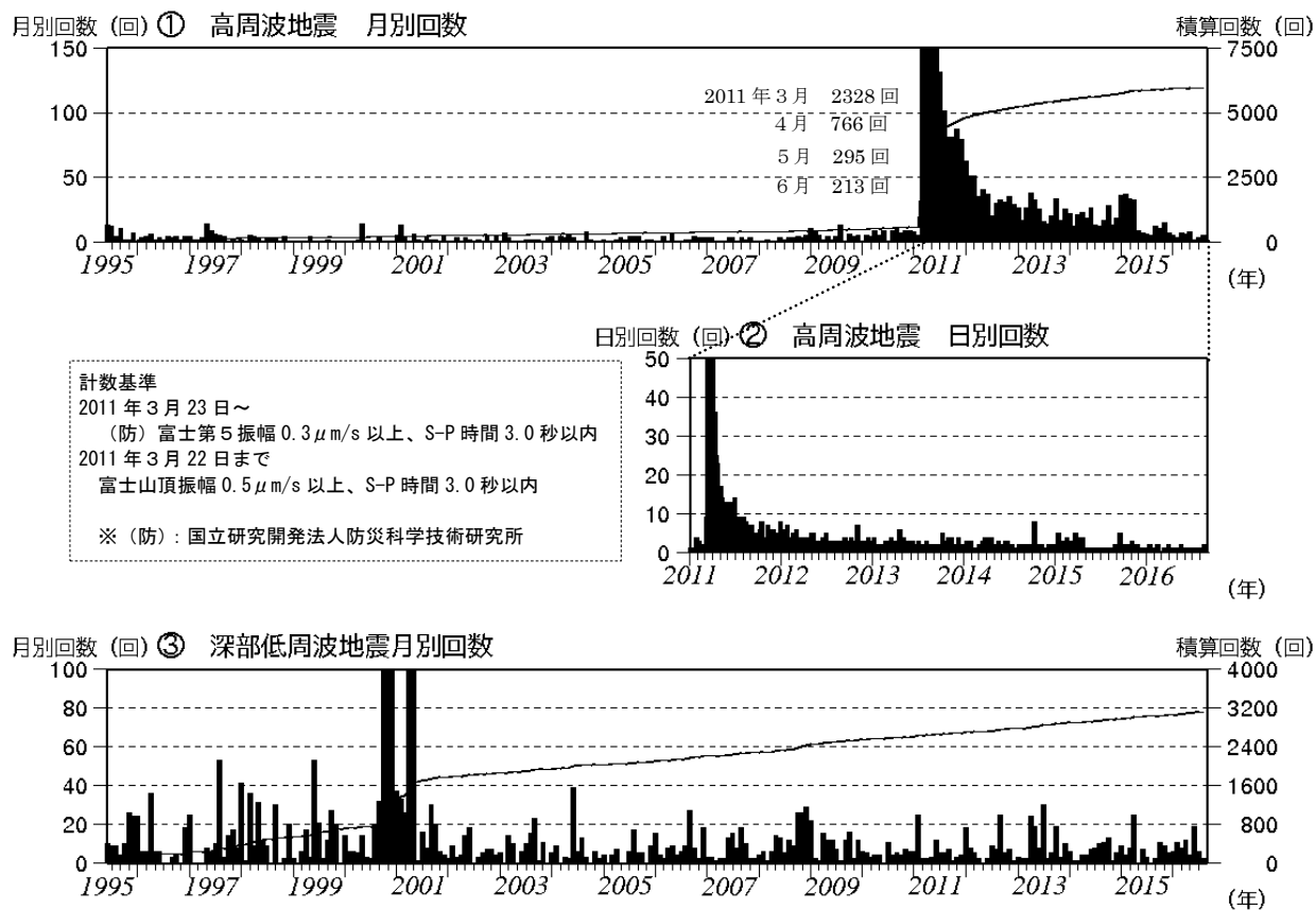
図3 富士山 月別・日別地震回数とその積算回数(1995年6月～2016年8月31日)
