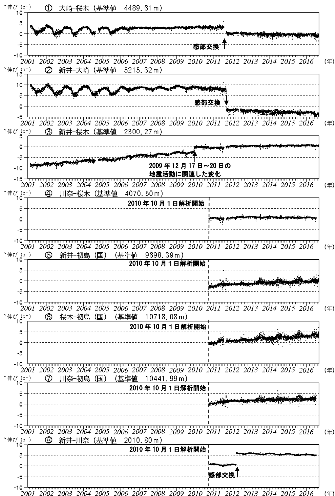
図 6-1 伊豆東部火山群 GNSS 連続観測による基線長変化 (2001 年 1 月～2016 年 8 月 31 日) (観測開始は 2001 年 3 月) (国): 国土地理院
