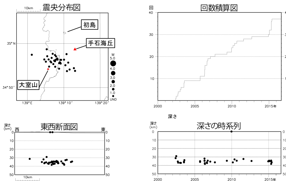
図 3 伊豆東部火山群 一元化震源による深部低周波地震の発生状況 (2000 年 1 月 1 日～2016 年 8 月 31 日) 図 2～3 で表示している震源には、震源決定時の計算誤差の大きなものがある。 この地図の作成には、国土地理院発行の『数値地図 25000 (行政界・海岸線)』を使用した。
