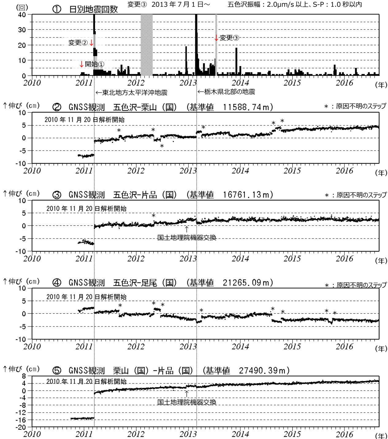
図 4 日光白根山 火山活動経過図 (2010 年 11 月 20 日～2016 年 8 月 31 日)
