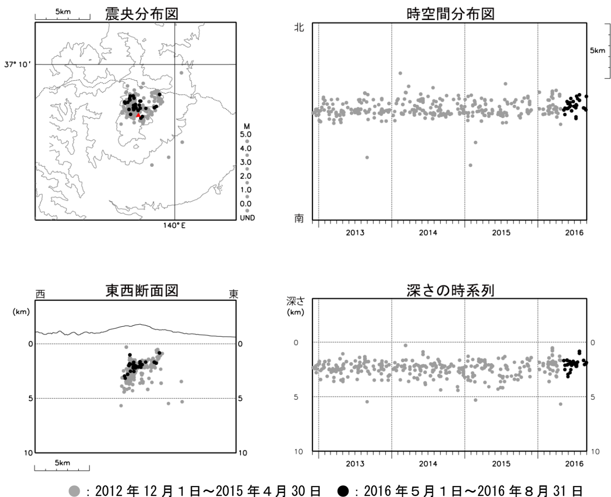
図 4 那須岳 山体周辺の観測点による震源分布図 (2012 年 12 月 1 日～2016 年 8 月 31 日) 半無限均質速度構造 ( V_p = 4.0\text{km/s} , V_p/V_s = 1.73 )
