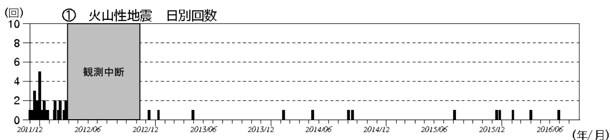
図3 弥陀ヶ原 立山室堂に設置した地震計による地震回数
