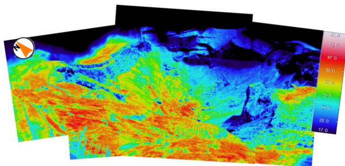
図9 富士山 赤外熱映像装置による山頂火口の地表面温度分布（8月18日）
