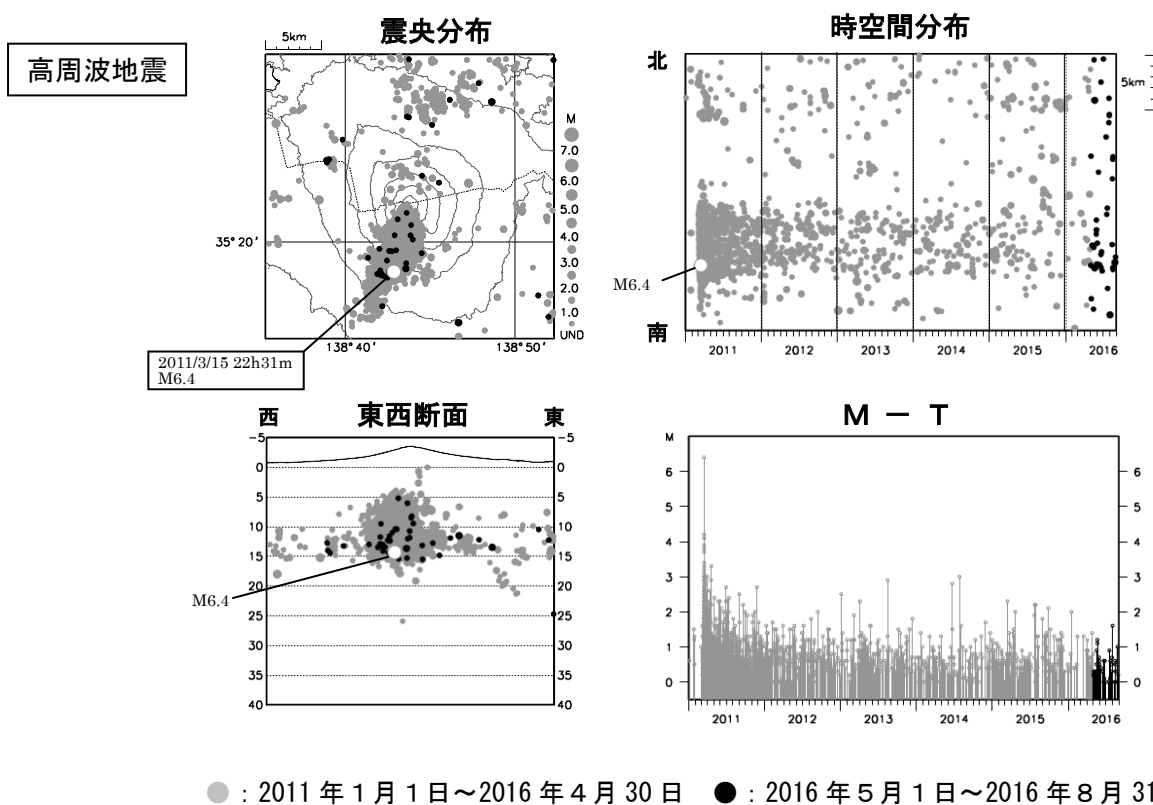
図 4-1 富士山 一元化震源による高周波地震の活動 (1999 年 10 月 1 日～2016 年 8 月 31 日)
