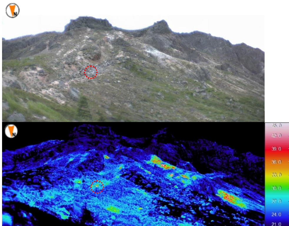
図 5 焼岳 昭和 37 年噴火跡噴気孔、及び焼岳北峰北側斜面周辺の地表面温度分布 昭和 37 年噴火跡噴気孔（図中赤丸）では弱い噴気が認められた。また、北峰北側斜面では至る所に噴気孔が存在し、ごく弱い噴気が認められた。前回（2015 年 7 月 15 日）と比較して、高温領域に特段の変化は認められなかった。
