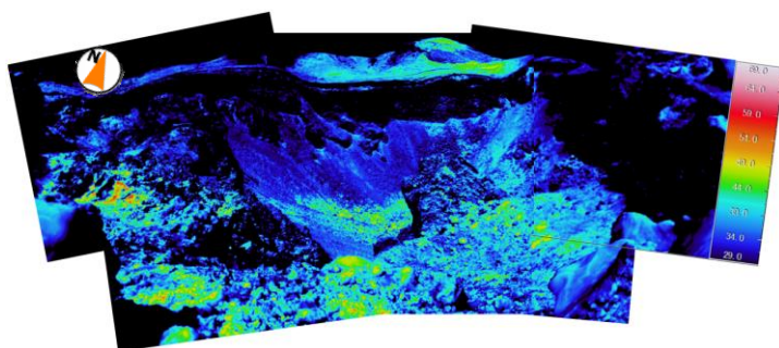
図10 富士山 赤外熱映像装置による山頂火口の地表面温度分布（8月18日）
