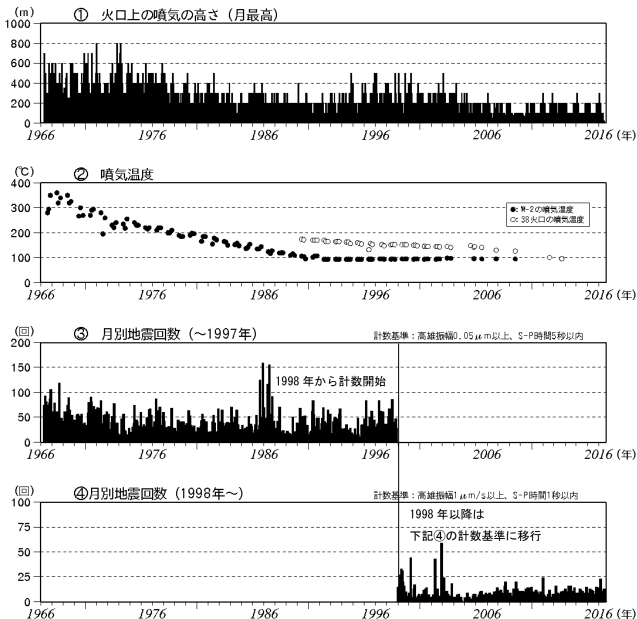
図3 那須岳 火山活動経過図 (1966年1月～2016年8月31日)
