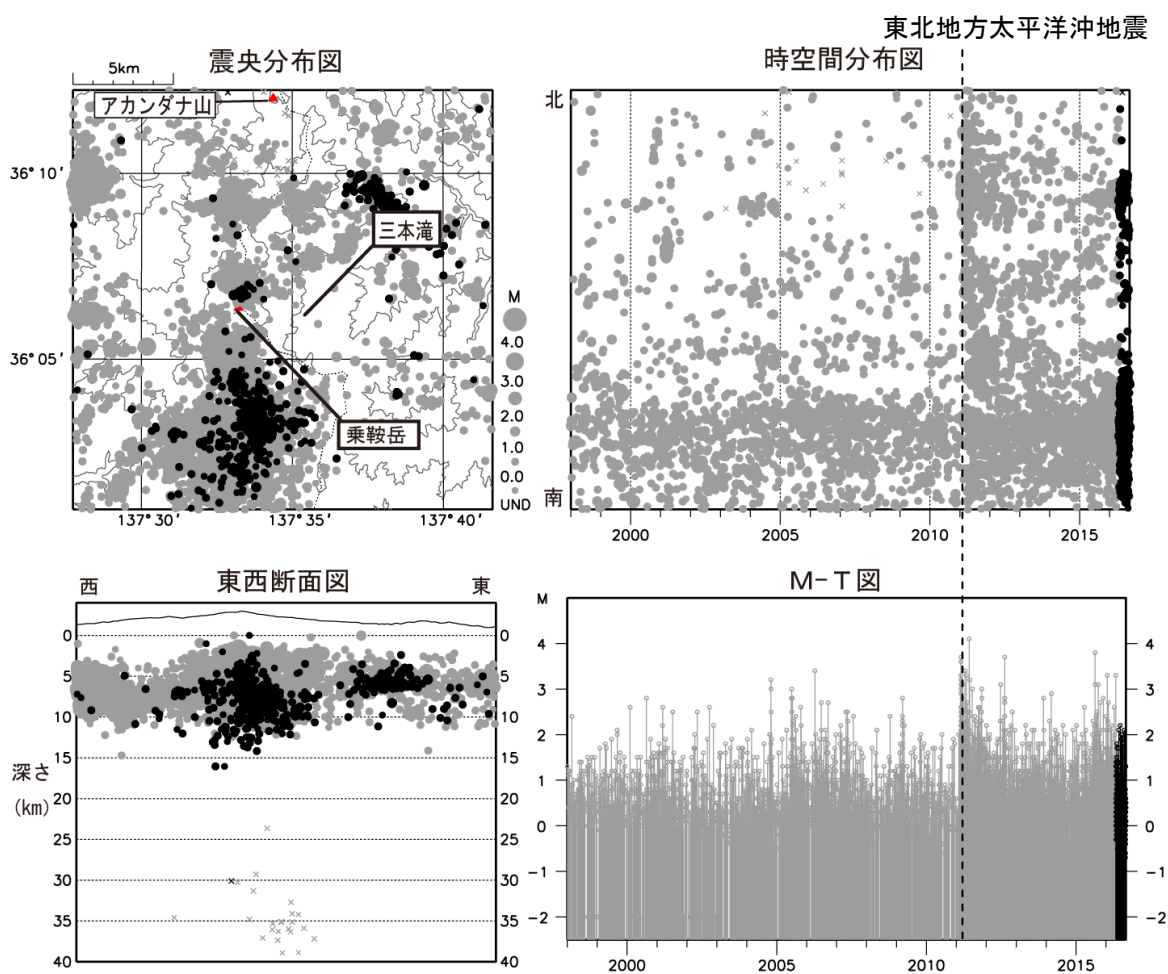
図 5 乗鞍岳 一元化震源による山体・周辺の地震活動(1998年1月1日～2016年8月31日)
