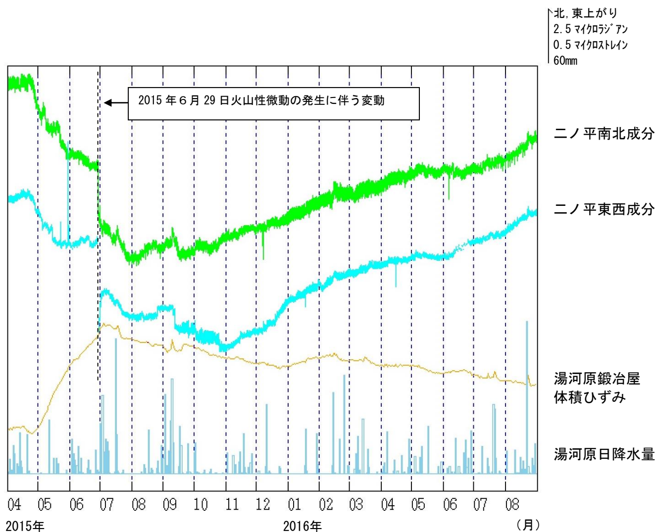
図8 箱根山 ニノ平観測点傾斜データ及び湯河原鍛冶屋観測点における 体積ひずみデータの変化 (2015年4月1日～2016年8月31日)
