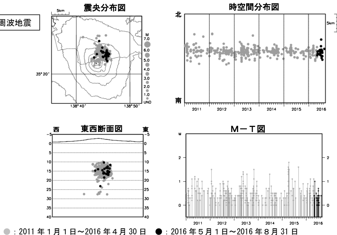
図4-2 富士山 一元化震源による深部低周波地震の活動
