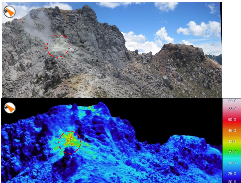
図 3 焼岳 北峰南側噴気孔の状況、及び北峰南斜面周辺の地表面温度分布 噴気孔（図中赤丸）からは高さ 20m ほどの噴気が確認された。前回（2015 年 7 月 15 日）と比較して、高温領域に特段の変化は認められなかった。
