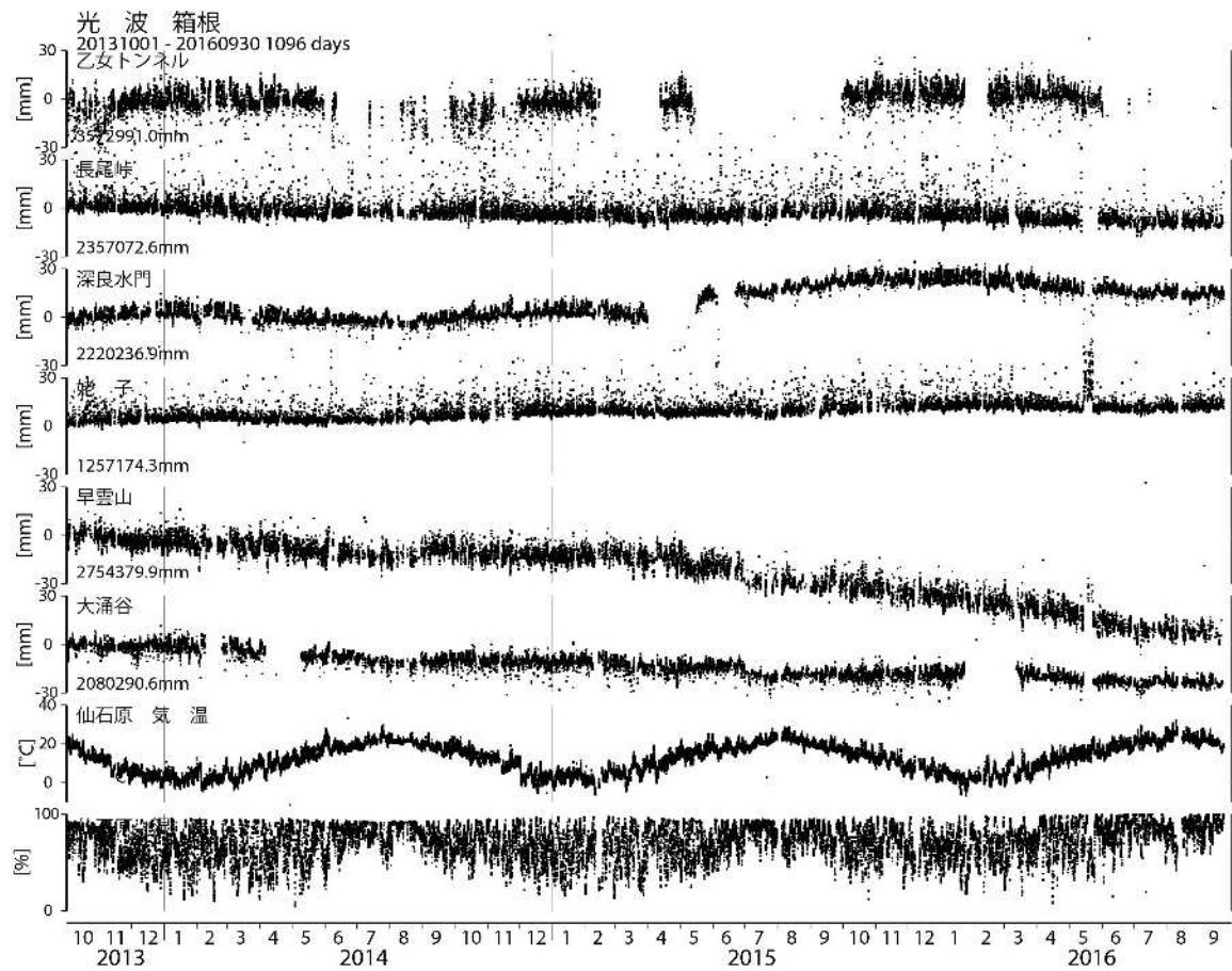
図6 光波測量 (2013年10月1日~2016年9月23日)
