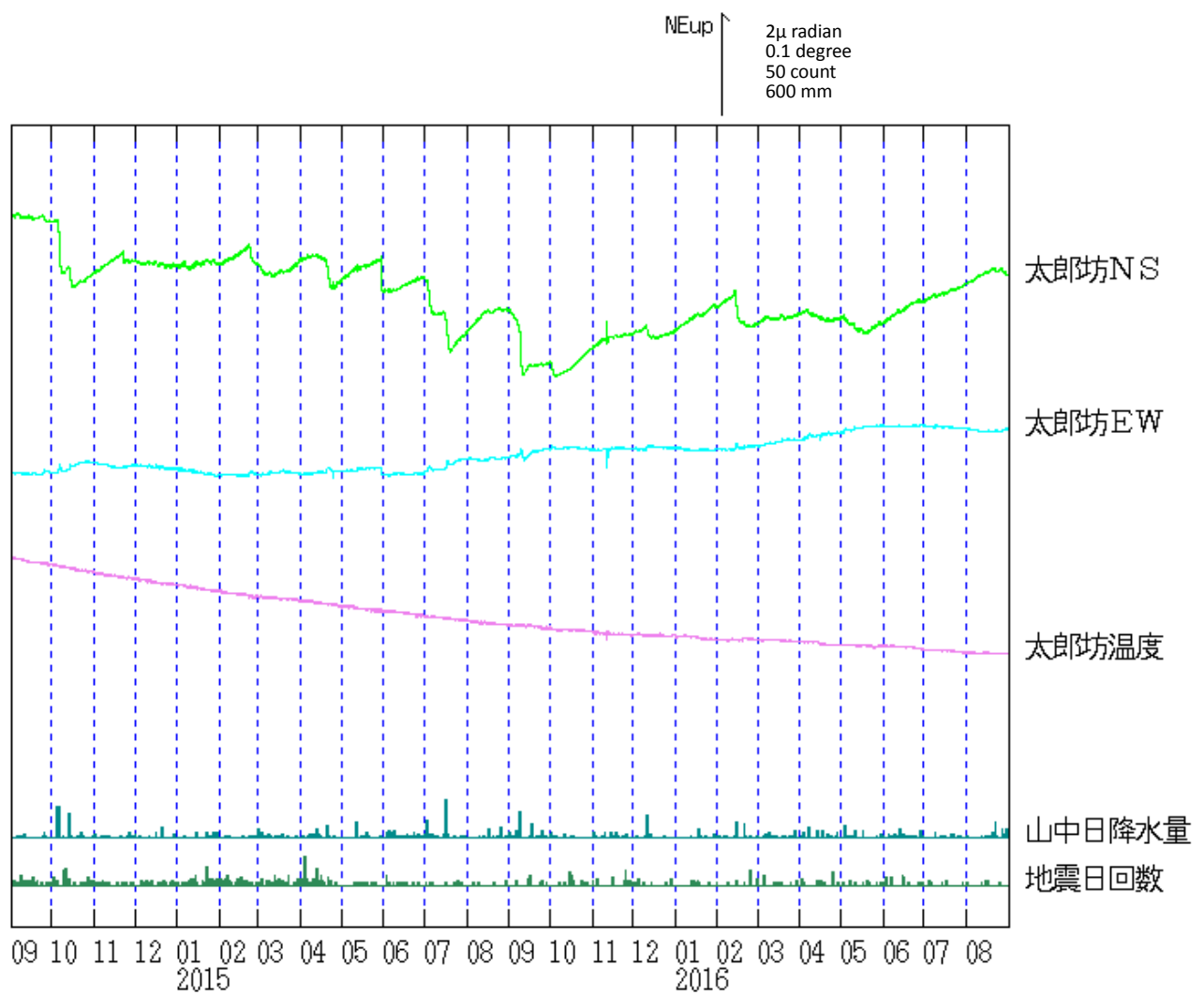
図 7 富士山 太郎坊観測点における傾斜変動
