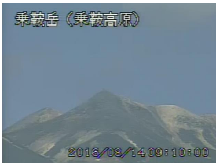
図 2 乗鞍岳 山頂部の状況 (2016 年 8 月 14 日 乗鞍高原遠望カメラによる)
