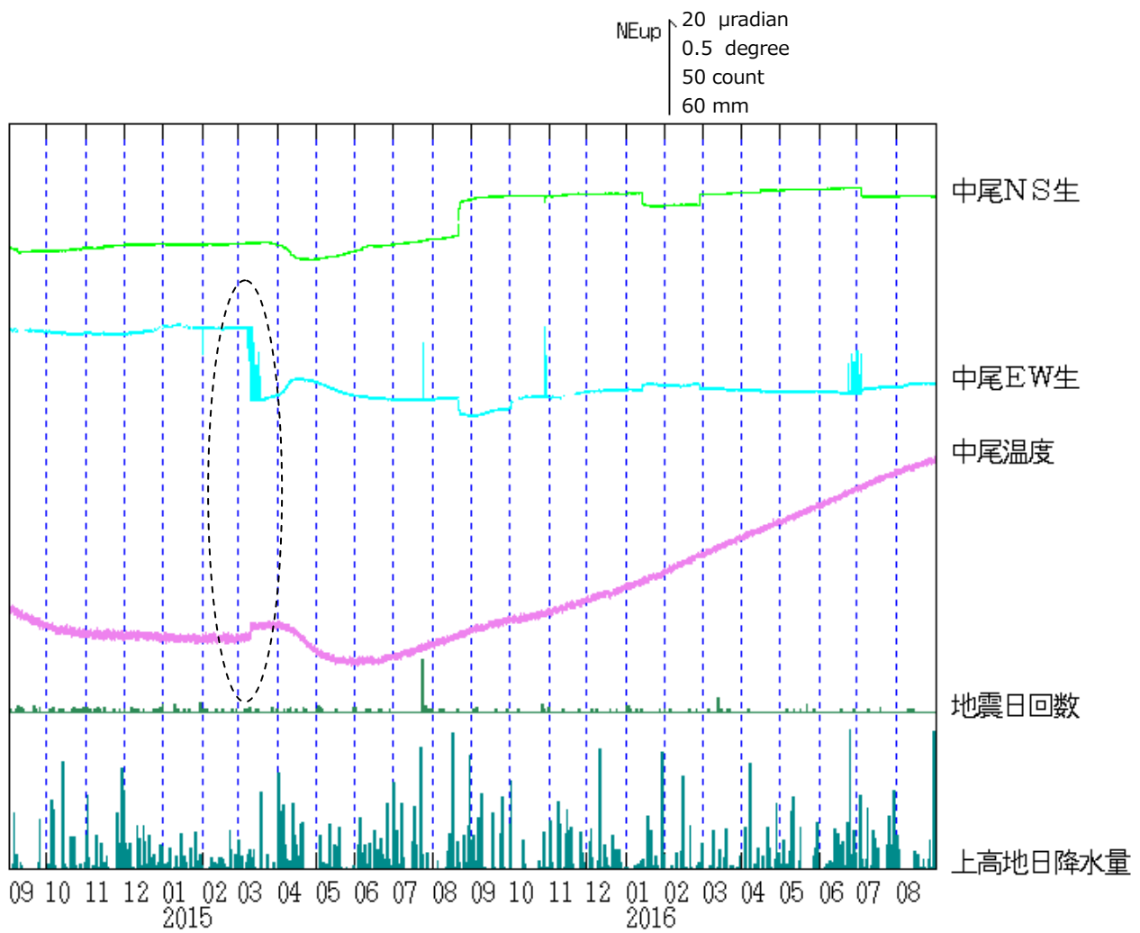
図 12 焼岳 中尾観測点における傾斜変動
