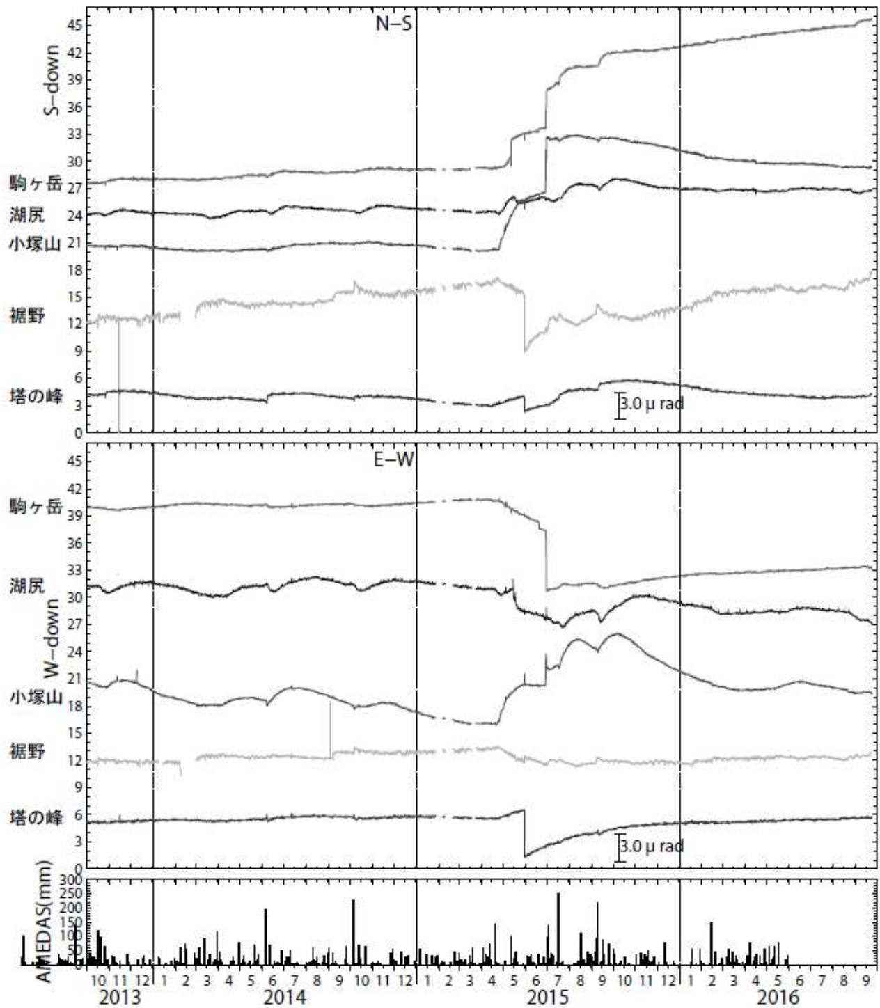
図4 傾斜変動 (2013年10月1日～2016年9月20日)
