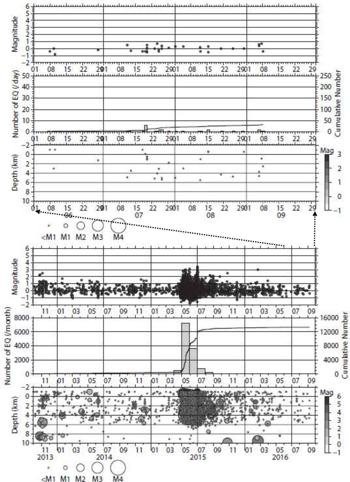
図3 箱根火山周辺の地震活動（2013年10月1日～2016年9月20日）
