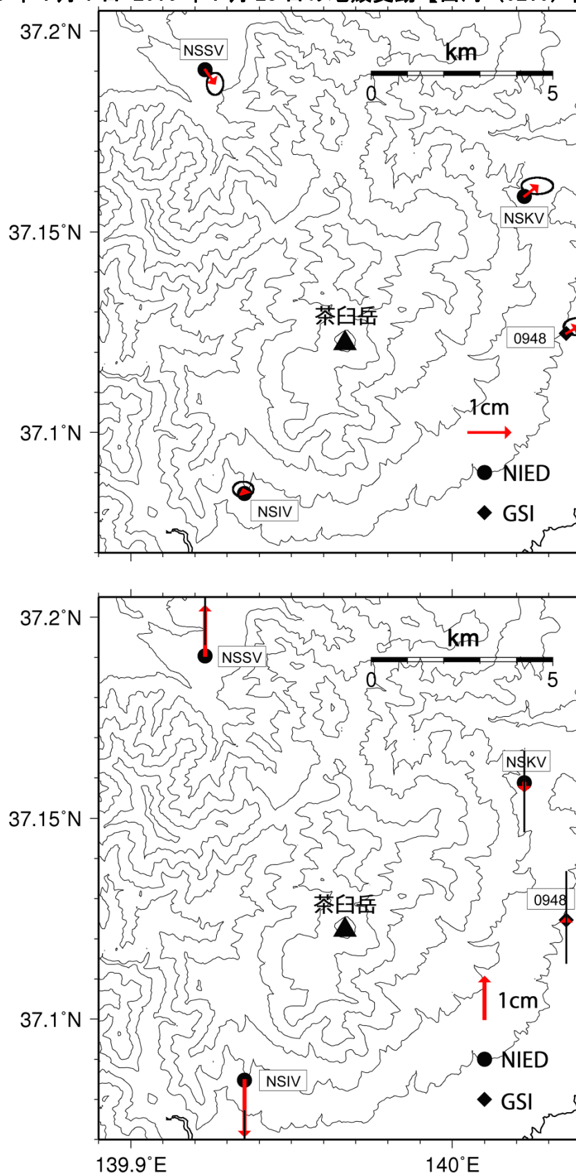
図 1 那須岳周辺 V-net 観測点における GNSS 解析結果.
