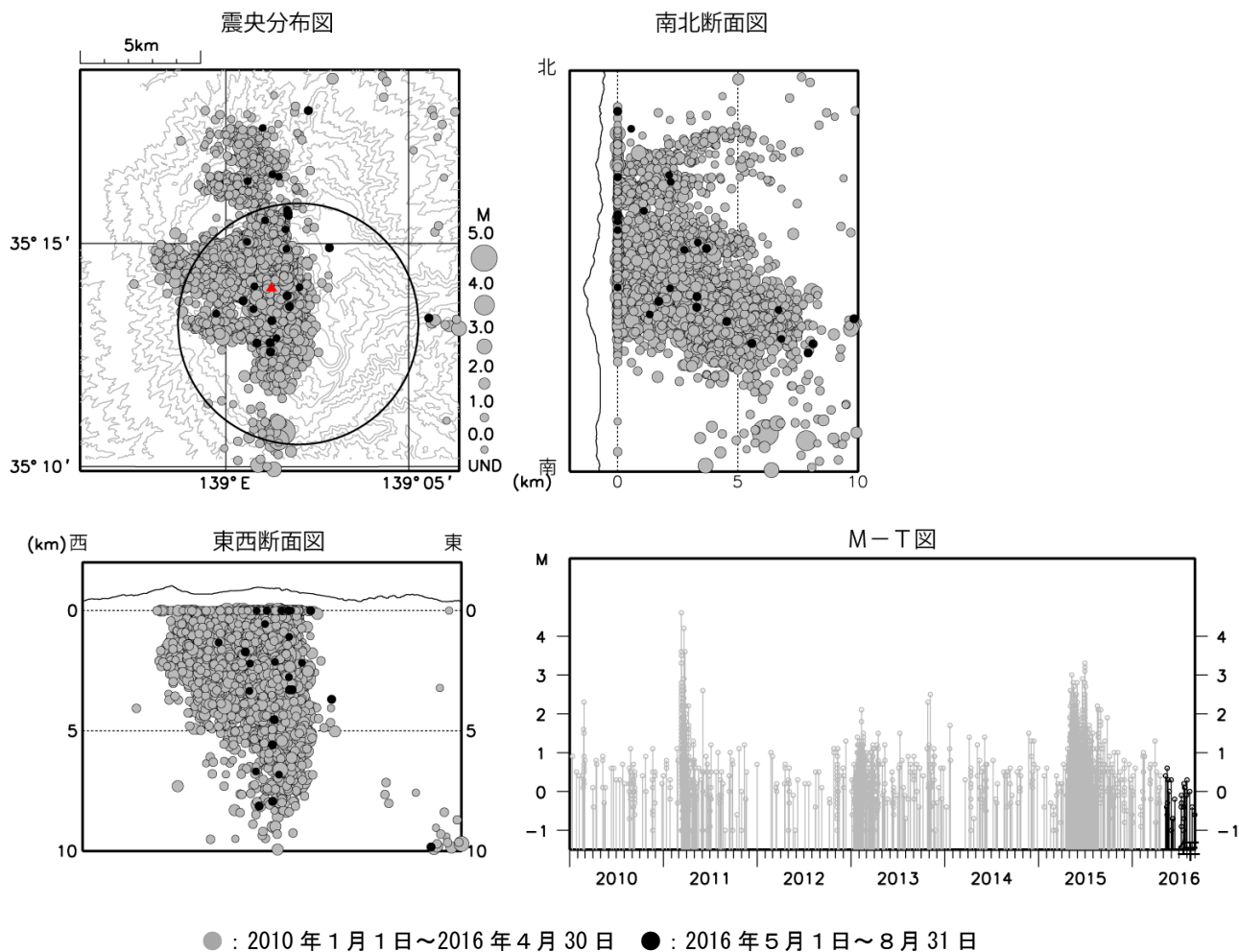
図6 箱根山 一元化による大涌谷周辺の震源分布図(2010 年 1 月 1 日～2016 年 8 月 31 日)
