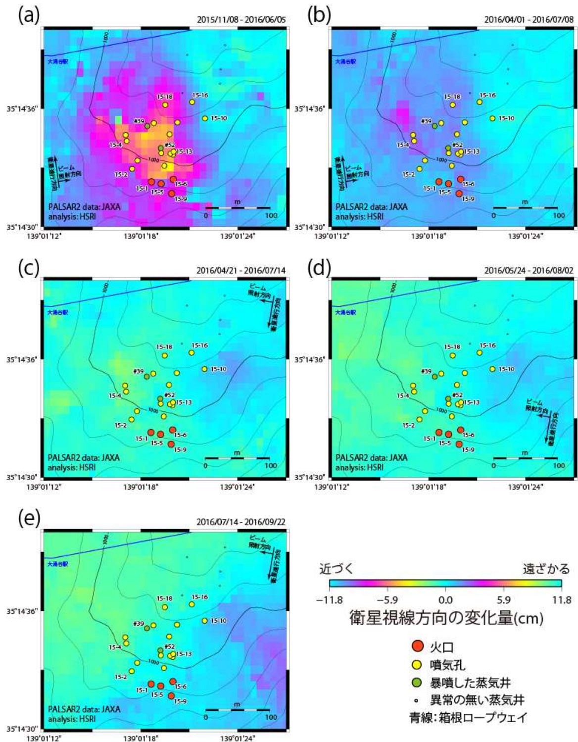
図 1 干渉 SAR 解析による大涌谷の地表面変位
