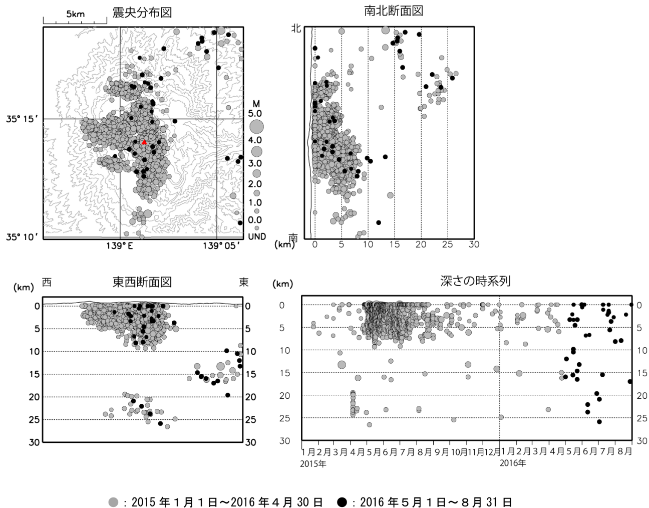
図7 箱根山 一元化による最近の震源分布図（深さ 30km まで） （2015 年 1 月 1 日～2016 年 8 月 31 日）
