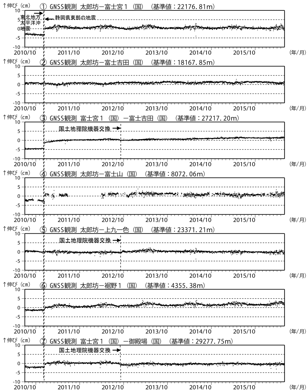
図 5 富士山 GNSS 連続観測による基線長変化 (2010 年 10 月 1 日～2016 年 8 月 31 日)
