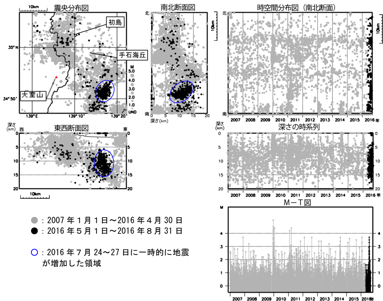
図 2 伊豆東部火山群 一元化震源による地震活動の推移 (2007 年 1 月 1 日～2016 年 8 月 31 日) 今期間、地震活動は概ね低調に経過した。 この地図の作成には、国土地理院発行の『数値地図 25000 (行政界・海岸線)』を使用した。
