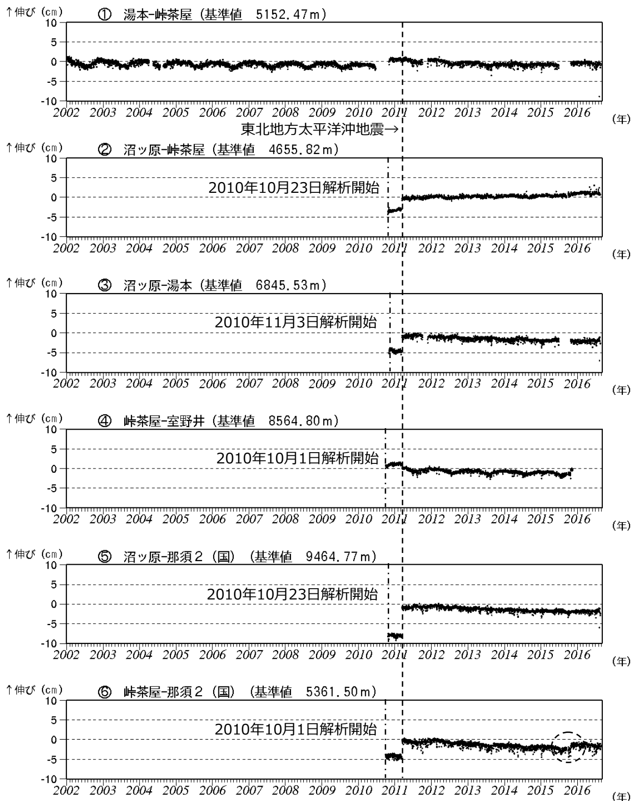
図5 那須岳 GNSS 連続観測による基線長変化 (2002 年 1 月 1 日～2016 年 8 月 31 日)
