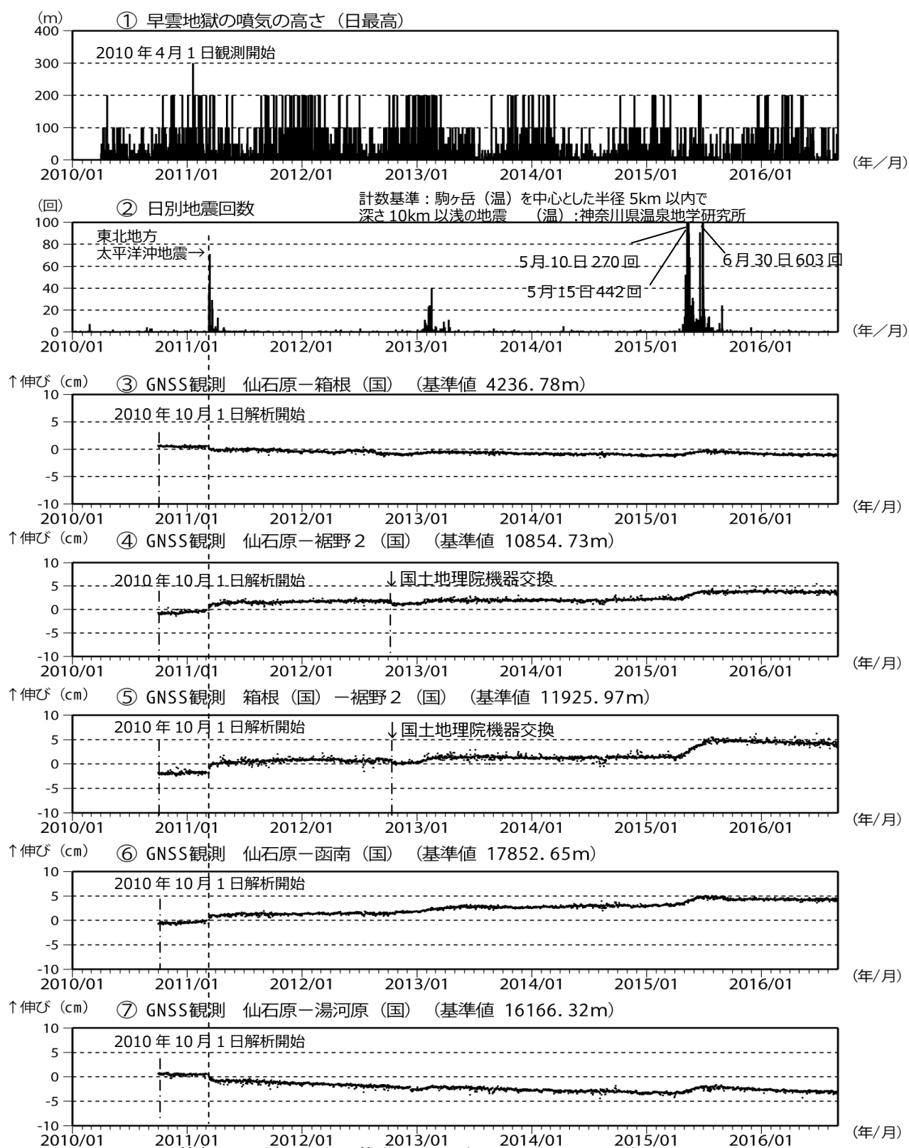
図5 箱根山 火山活動の推移 (2010年1月1日～2016年8月31日)
