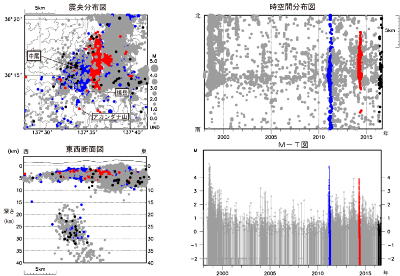
図 10 焼岳 一元化震源による地震活動（1998 年 1 月 1 日～2016 年 8 月 31 日）
