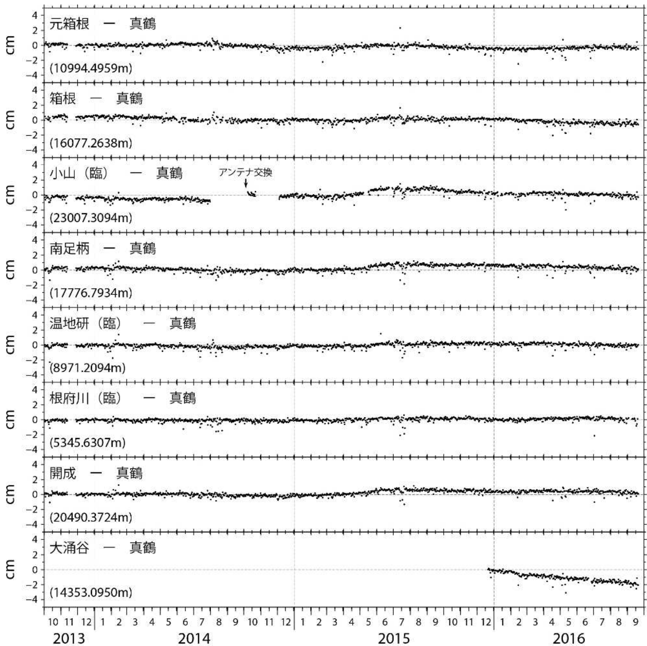
図5 GPS 基線長変動 (2013 年 10 月 1 日～2016 年 9 月 20 日)
