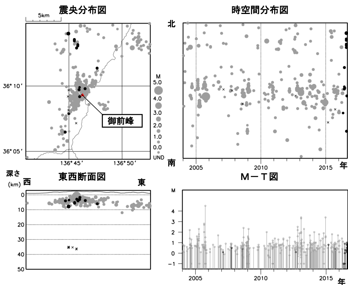
図 4 白山 一元化震源による白山付近の地震活動（2004 年 1 月 1 日～2016 年 8 月 31 日）
