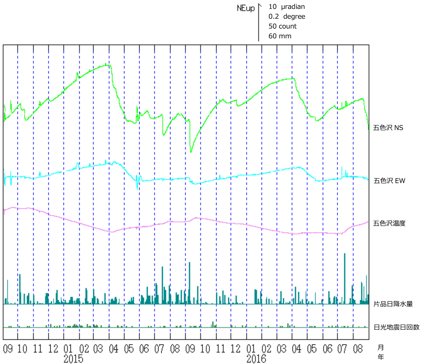
図5 日光白根山 五色沢観測点における傾斜変動 (2014年9月1日～2016年8月31日、時間値、潮汐補正済み) ・火山活動によるとみられる傾斜変動は認められない。
