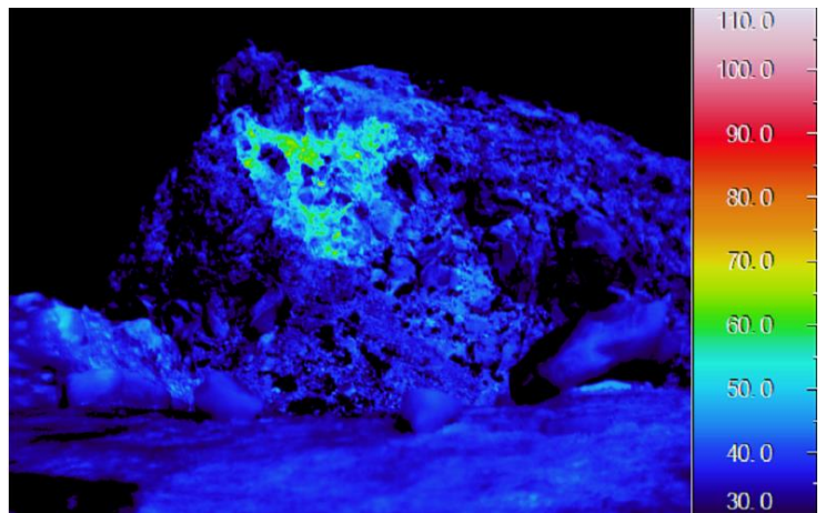
図 4 焼岳 北峰東側噴気孔の状況、及び北峰東斜面周辺の地表面温度分布 噴気孔（図中赤丸）からは高さ 8 m ほどの噴気が確認された。前回（2015 年 7 月 15 日）と比較して、高温領域に特段の変化は認められなかった。
