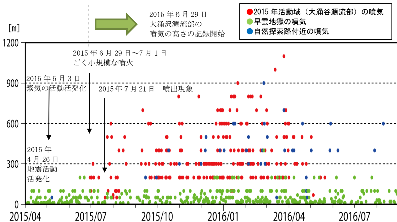
図4 箱根山 遠望カメラによる噴気の高さ（火口上）の推移 （2015年4月1日～2016年8月31日）
