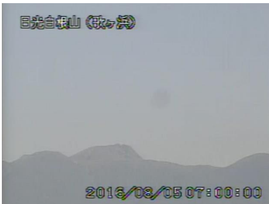
図 1 日光白根山 山頂部の状況 (2016 年 8 月 5 日 歌ヶ浜遠望カメラによる)
