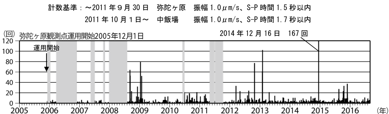
図 3 白山 日別地震回数（2005 年 12 月～2016 年 8 月 31 日）（図の灰色部分は機器障害による欠測期間）
