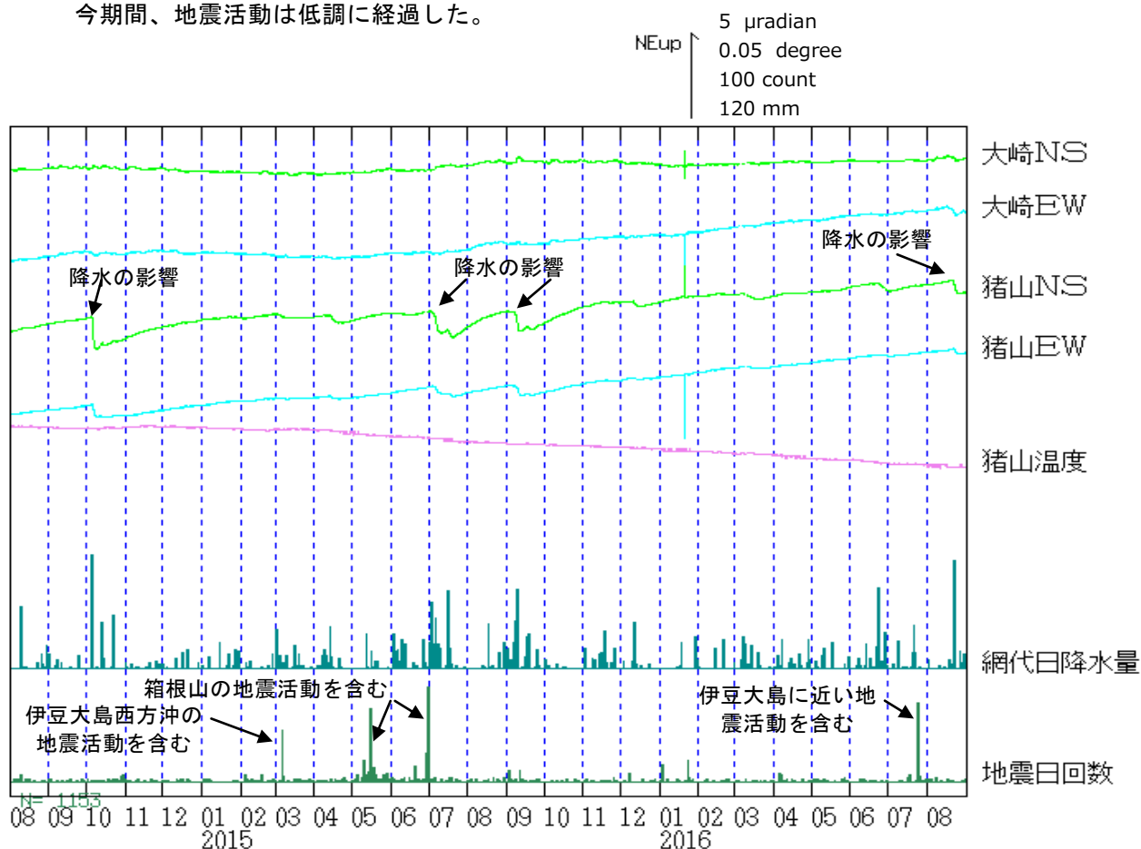
図5 伊豆東部火山群 大崎及び猪山観測点における傾斜変動 （2014年8月1日～2016年8月31日、時間値、いずれも潮汐補正済み） 今期間、火山活動によると見られる傾斜変動は認められなかった。
