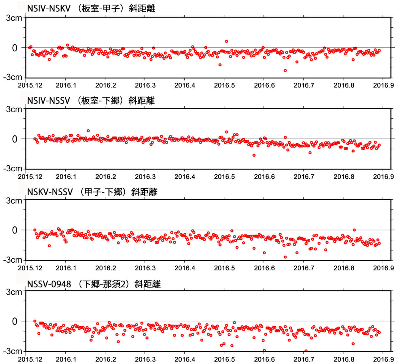
図 2 防災科研観測点 3 点 (板室, 甲子, 下郷) 間及び, 下郷-GEONET 那須 2 間の基線長変化.
