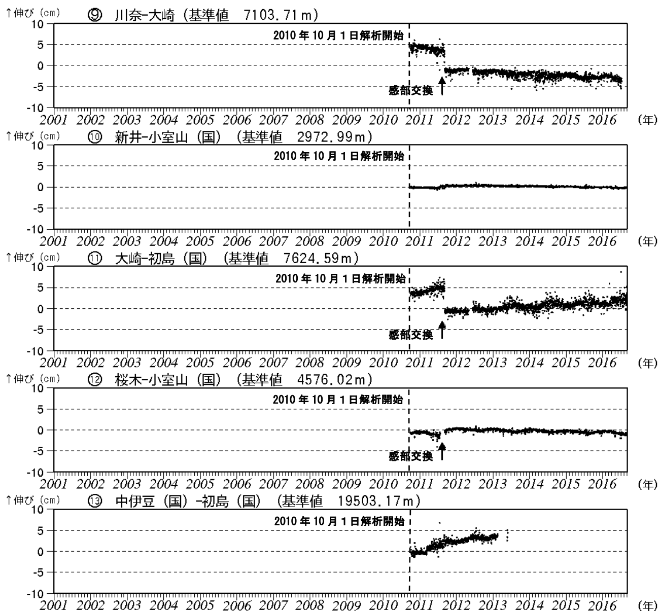
図 6-2 伊豆東部火山群 GNSS 連続観測による基線長変化 (2001 年 1 月～2016 年 8 月 31 日)
