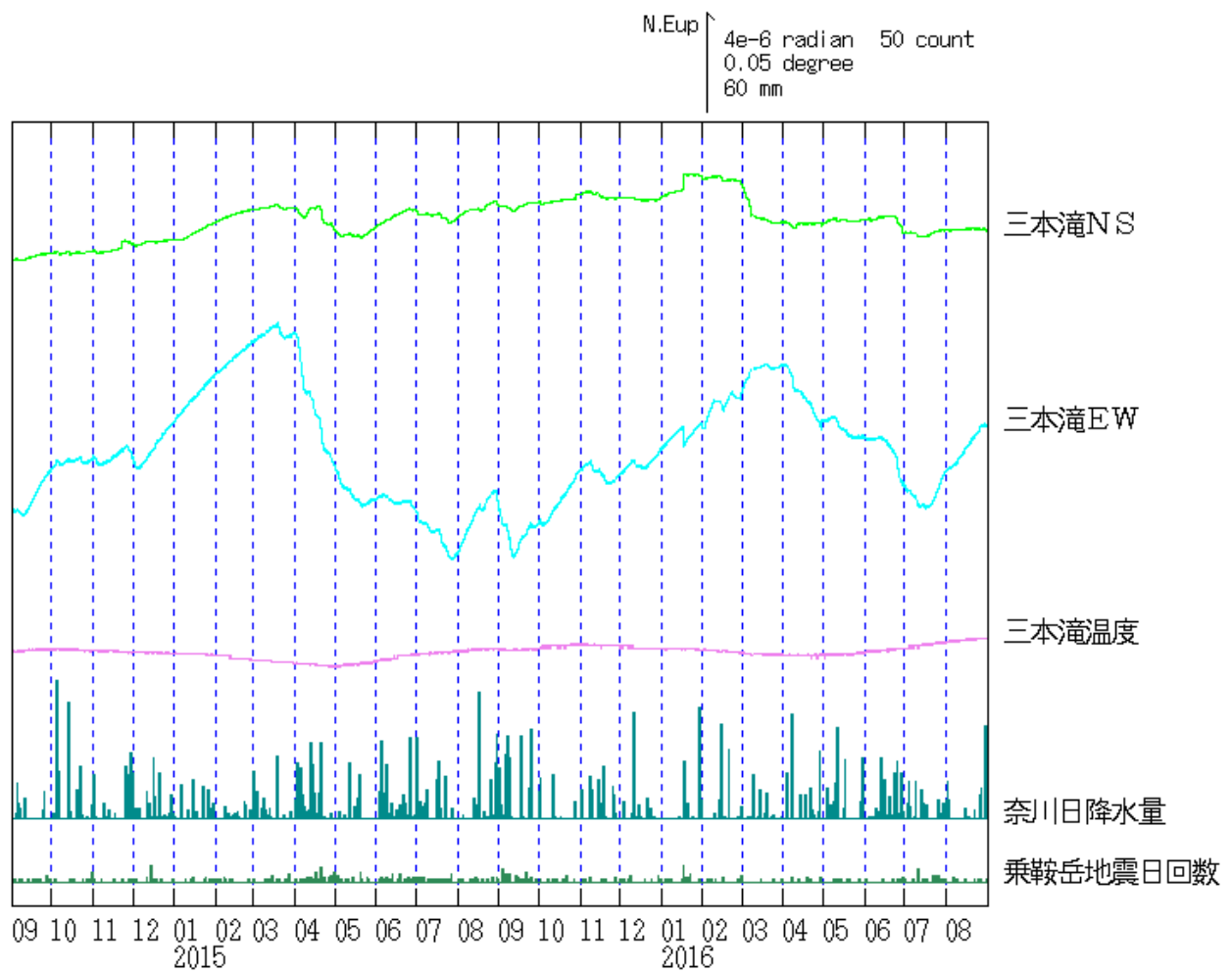
図6 乗鞍岳 三本滝観測点における傾斜変動 (2014年9月1日～2016年8月31日、時間値、潮汐補正済み) ・火山活動によるとみられる傾斜変動は認められない。
