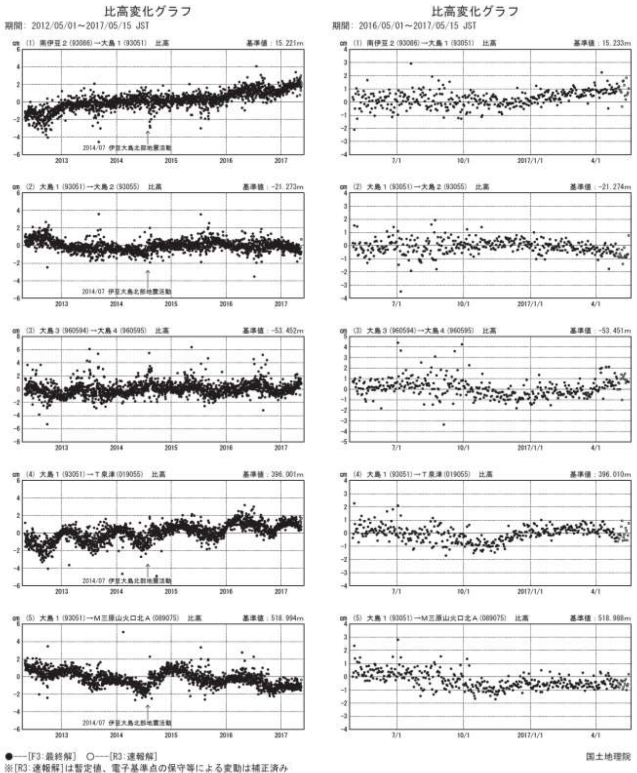
第 2-2 図 伊豆大島の GNSS 連続観測結果
