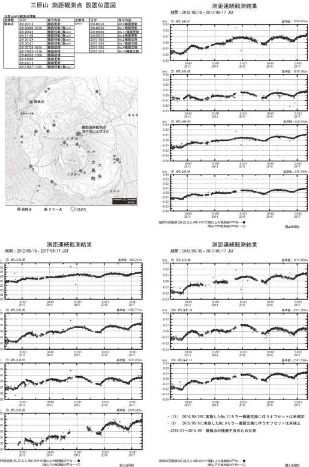
第4図 伊豆大島の光波測距観測結果 (左上段：観測点配置図、右上段及び下段：連続観測結果 2012年5月～2017年5月)
