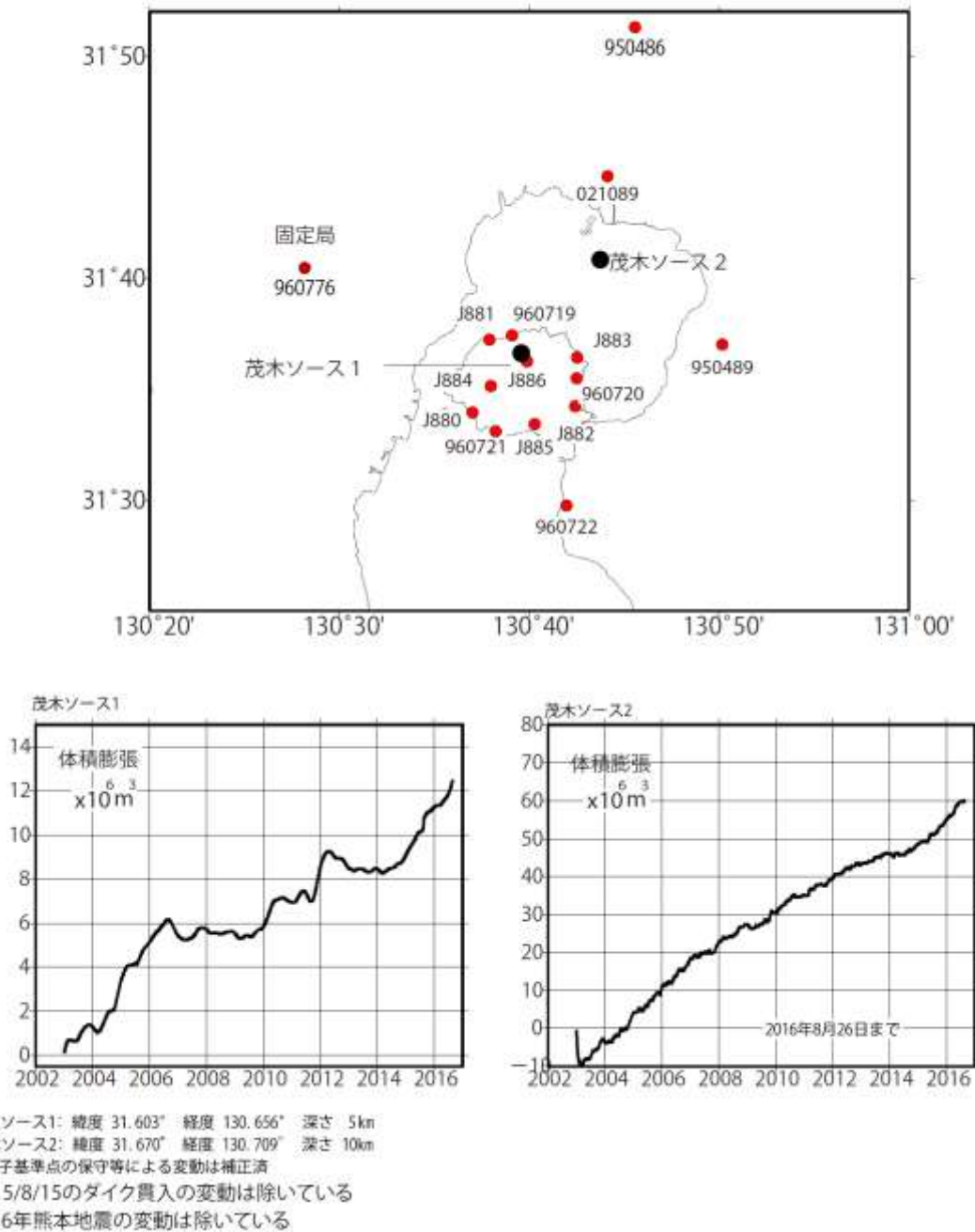
第5図 時間依存インバージョンの手法による桜島の変動源の体積変化推定・茂木ソース2つを仮定（上段：推定に用いた観測点（赤点）の配置と茂木ソースの位置（黒丸）、下段左、推定された茂木ソース体積の時間変化・桜島直下、下段右：推定された茂木ソース体積の時間変化・始良カルデラ深部）
