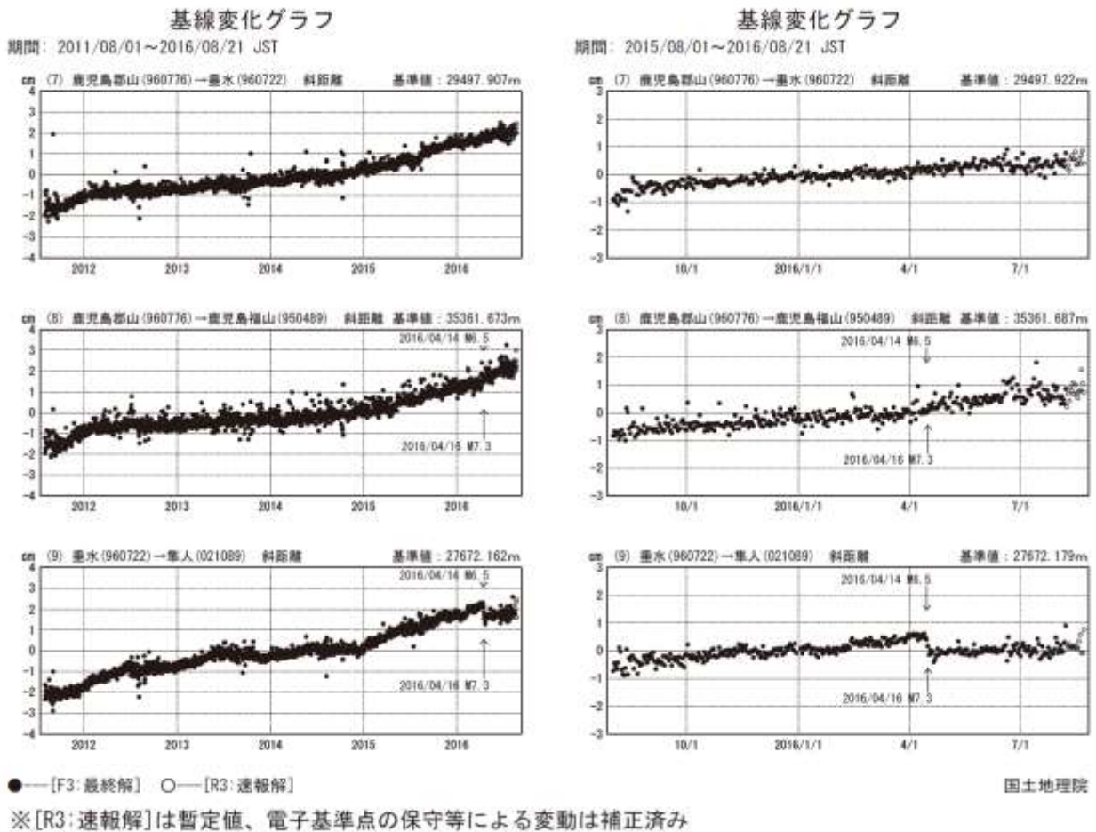
第 2-2 図 桜島周辺の GNSS 連続観測による基線変化グラフ (左列: 2011 年 8 月~2016 年 8 月、右列: 2015 年 8 月~2016 年 8 月)
