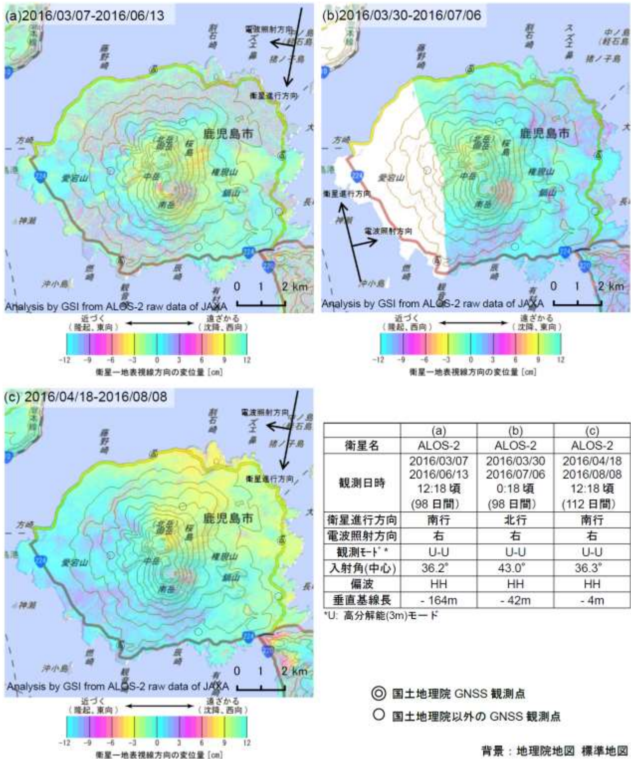
第8図 「だいち2号」PALSAR-2による桜島周辺地域の解析結果
