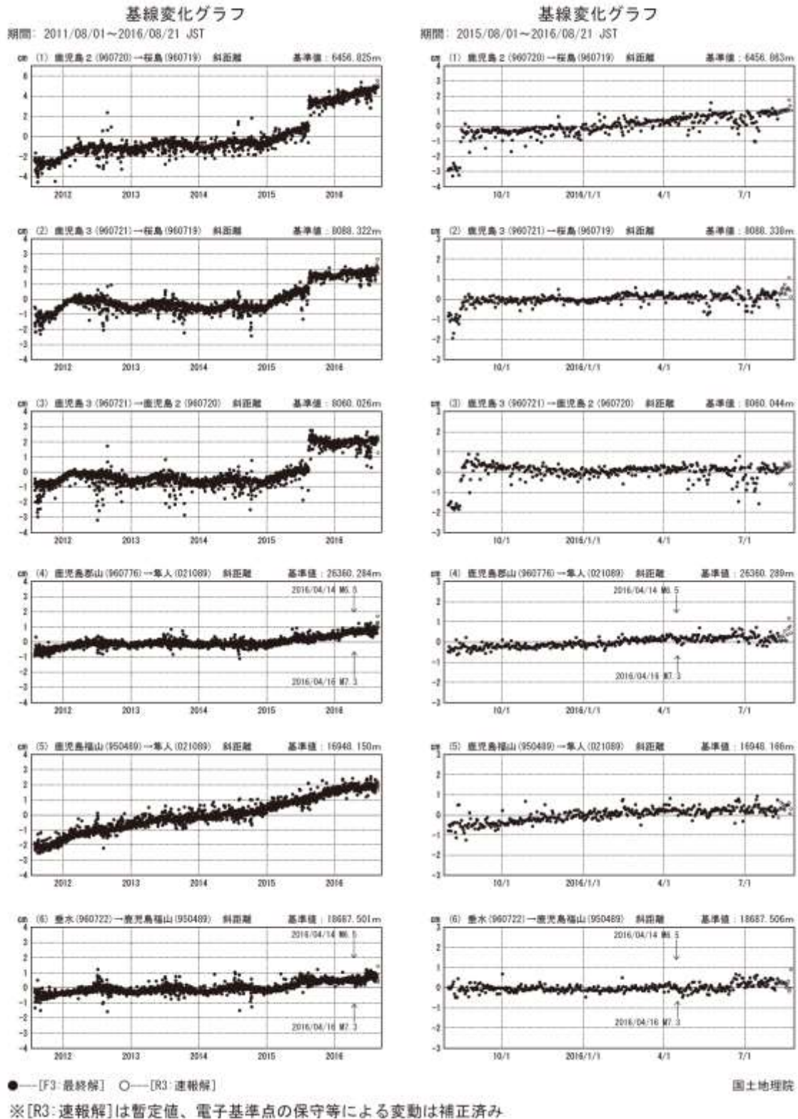
第 2-1 図 桜島周辺の GNSS 連続観測による基線変化グラフ (左列: 2011 年 8 月~2016 年 8 月、右列: 2015 年 8 月~2016 年 8 月)
