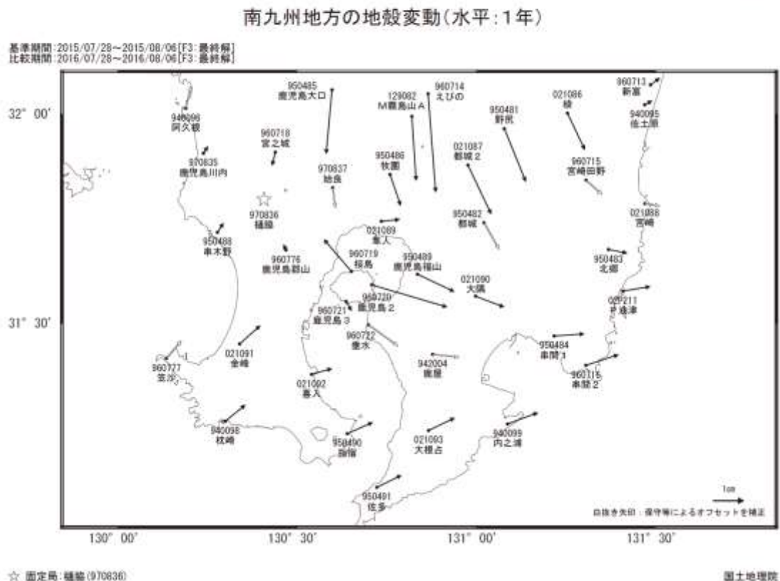
第3図 桜島周辺におけるGNSS観測点の水平変動ベクトル図(上段:2016年4月~2016年7月、下段:2015年7月~2016年7月)
