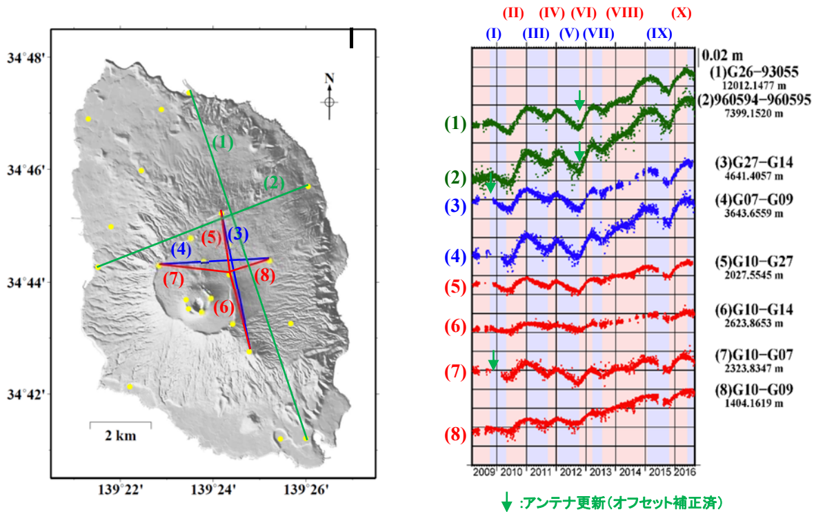
第 4 図 2009 年 3 月 1 日から 2016 年 9 月 3 日までの GNSS 基線長変 Fig. 4 Temporal changes of GNSS baseline lengths during a period from March 1, 2009 to September 3, 2016.
