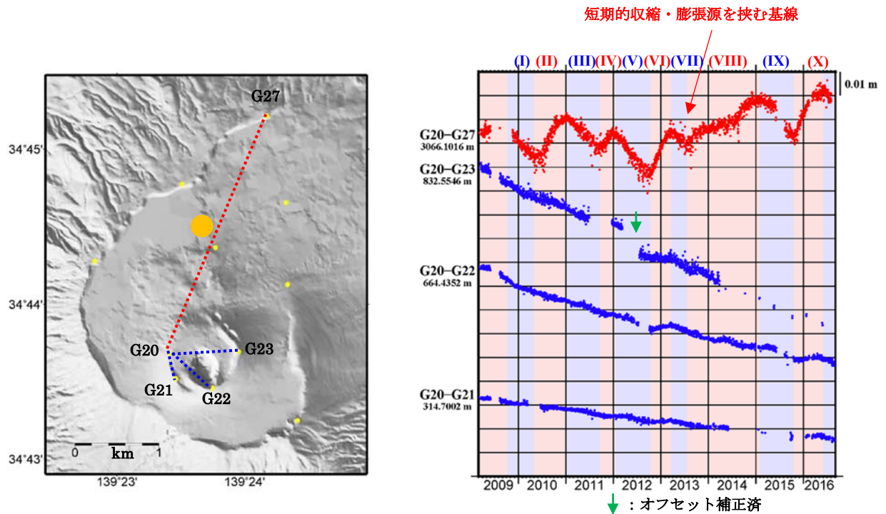
第12図 (左) 基線と短期的収縮・膨張源との位置関係。(●: 短期的収縮・膨張源)。(右) 三原山火口西(G20)を基準とした基線長変化(2009年3月1日から2016年9月3日まで)。
