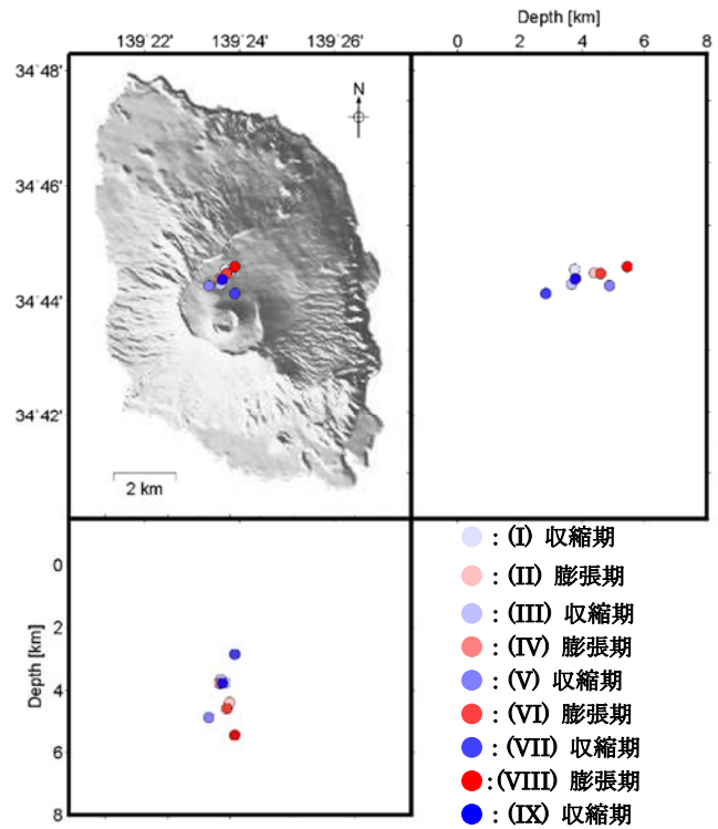
第 8 図 期間(I)～(IX)について推定された収縮源・膨張源の位置。
