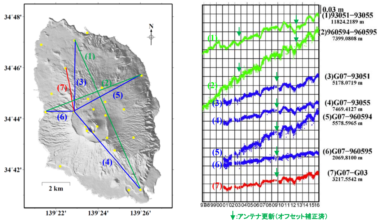
第2図 1997年10月1日から2016年9月3日までのGNSS基線長変化。
