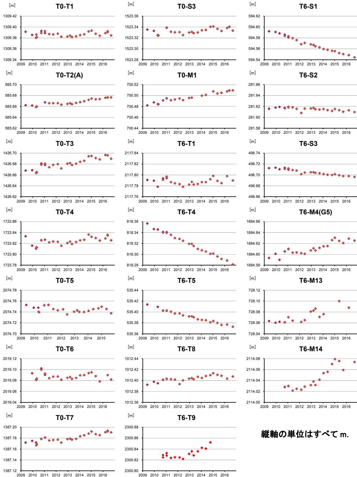
第 15 図 伊豆大島カルデラ内の EDM 繰返し観測網 (第 13 図 B) による斜距離変化 (2009 年 3 月～2016 年 9 月)。
