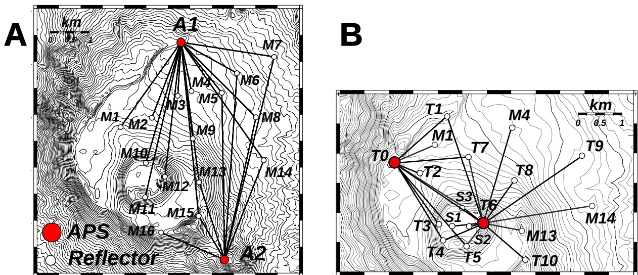
第13図 伊豆大島カルデラ内の光波測距観測点配置図と測線。
