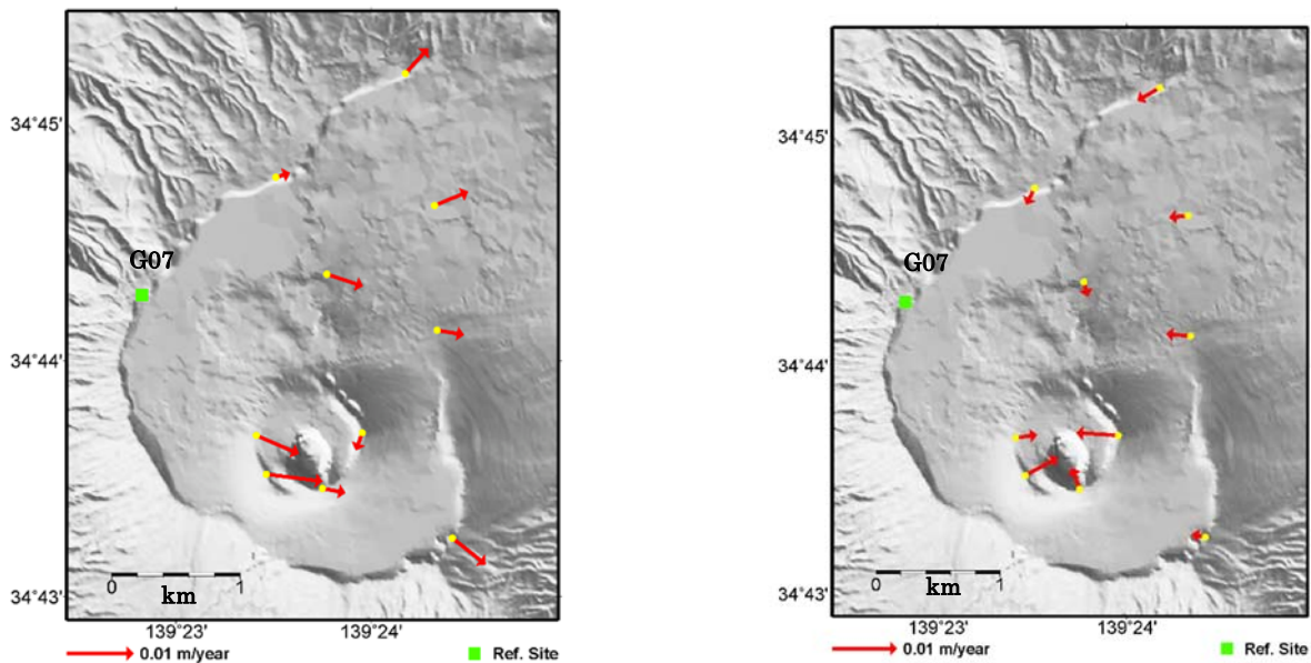
第10図 北西カルデラ縁 (G07) を基準とした三原山観測点の相対変位 (2013年9月4日から2016年9月3日まで)。(右) 推定した変動源 (図12 (左) 参照) とその体積変化量 (図9参照) から求められる各点の水平変位を補正したもの。火口付近の収縮が明瞭になっている。
