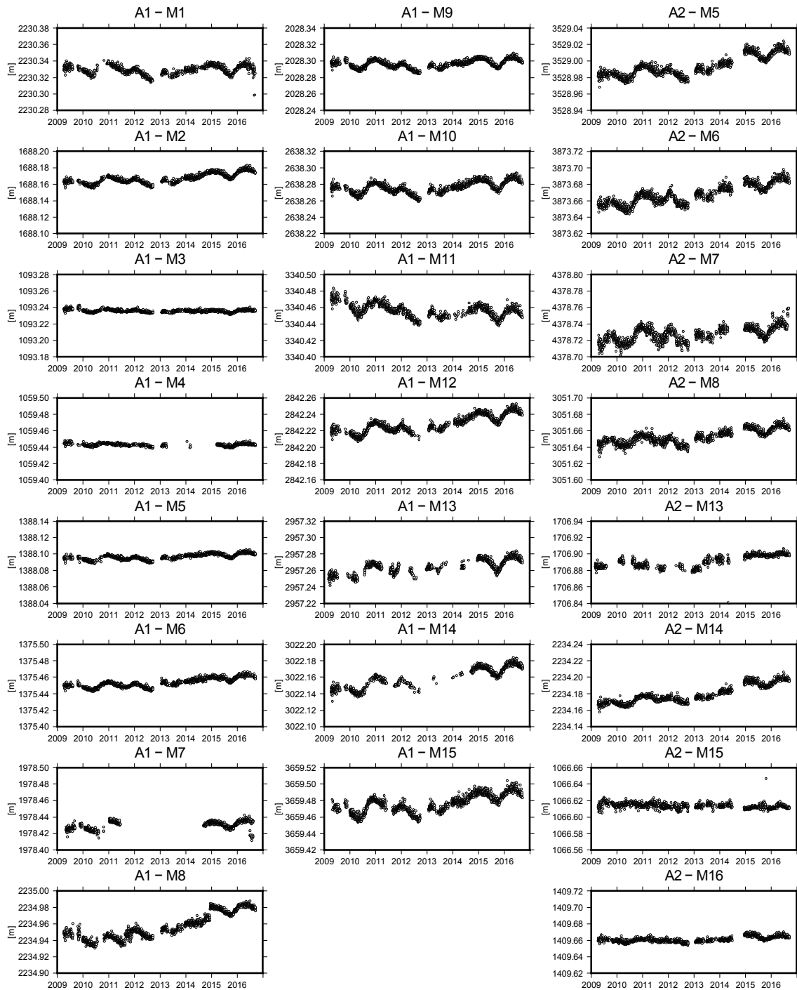
第 14 図 伊豆大島カルデラ内の EDM 連続観測網 (第 13 図 A) による斜距離変化 (2009 年 4 月 1 日 ~2016 年 9 月 23 日)。
