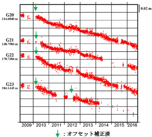
第 11 図 北西カルデラ縁 (G07) を基準とした三原山観測点の上下の相対変位 (2009 年 3 月 1 日から 2016 年 9 月 3 日まで)。
