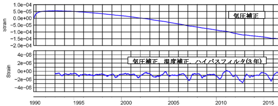
第 5 図 1990 年 10 月から 2016 年 9 月までの体積ひずみ変化. (上) 気圧補正のみ. (下) 短周期成分.
