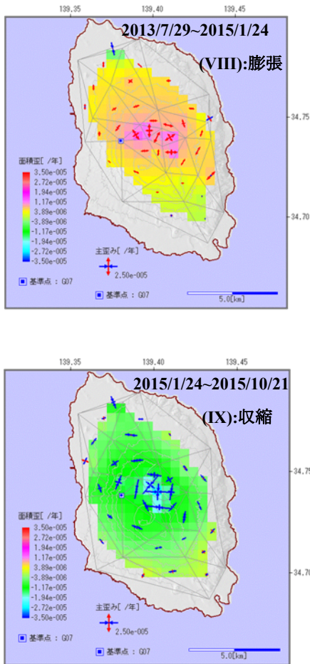
第 7 図 GNSS データから作成した短期的収縮，膨張の主歪・面積ひずみ分布（年率）の例。
