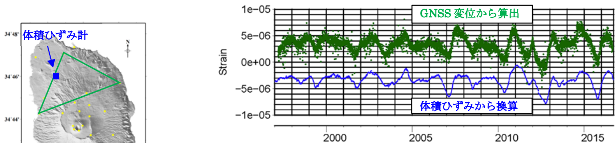
第 6 図 1997 年 1 月から 2016 年 9 月までの面積ひずみ短周期成分の経年変化. 青: 体積ひずみから換算した面積ひずみ. 緑: 左図三角形で示された 3 観測点の GNSS データから算出した面積ひずみ.
