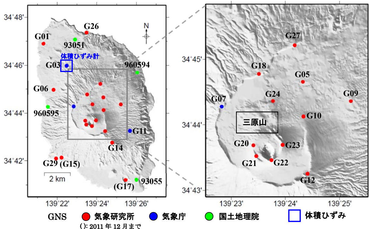
第 1 図 GNSS および体積ひずみ連続観測点位置。
