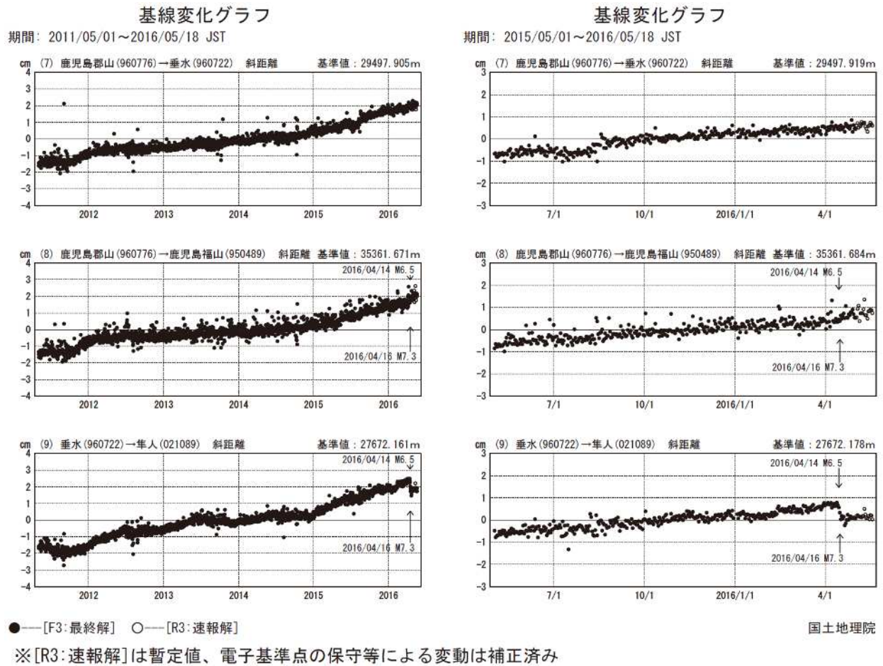
第2図(b) 桜島周辺のGNSS連続観測による基線変化グラフ(左列:2011年5月~2016年5月、右列:2015年5月~2016年5月)
