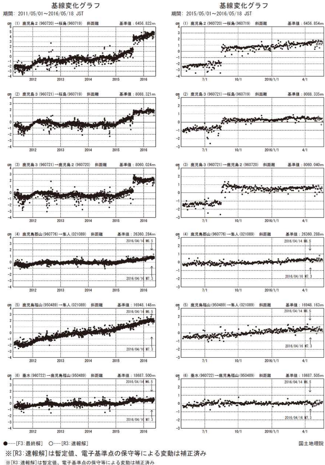
第2図(a) 桜島周辺のGNSS連続観測による基線変化グラフ(左列:2011年5月~2016年5月、右列:2015年5月~2016年5月)
