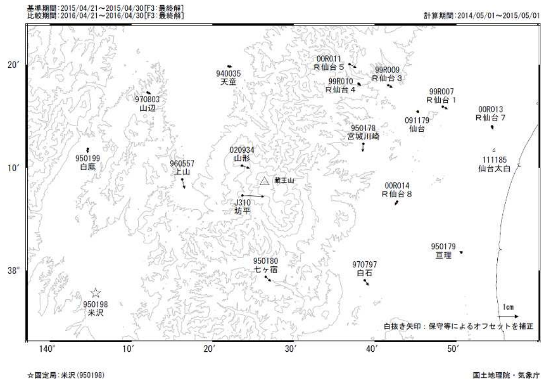
第2図 蔵王山周辺の電子基準点・気象庁 GNSS 観測点の統合解析による一次トレンド除去後の水平変動ベクトル図 (2015 年 4 月 ~ 2016 年 4 月)
