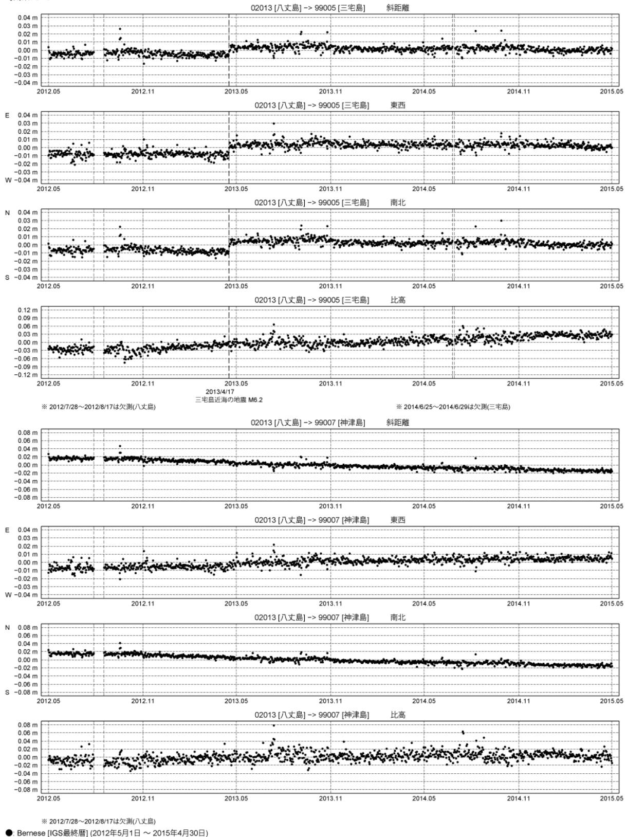
第 6 図 八丈島基点での三宅島および神津島の GPS 連続観測結果 (2012/5/1~2015/4/30)
