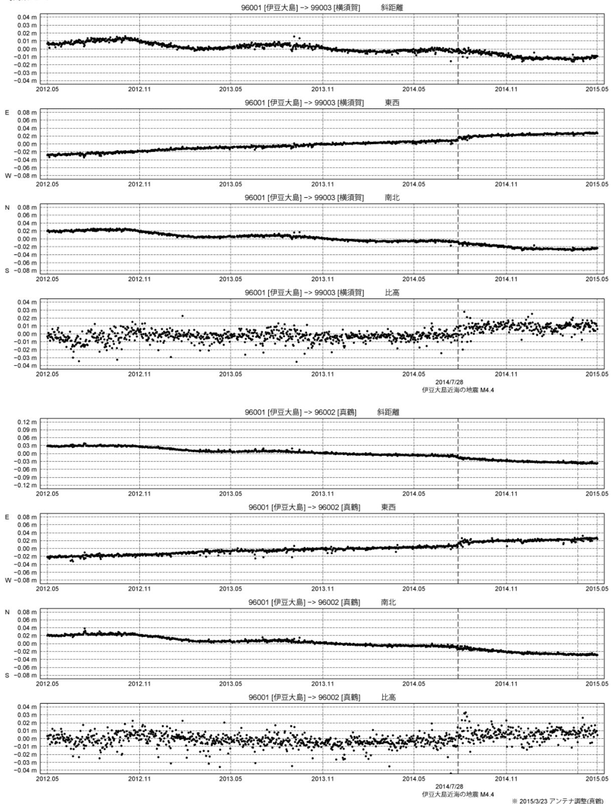
第 2 図 伊豆大島基点での横須賀および真鶴の GPS 連続観測結果 (2012/5/1~2015/4/30)
