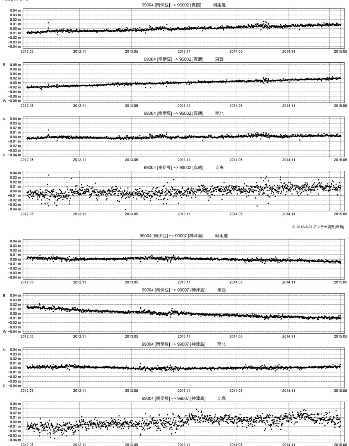
第 7 図 南伊豆基点での真鶴および神津島の GPS 連続観測結果 (2012/5/1~2015/4/30)
