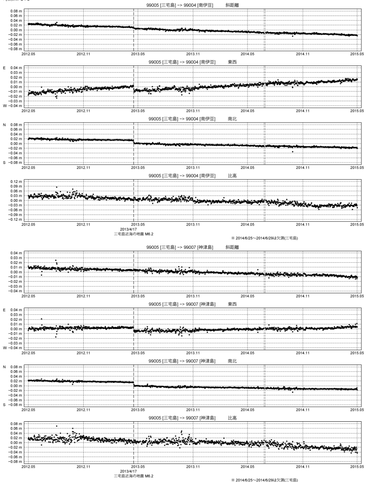
第 5 図 三宅島基点での南伊豆および神津島の GPS 連続観測結果(2012/5/1~2015/4/30)
