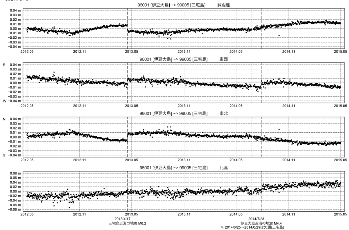
第 4 図 伊豆大島基点での三宅島の GPS 連続観測結果 (2012/5/1~2015/4/30)
