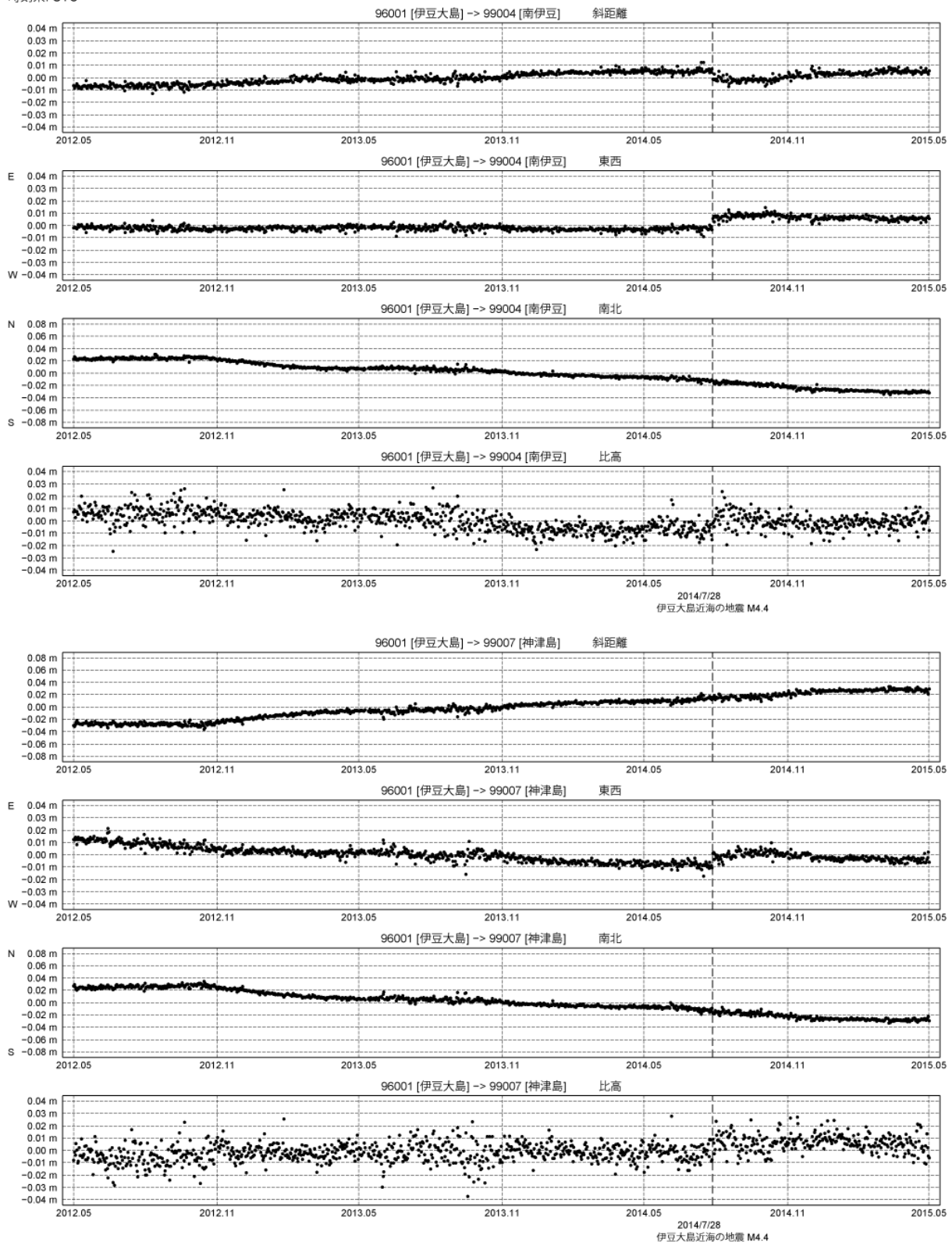
第 3 図 伊豆大島基点での南伊豆および神津島の GPS 連続観測結果 (2012/5/1~2015/4/30)
