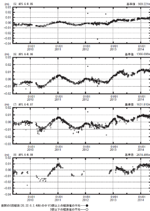
第4図 伊豆大島の光波測距観測結果(上段左：観測点配置図、上段右・下段左右：連続観測結果)
