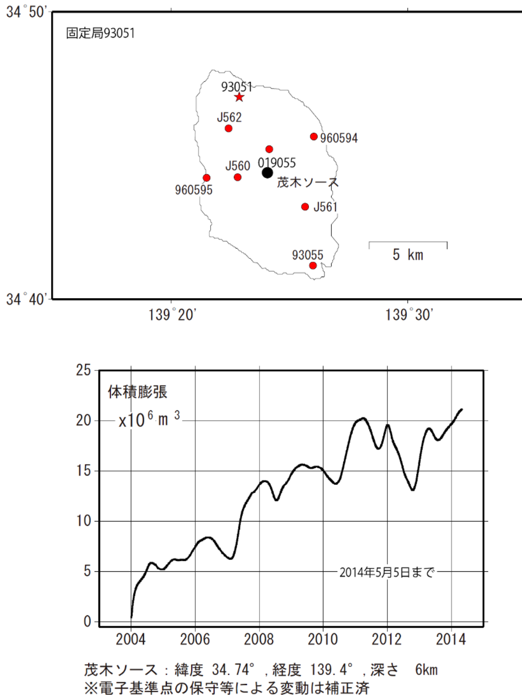
第5図 時間依存インバージョンの手法による伊豆大島の変動源の体積変化推定（上段：推定に用いた観測点（赤点）、固定点（星印）の配置と茂木ソースの位置（黒丸）、下段：推定された茂木ソース体積の時間変化）
