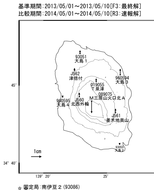
第3図 伊豆大島におけるGNSS連続観測点の変動ベクトル図(上段：水平変動、下段：上下変動、左列：2013年5月～2014年5月、右列：2014年2月～2014年5月)
