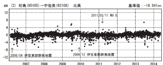
第 1 図 伊豆東部火山群周辺の GNSS 連続観測基線図 (上段左: 基線図、上段右: 保守履歴、下段: 3 成分 2006 年 3 月～2014 年 5 月)
