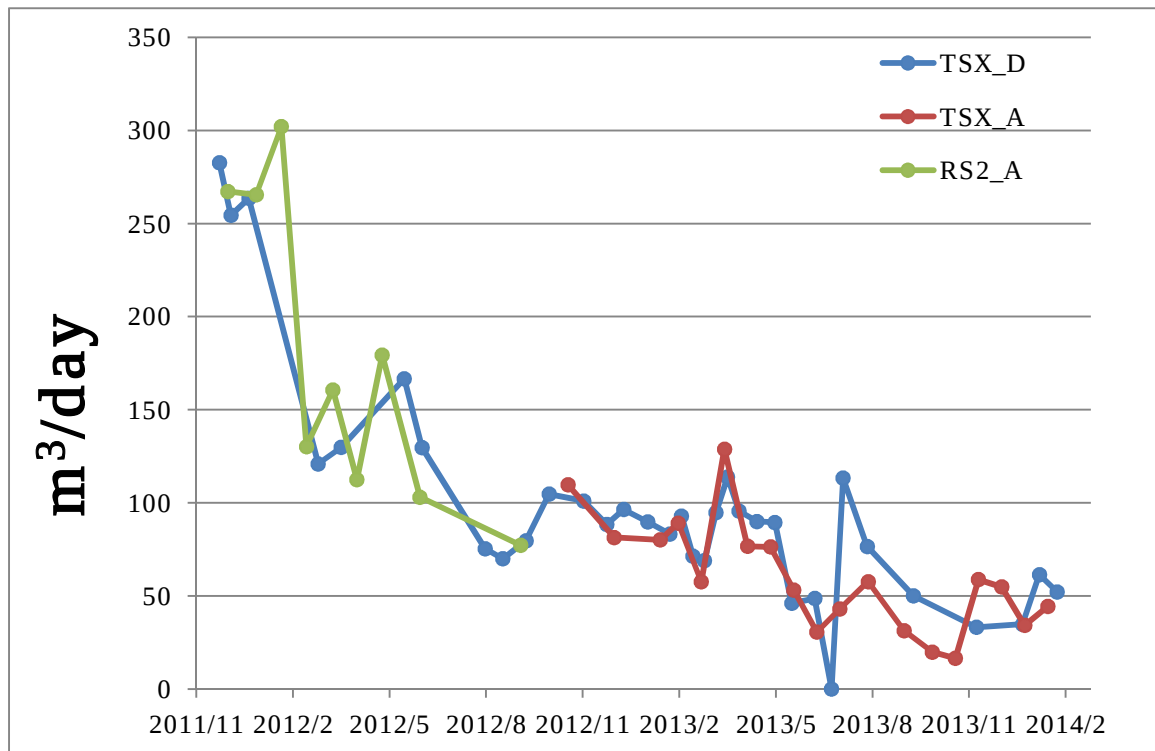
第 2 図. 火口内のスラントレンジ変化は上下変位のみによる，と仮定して求めた体積増加速度の時間変化。青線は TerraSAR-X (TanDEM-X)/南行軌道のデータから，赤線は TerraSAR-X (TanDEM-X)/北行軌道のデータから，緑線は RADARSAT-2 のデータからそれぞれ見積もられた値（※なお，隆起部分の地殻変動データのみを使用）。2013 年 6 月下旬に一度体積の増加が停止したが，その後再開した。
