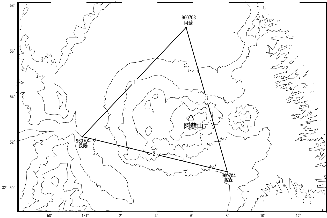
阿蘇山 GNSS連続観測基線図(1)
