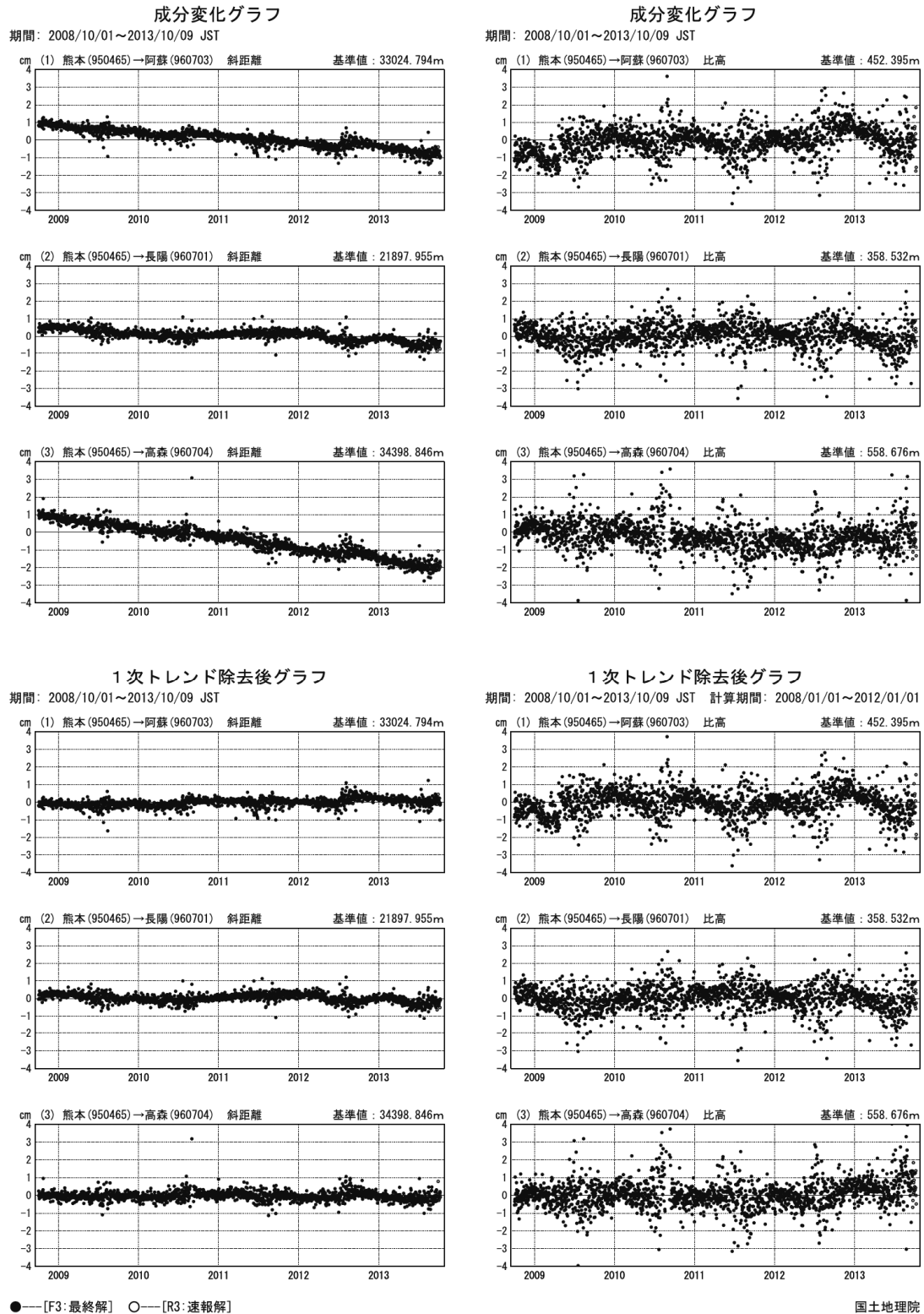
第4図 阿蘇山周辺のGNSS連続観測結果（上段左列：基線長、上段右列：比高、下段左列：一次トレンド除去・基線長、下段右列：一次トレンド除去・比高）（2008年10月～2013年10月）
