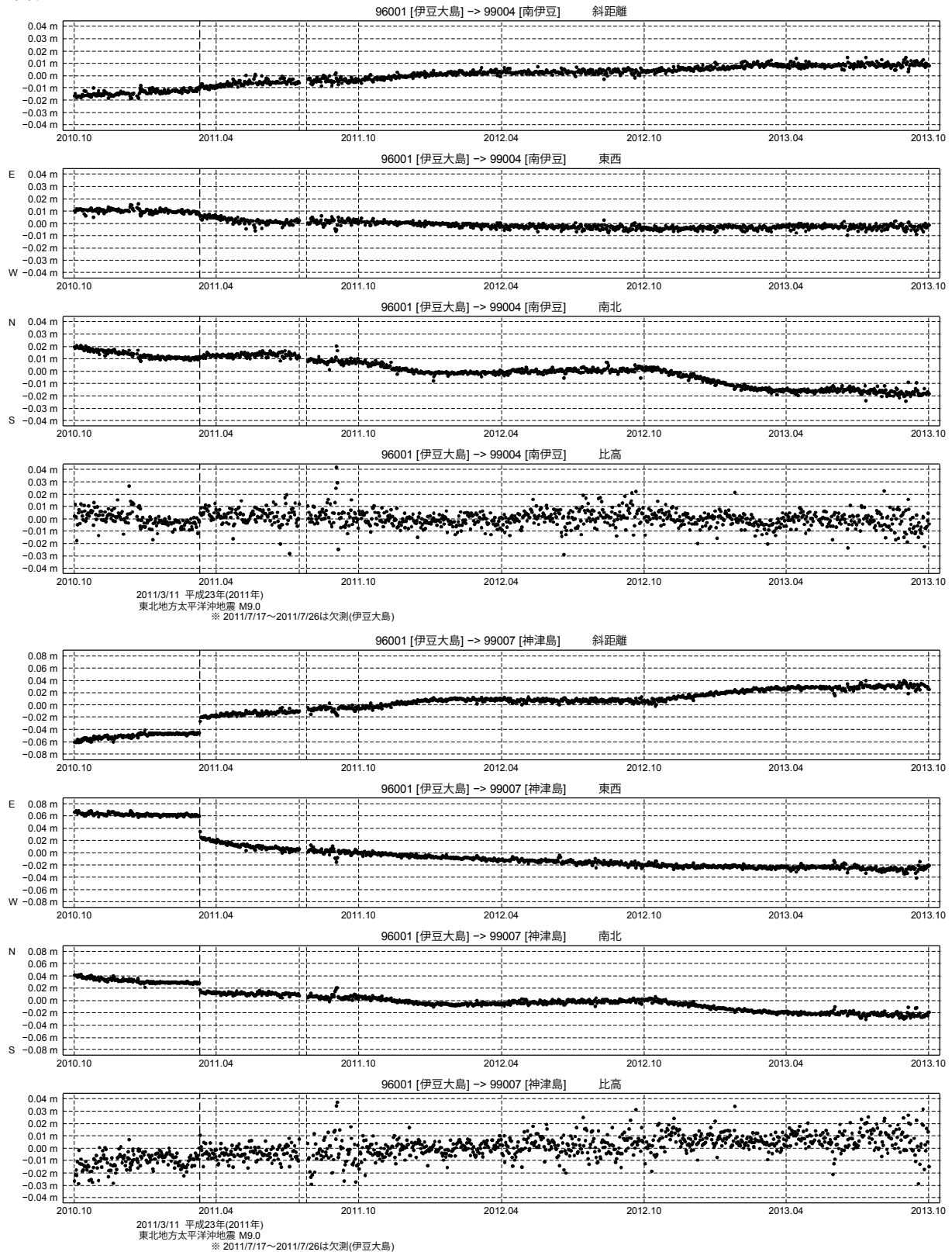
第 3 図 伊豆大島基点での南伊豆および神津島の GPS 連続観測結果 (2010/10/1~2013/9/30)
