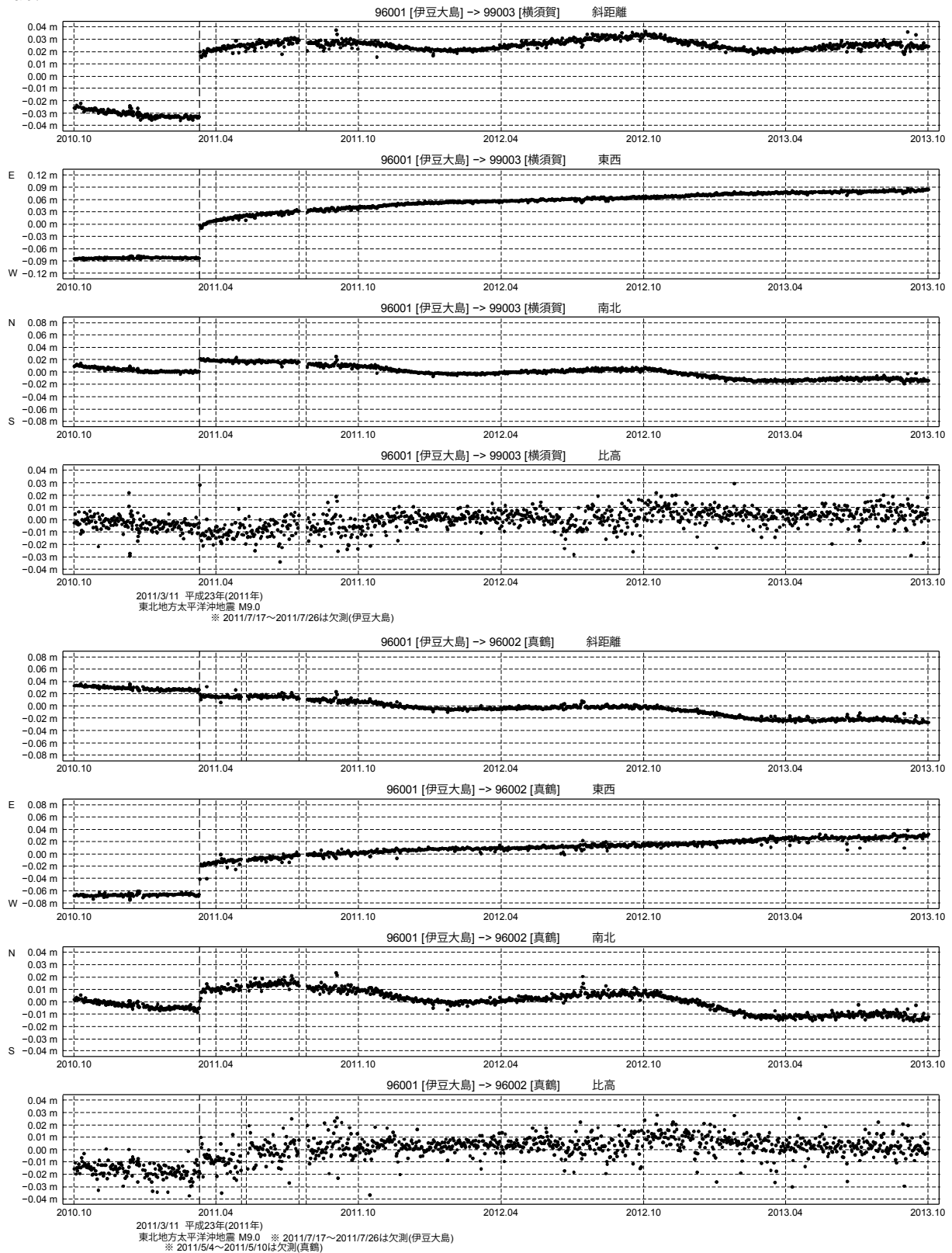
第 2 図 伊豆大島基点での横須賀および真鶴の GPS 連続観測結果 (2010/10/1~2013/9/30)
