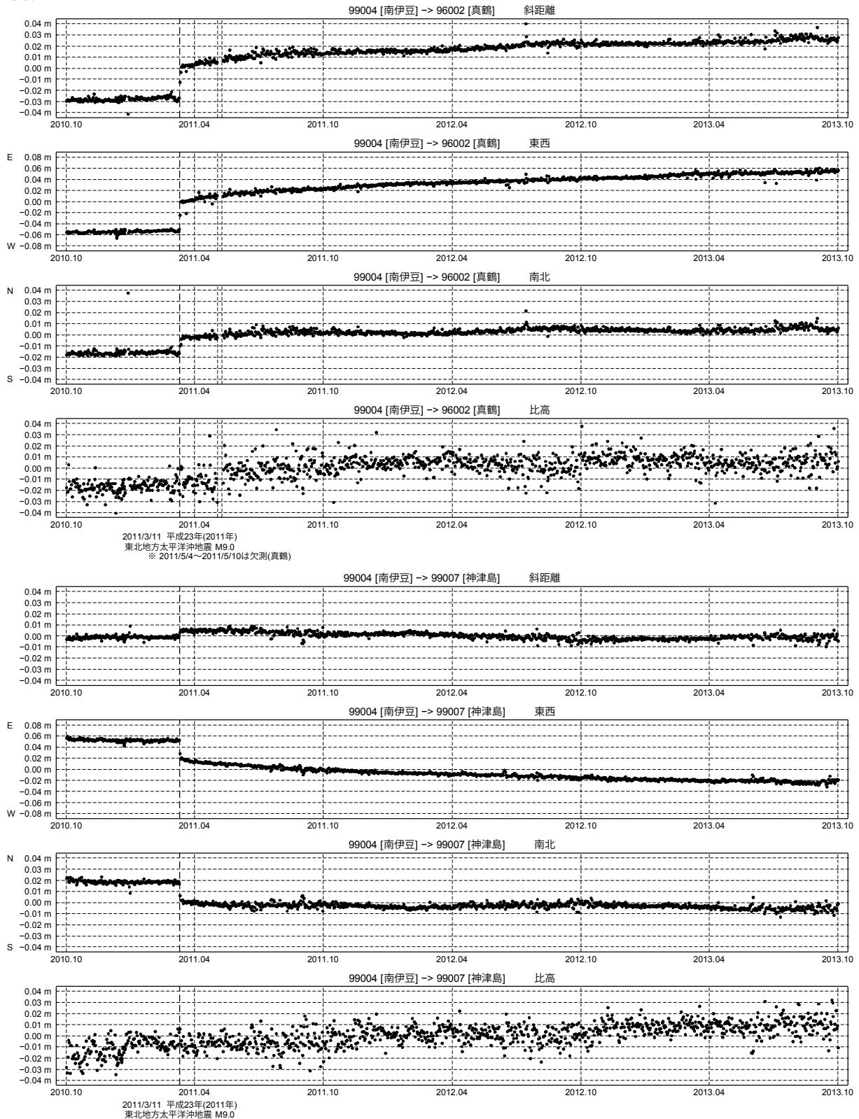
第 7 図 南伊豆基点での真鶴および神津島の GPS 連続観測結果 (2010/10/1~2013/9/30)
