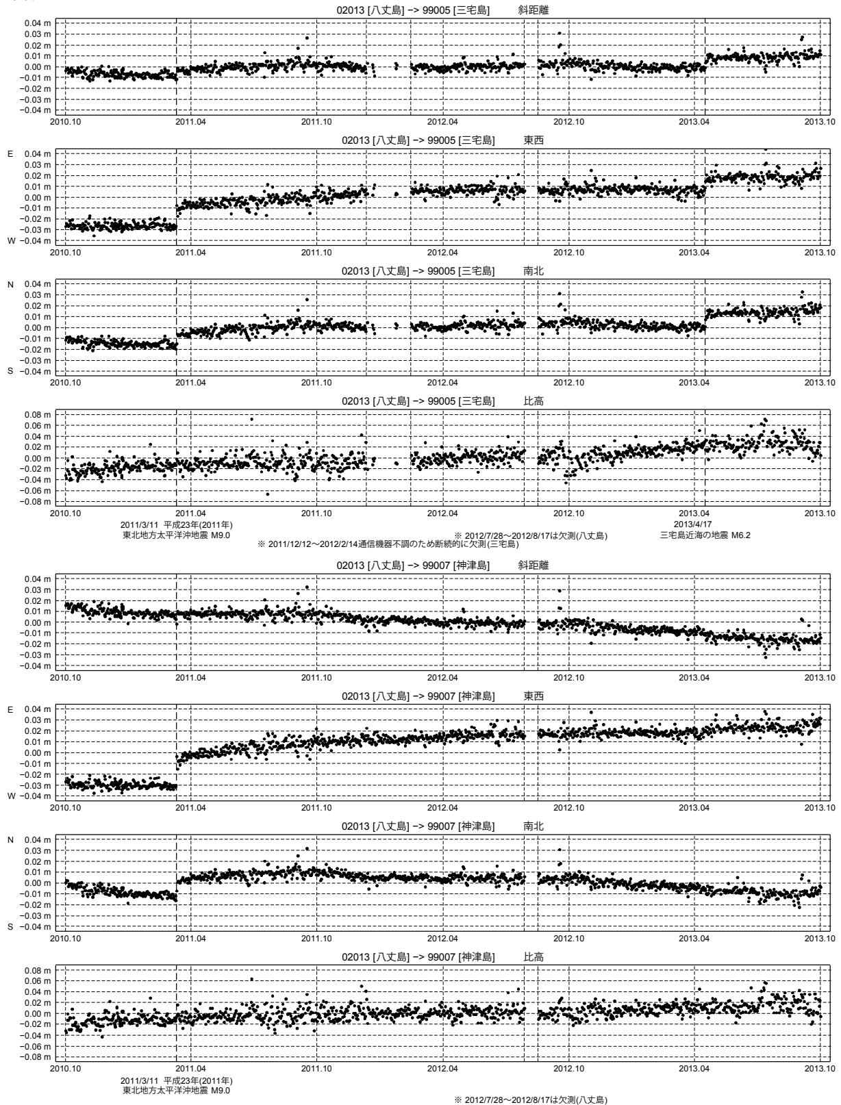
第 6 図 八丈島基点での三宅島および神津島の GPS 連続観測結果 (2010/10/1~2013/9/30)
