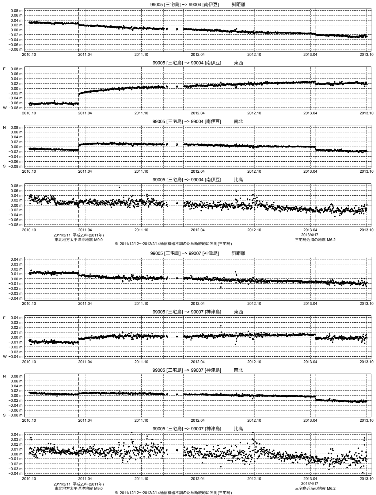
第 5 図 三宅島基点での南伊豆および神津島の GPS 連続観測結果 (2010/10/1~2013/9/30)
