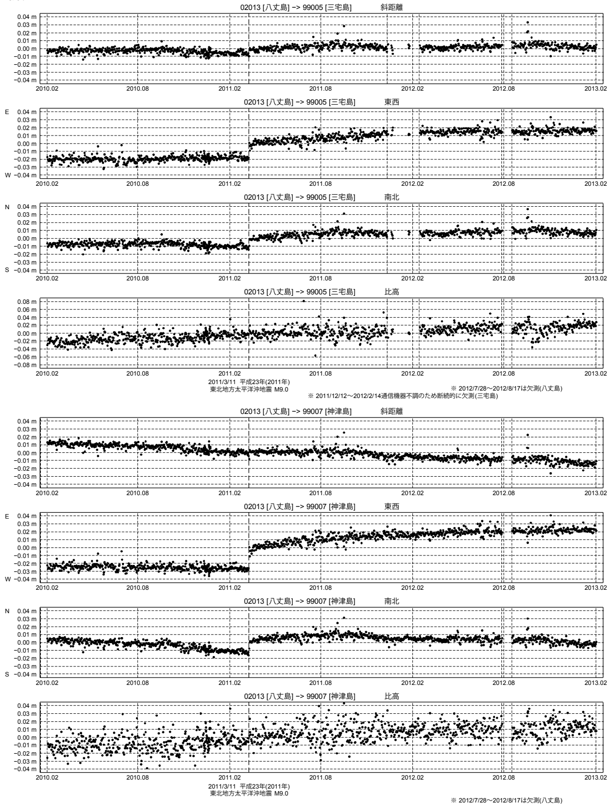
第6図 八丈島基点での三宅島および神津島の GPS 連続観測結果 (2010/2/1~2013/1/31)
