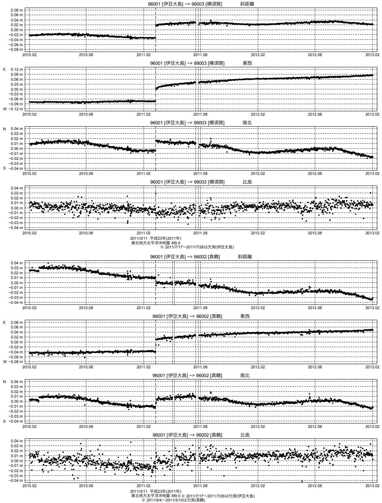
第2図 伊豆大島基点での横須賀および真鶴のGPS連続観測結果 (2010/2/1~2013/1/31)
