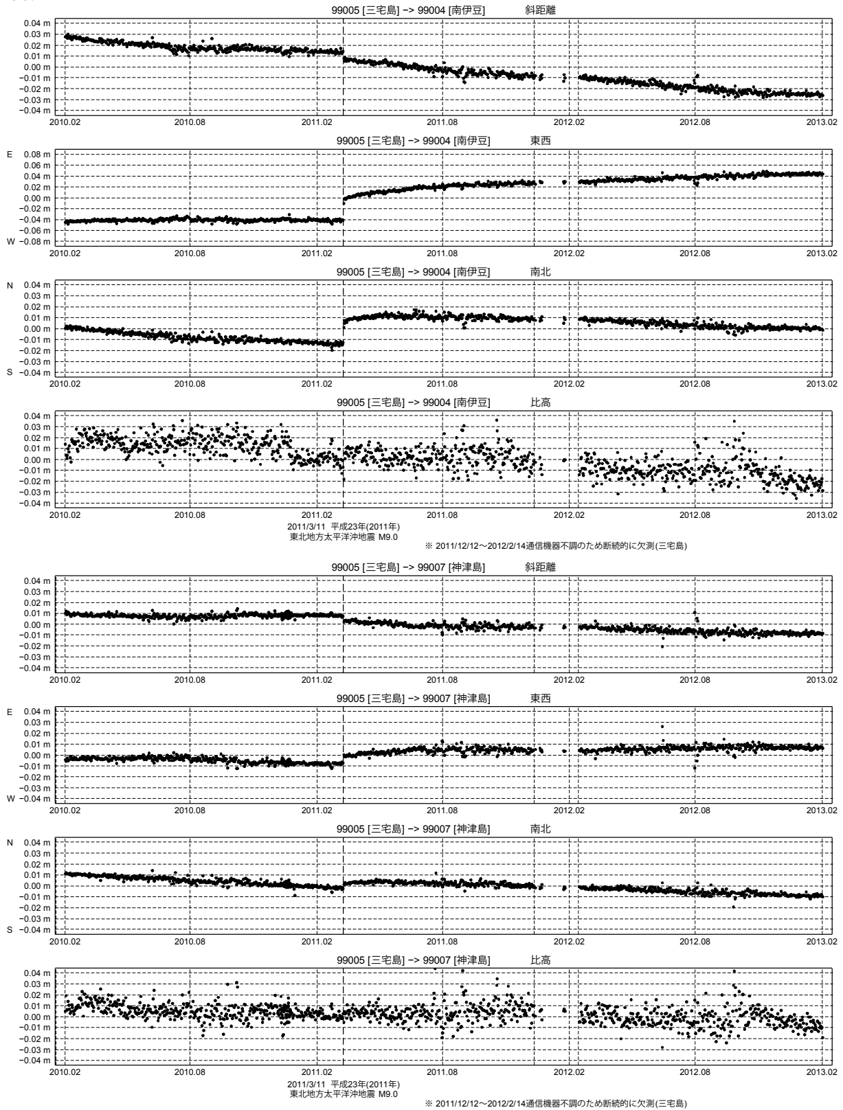
第5図 三宅島基点での南伊豆および神津島の GPS 連続観測結果 (2010/2/1~2013/1/31)
