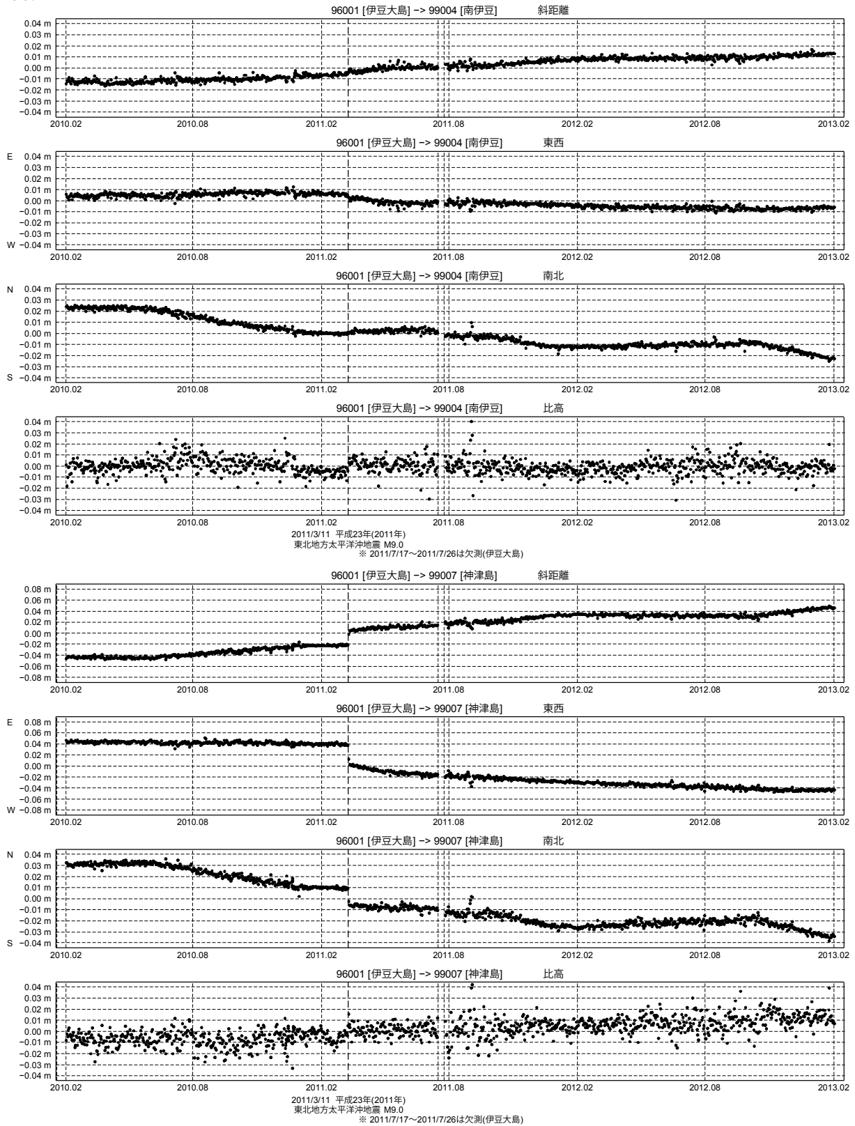
第3図 伊豆大島基点での南伊豆および神津島のGPS連続観測結果(2010/2/1~2013/1/31)
