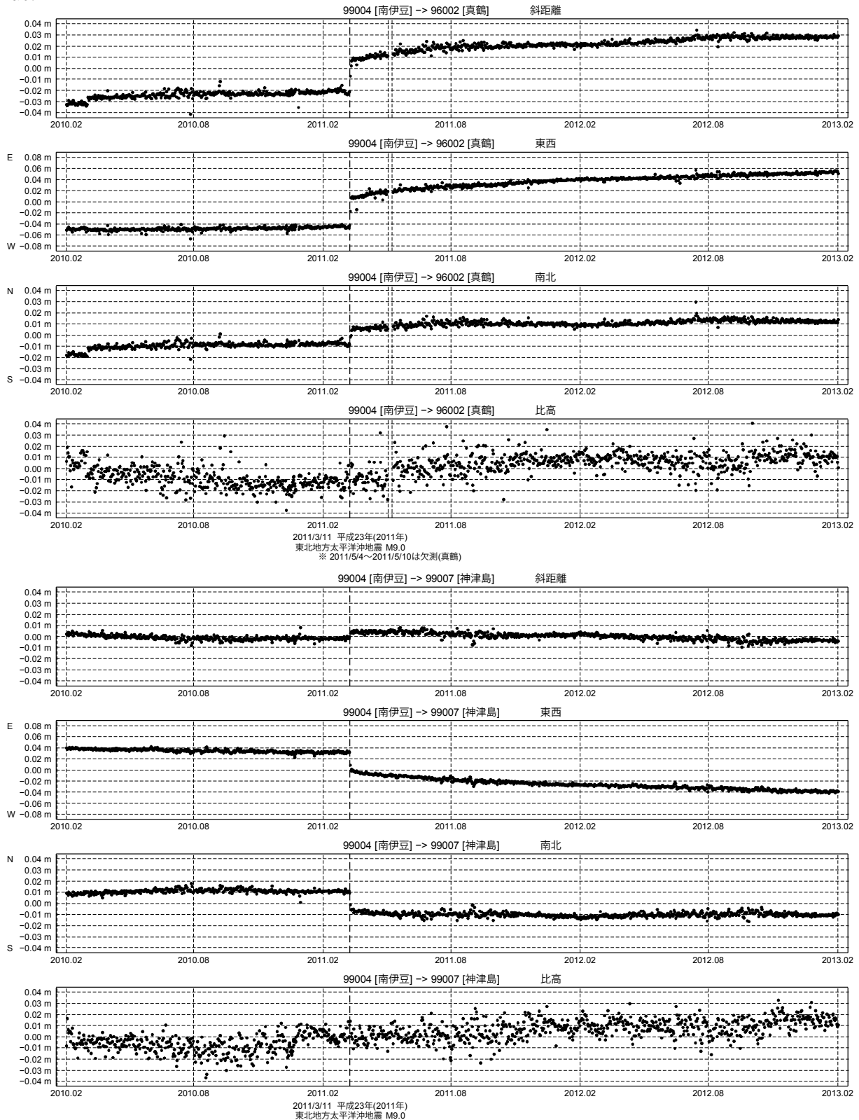
第7図 南伊豆基点での真鶴および神津島のGPS連続観測結果 (2010/2/1~2013/1/31)
