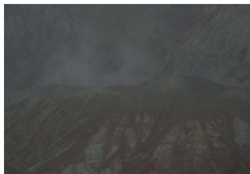
写真75 硫黄島
