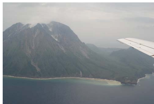
写真46 薩摩硫黄島
