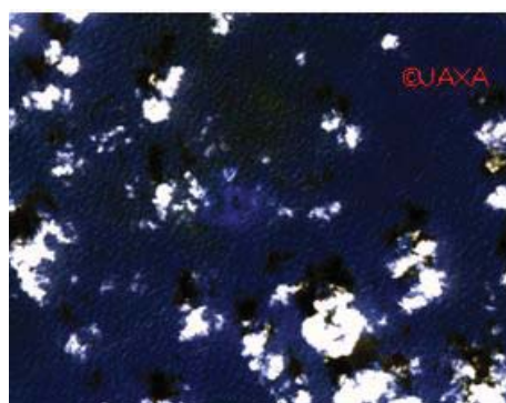
衛星写真1 福徳岡ノ場 Satellite Photo. 1 Fukutoku-Okanob
