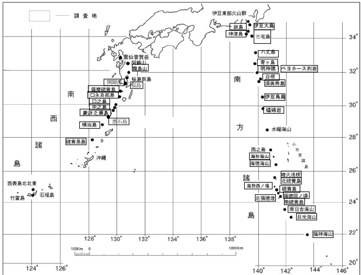
図 火山噴火予知調査位置 Fig. Submarine volcanoes and volcanic island
