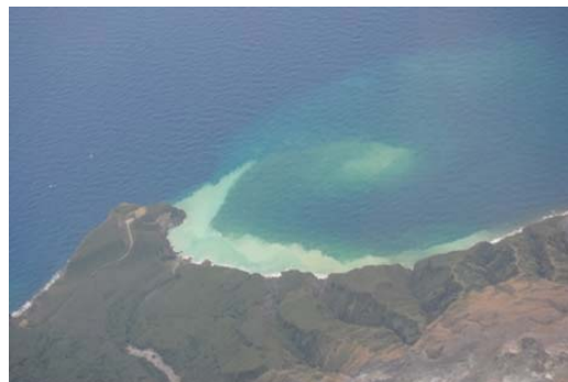
写真50 薩摩硫黄島
