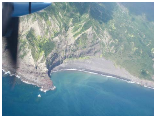
写真64 諏訪之瀬島
