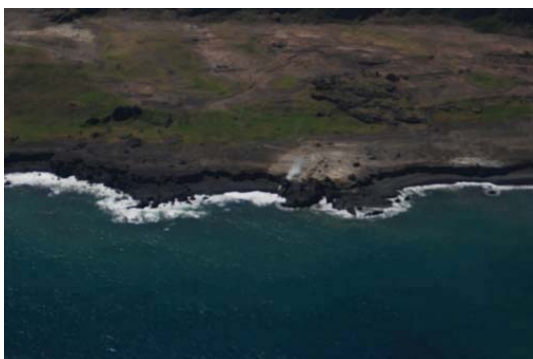
写真20 硫黄島
