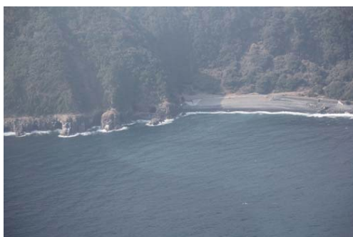
写真3 伊豆大島
