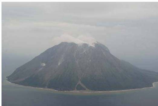
写真47 薩摩硫黄島
