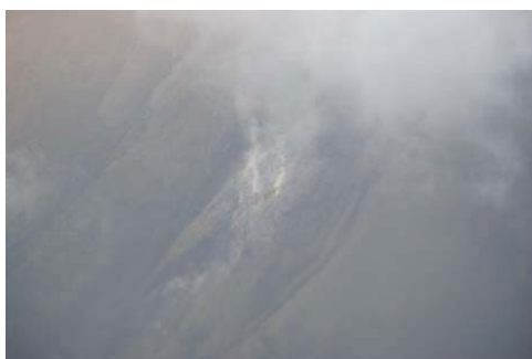
写真62 中之島
