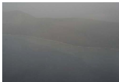
写真73 硫黄鳥島
