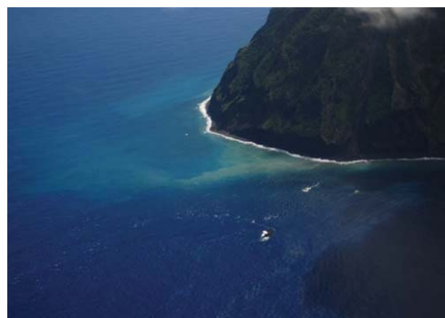
写真33 南硫黄島 Photo. 33 Minami-Ioto
