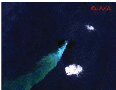
衛星写真5 福徳岡ノ場
