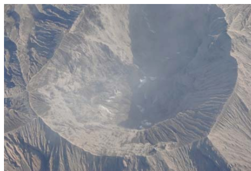
写真42 桜島 Photo. 42 Sakurajima
