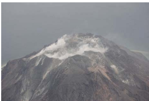
写真51 薩摩硫黄島
