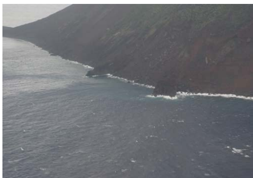
写真81 横当島
