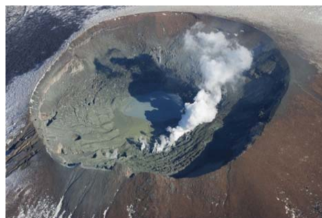
写真36 霧島 Photo. 36 Kiriima
