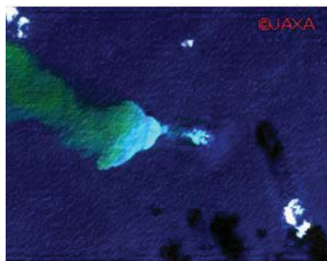
衛星写真4 福徳岡ノ場
