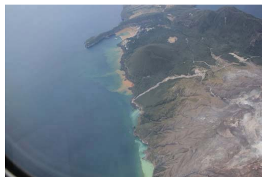
写真48 薩摩硫黄島
