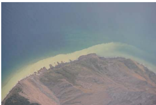
写真49 薩摩硫黄島
