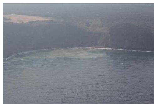
写真4 伊豆大島
