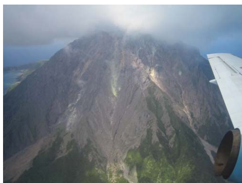
写真43 薩摩硫黄島
