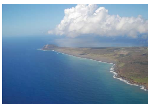
写真19 硫黄島 Photo. 19 Ioto
