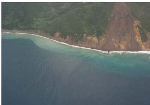
写真57 口之島
