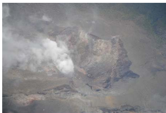
写真56 口永良部島
