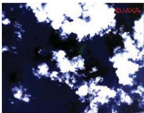
衛星写真2 福徳岡ノ場 Satellite Photo. 2 Fukutoku-Okanob
