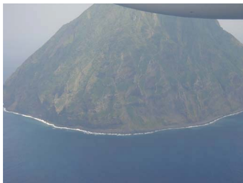
写真34 南硫黄島 Photo. 34 Minami-Ioto
