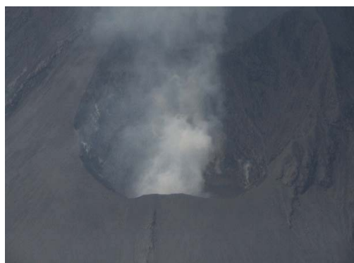
写真38 桜島 Photo. 38 Sakurajima
