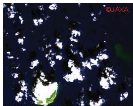
衛星写真3 福徳岡ノ場 Satellite Photo. 3 Fukutoku-Okanob
