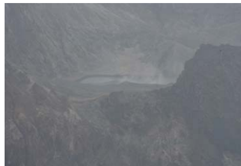
写真79 硫黄島
