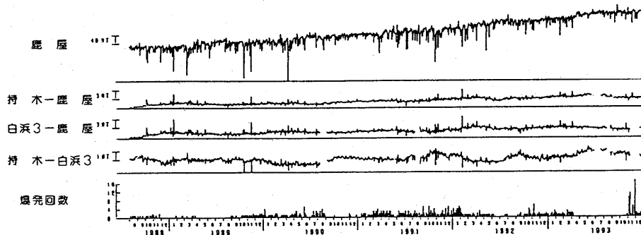
第 2 図 鹿屋の地磁気全磁力夜間値, および地磁気全磁力夜間値の相互差 (持木-鹿屋, 白浜3-鹿屋, 持木-白浜3) の日平均値変化。下段は日別爆発回数。
