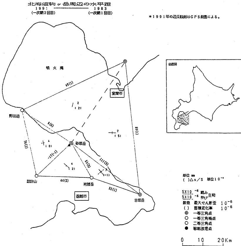
第1図 北海道駒ヶ岳周辺の水平歪
