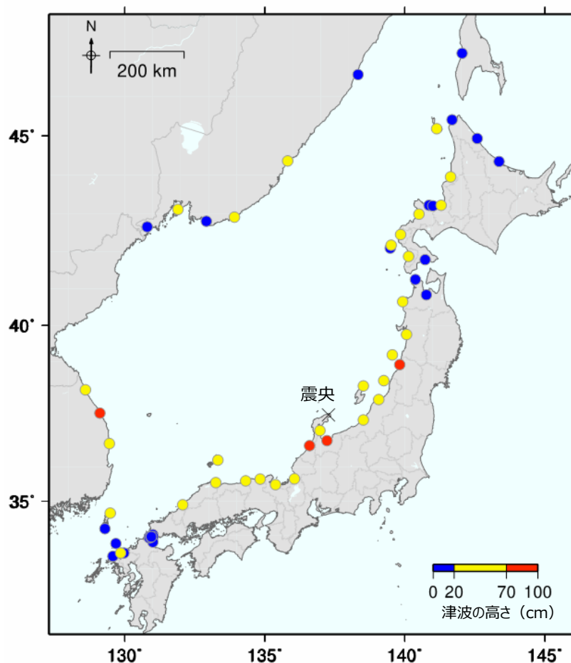
津波を観測した地点
