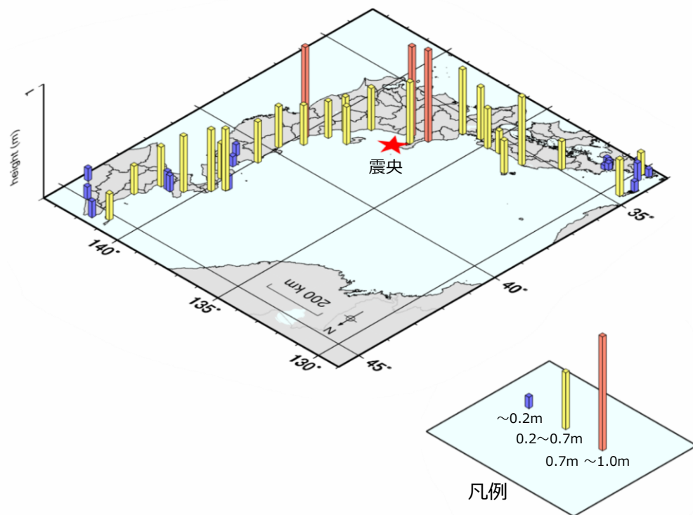
国内の津波観測施設で観測された津波の高さ
