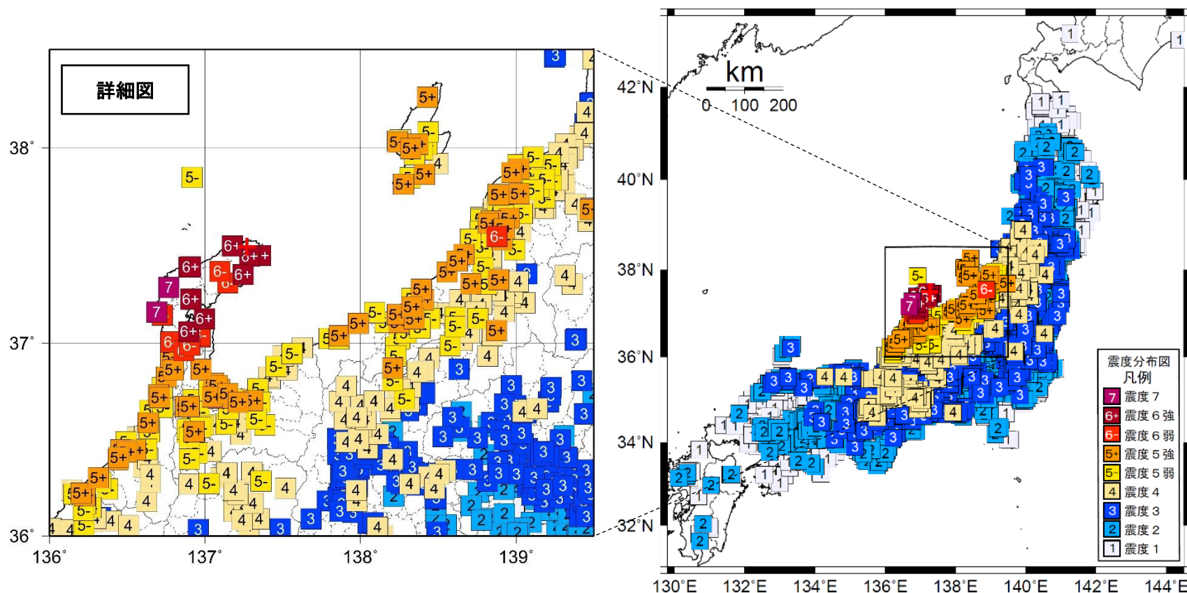
1月1日16時10分 石川県能登地方の地震（M7.6、深さ16km、最大震度7）の震度分布図 （+印は震央を表す）
