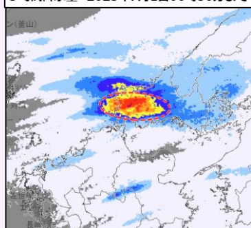
7/1九州北部地方における例
