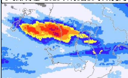
3時間降水量 2023年7月3日18時00分まで
