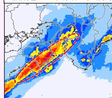
6/2近畿地方における例
