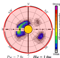
図2.8 二次元スペクトルから有義波高を算出する方法
