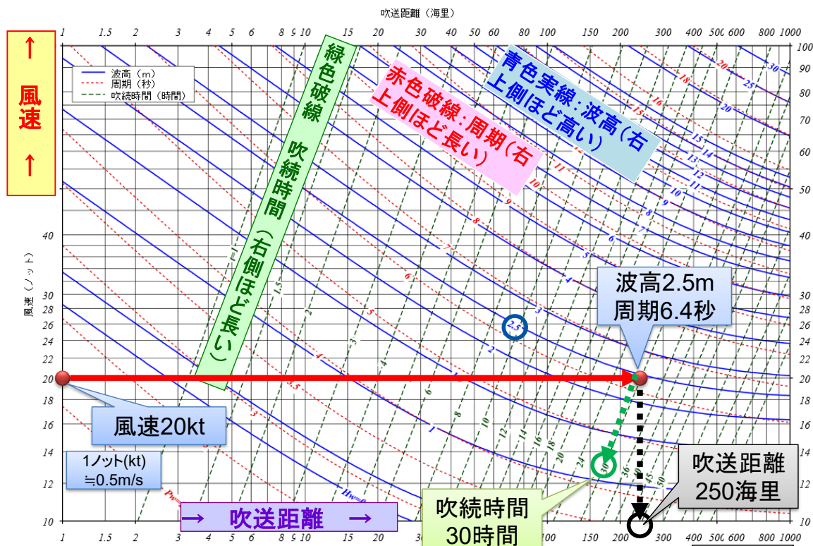
図4.2 Bretschneider(1970)に基づく風浪推算の図
