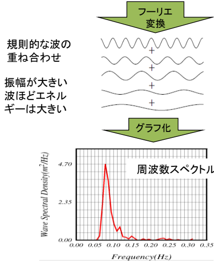
図2.5 スペクトルの求め方
