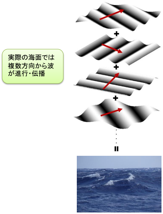
図2.6 二次元スペクトルの概念図
