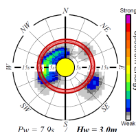
図2.9 二次元スペクトルから卓越周期を算出する方法
