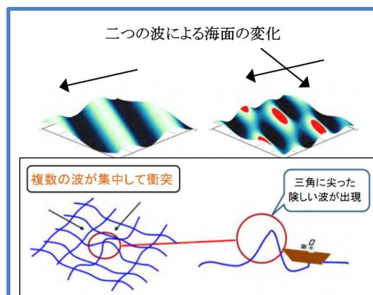
図付2.21 二つの波による海面の変化 (赤い部分は単一の波の最大より高い部分、図は内閣府(2017)を引用)
