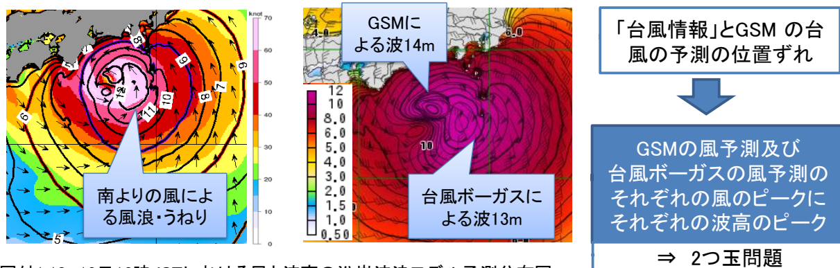
図付1.18 12日12時JSTにおける風と波高の沿岸波浪モデル予測分布図 12日00UTCを初期値とした3時間予測値(左)及び11日00UTCを初期値とした27時間予測値(右)
