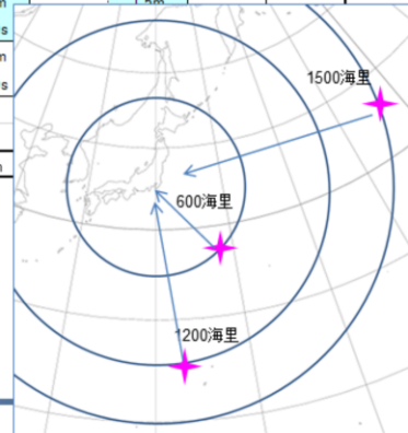
図4.5 うねりの推算早見表
