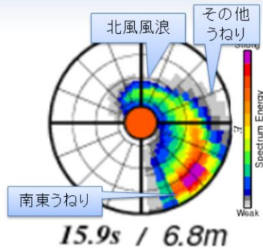
図付.1.14 2019/10/11 18UTC、室戸岬沖(図付.1.13の●地点)における沿岸波浪モデルの波浪二次元スペクトル図(18時間予報値)
