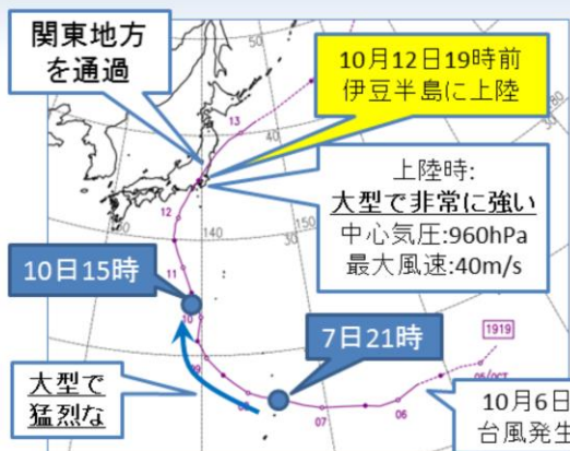
図付.1.1. 台風第19号経路図
