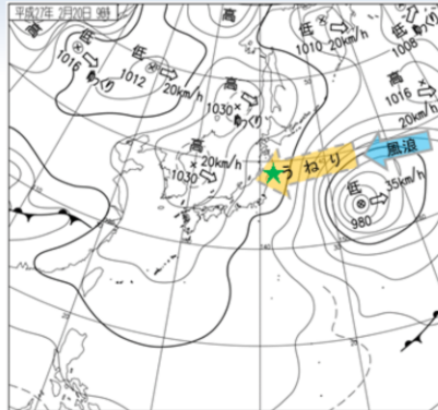
図3.4 2015年2月20日09時 実況天気図
