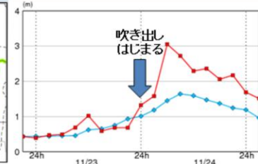
図3.8 和歌山南西沖GPS波浪計の波高の経過 赤:実況 青:予想
