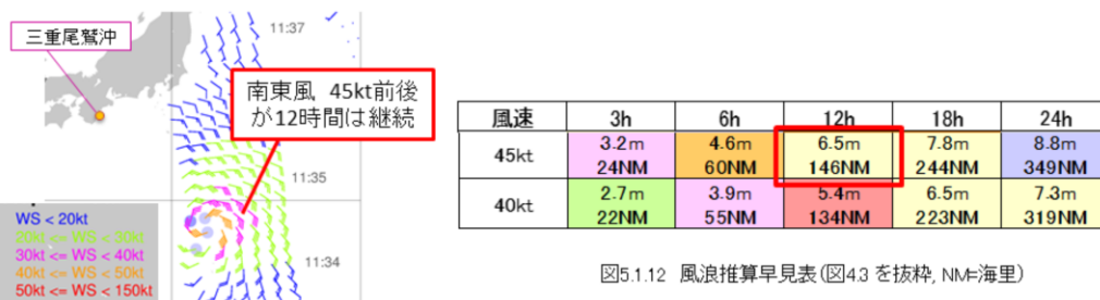
図5.1.11 Metop-Aによる海上風観測 (2019/09/07 11:30UTC頃)
