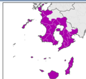
図5.2.3 ■ 波浪特別警報の発表地域
