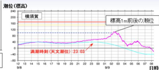
図5.1.6 潮位観測地点(横須賀)における天文潮位(青線)と観測の潮位(ピンク色の線) 縦軸は潮位(標高)で横軸は日時 赤い直線は高潮警報基準、黄色の直線は高潮注意報基準 (出典:横浜地方気象台, 東京管区気象台(2019))
