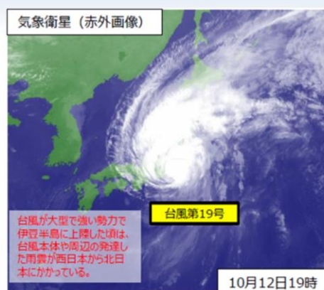
図付.1.2 10月12日19時の気象衛星による赤外雲画像
