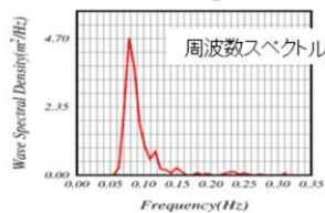
図2.5 スペクトルの求め方
