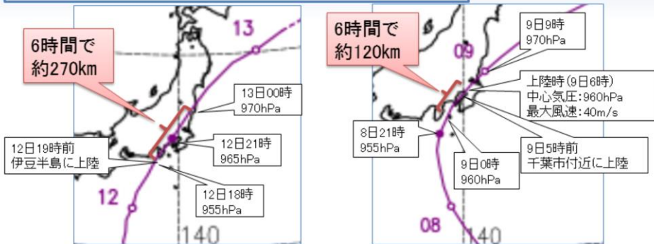
図付.1.23 台風第19号の台風経路図
