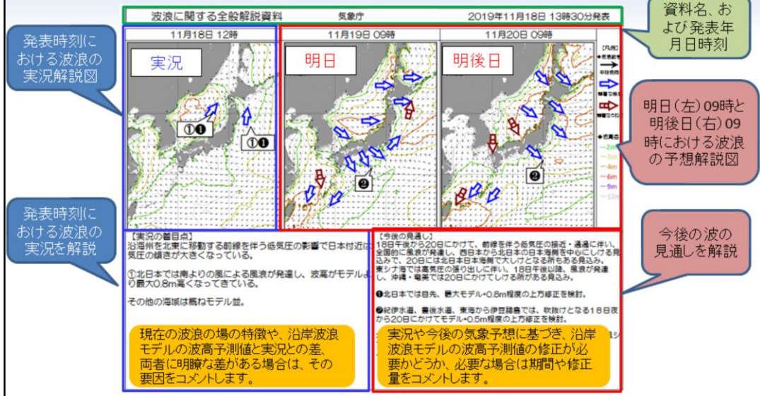
図4.1 波浪に関する全般解説資料の例
