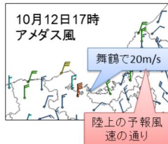
図付.1.11 10月12日17時のアメダス風速
