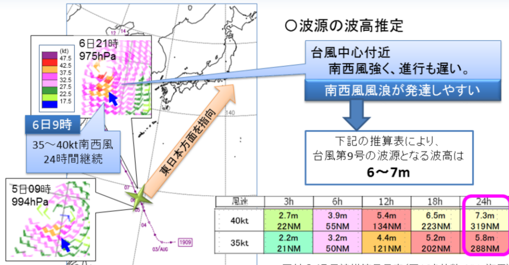
図付.2.16 台風第9号の経路とASCATによる海上風の観測
