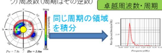
図2.9 二次元スペクトルから卓越周期を算出する方法
