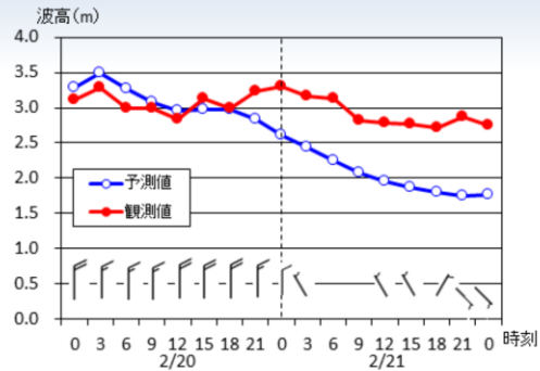
図3.5 宮城北部沖GPS波浪計(★)の波高と風向風速の経過
