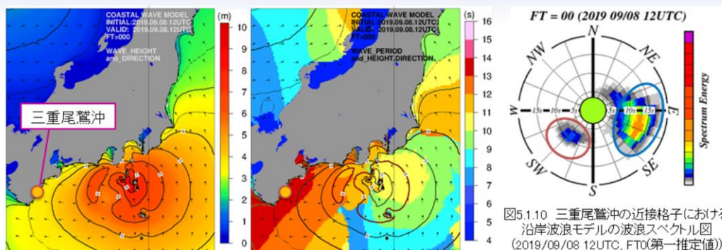
図5.1.9 沿岸波浪モデルの波高(左図)および周期(右図)分布図。ともに等値線は波高で矢印は波向。(2019/09/08 12UTC解析値)
