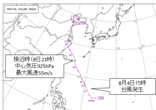
図付.2.1 台風第9号の経路図
