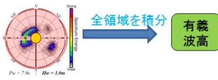
図2.8 二次元スペクトルから有義波高を算出する方法
