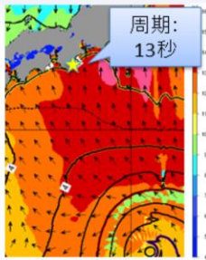
図付.2.10 10日00UTC沿岸波浪モデルFT=0:波高&周期
