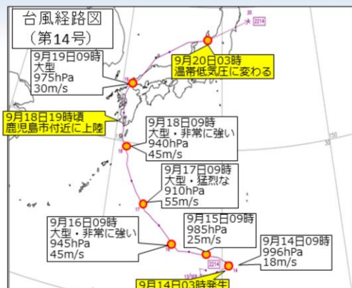
図5.2.1 台風第14号経路図
