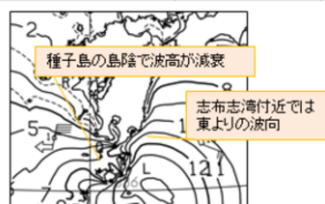
図5.2.5 9月18日9時の沿岸波浪実況図(等値線は有義波高)
