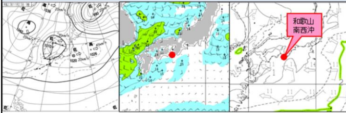
図3.6 2011年11月23日09時 実況天気図(左)、海上風予想図(中)、波浪予想図(右) 海上風予想図:矢羽は風向・風速、緑色は風速20kt台、水色は風速10kt台を示す。 波浪予想図:等値線は波高を表す。色付きの実線は1mごと、破線は0.5mごと。
