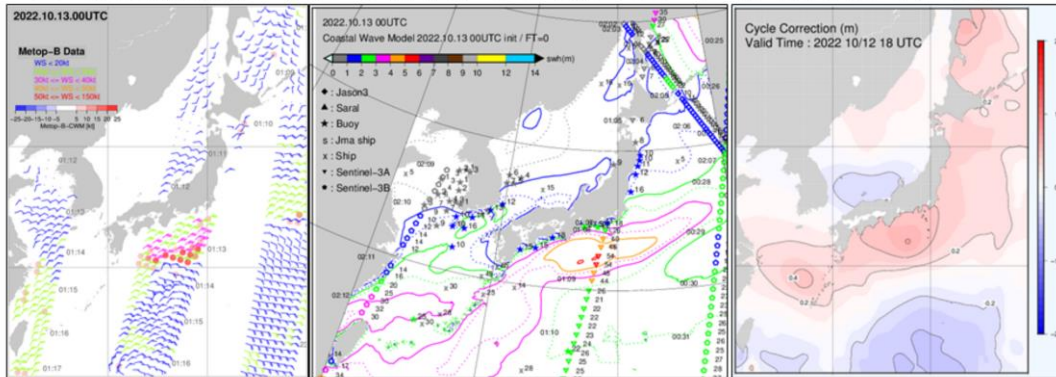
図3.1 衛星観測の風速(矢羽)と大気モデルの風速との差。図中の●の色が赤(青)いほど衛星観測の風速の方が大きい(小さい)。
