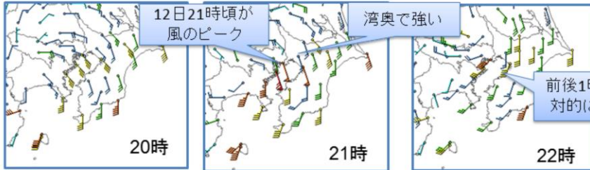
図付.1.28 関東地方周辺のアメダス風
