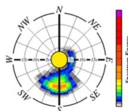
図5.1.21 沿岸波浪モデルの波浪スペクトル図(東京湾西部)(2019/09/08 18UTC, FT=0(第一推定値))
