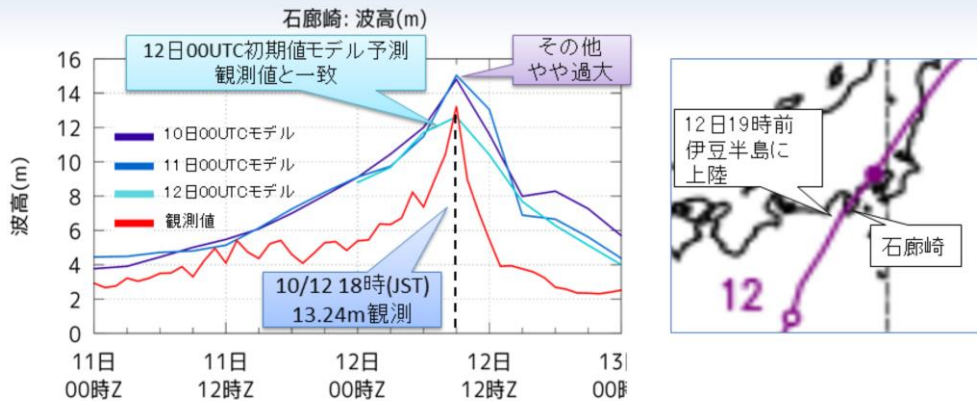
図付.1.21 台風経路図と石廊崎観測点の位置
