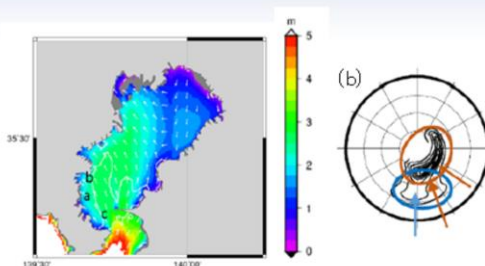
図5.1.20 9月9日0時における波浪の分布(左図)と地点bの波浪スペクトル図(下図)(出典:気象研究所(2020))
