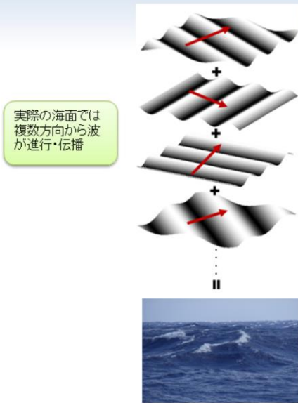
図2.6 二次元スペクトルの概念図
