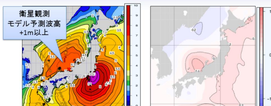
図付.1.6 2019年10月12日12UTCモデル波高第一推定値(左)とデータ同化による修正量(右)(左図の○は衛星観測データ、▽は沿岸波浪系データ、☆はブイデータ)
