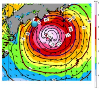
図付.1.13 2019/10/11 18UTC沿岸波浪モデル初期時刻の風と波高分布図
