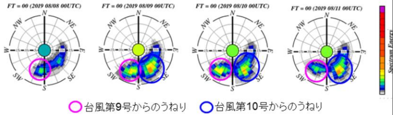
図付.2.11 図付.2.10★地点の波浪スペクトル(各初期値の第一推定値)
