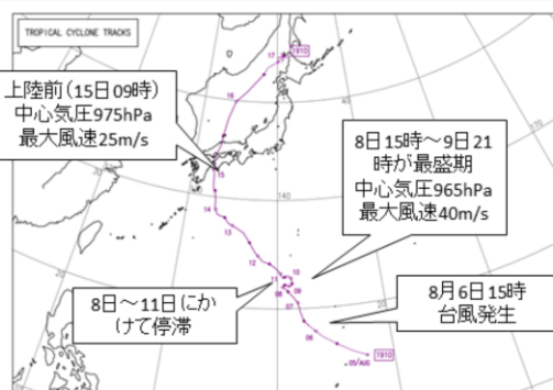
図付.2.2 台風第10号の経路図
