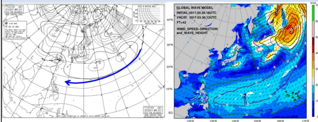
図3.9 2017年3月30日21時 予想天気図(左)、海上風・波高予想図(右)
