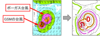
図3.13 波高の高い領域が二つに表現された台風の例
