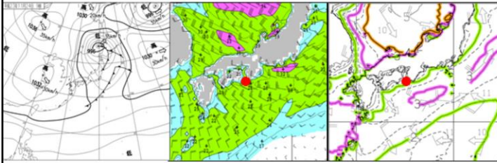
図3.7 2011年11月24日09時 実況天気図(左)、海上風予想図(中)、波浪予想図(右) 海上風予想図と波浪予想図の説明は図3.6と同じ(海上風予想図の赤色は風速30kt台)。
