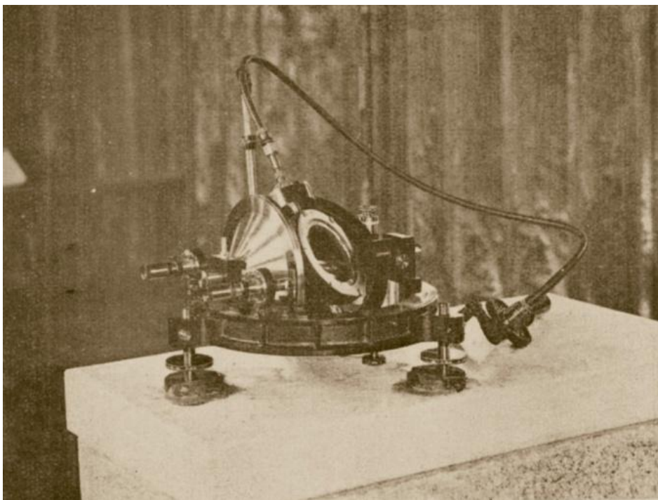
図 7-4-17 ウィルド・エーデルマン型アースインダクタ（I成分）（1913年～）
