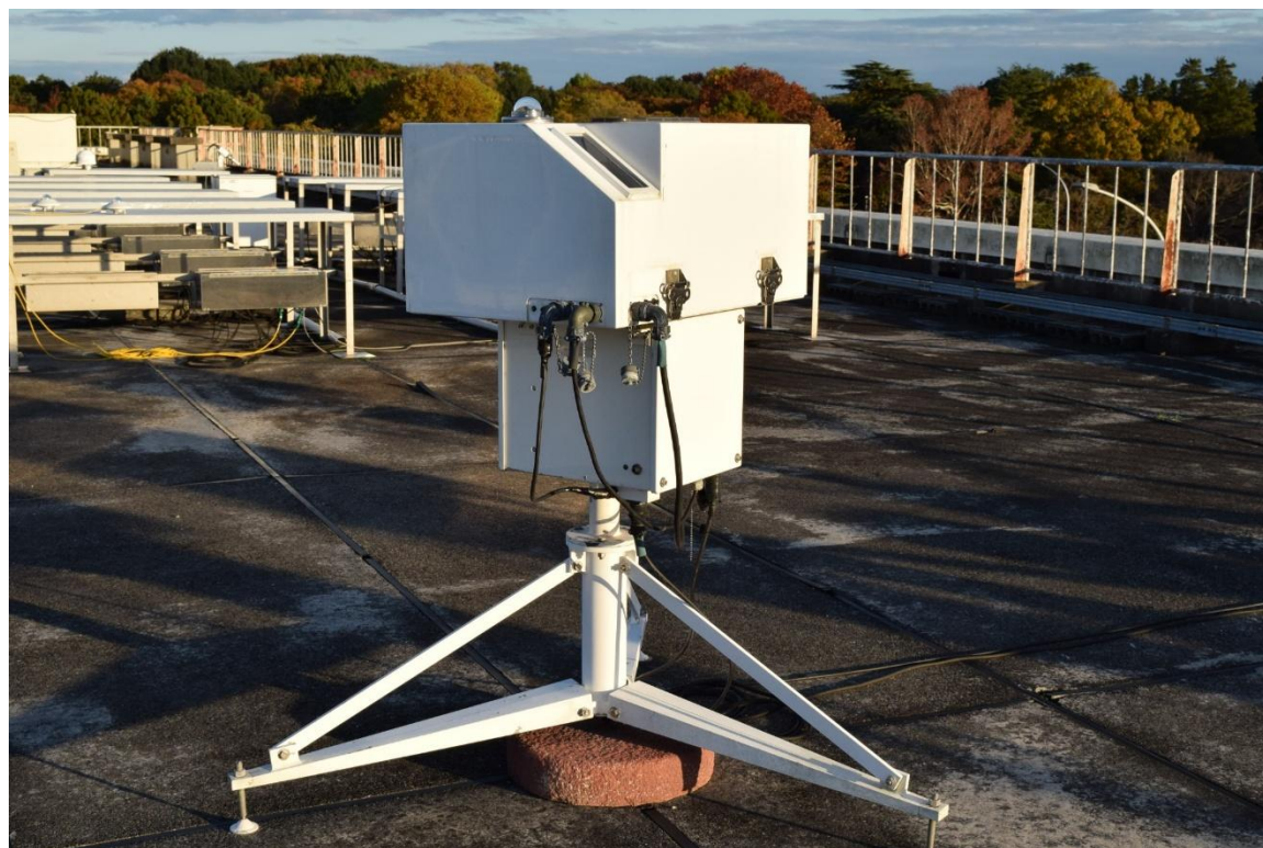
図 7-3-4 ブリュワー分光光度計
