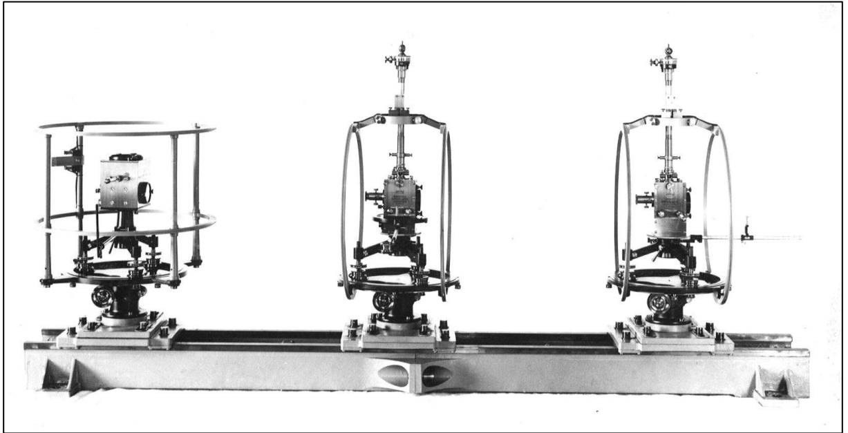
図 7-4-9 エッシェンハーゲン・シュミット型変化計（H、Z、D 成分）（1925年～） 鉛直分力（Z成分）（左）、偏角（D成分）（中）、水平分力（H成分）（右）
