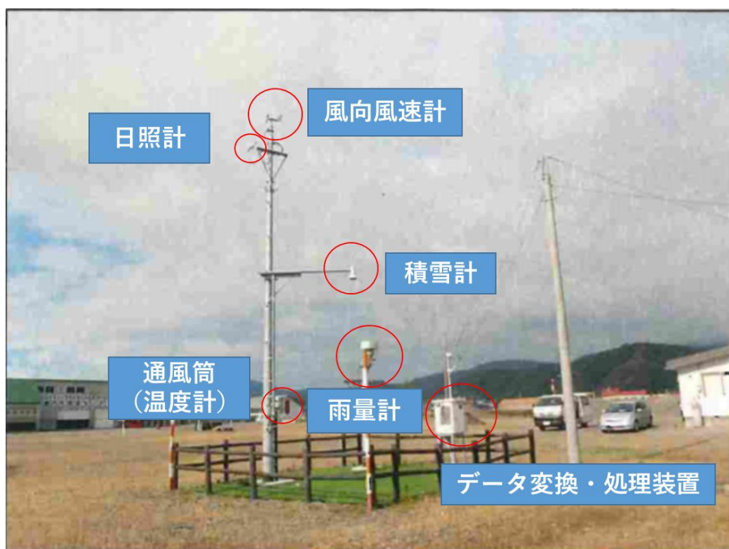
図 5-5-12 アメダス89型
