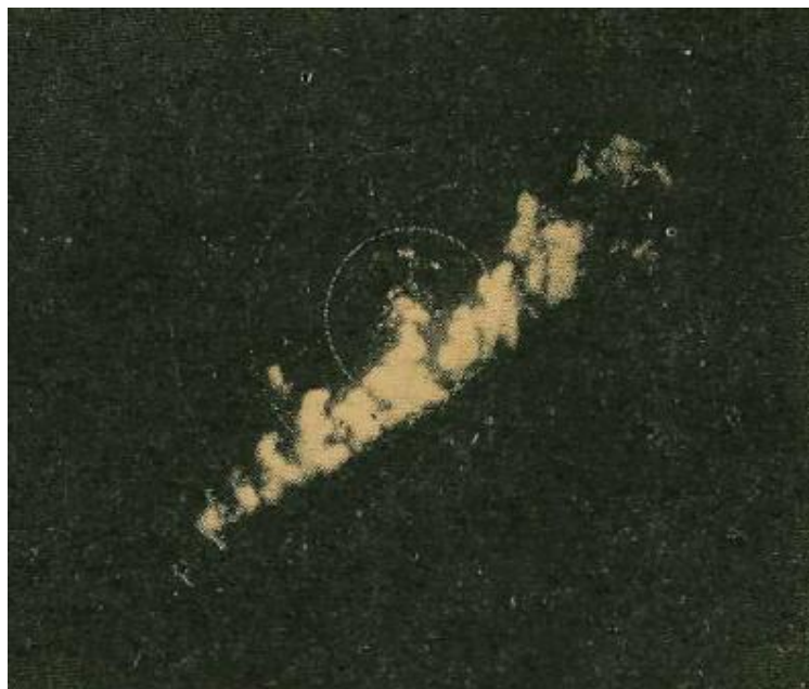
大阪レーダー1号機が 捉えた寒冷前線のエコー (昭和29年9月24日10時43分)
