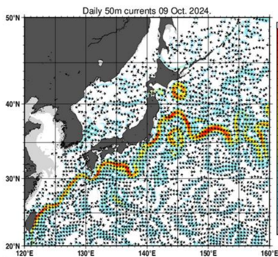
図1：日本近海の深さ50mの海流分布図（10月9日）
