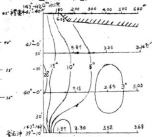
No. 4 自翻子冲至金石冲南北縱断水温图
