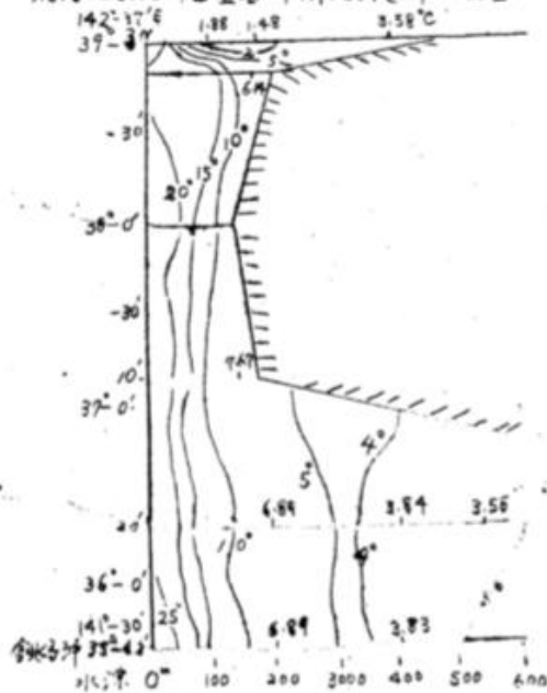
No. 4 自翻子冲至金石冲南北縱断水温图
