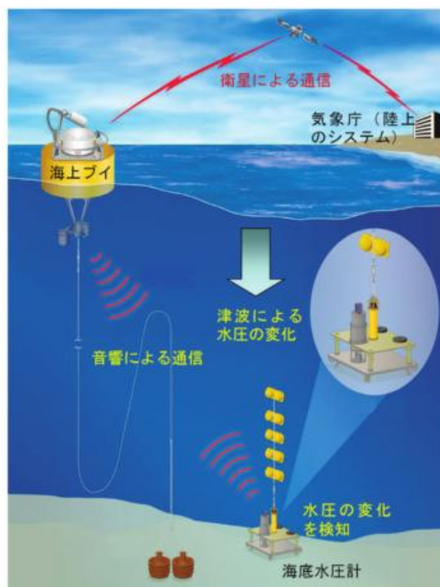
図 5-6-8 ブイ式海底津波計の海上設置作業（上）と観測システム概要（下） 東北地方太平洋沖の日本海溝東側に3基のブイ式海底津波計を整備。日本海溝付近で発生する津波を、既存の観測網に比べて場所によっては10分程度早く捉えることが可能。2012年12月から2016年8月までの期間、津波監視に活用された。
