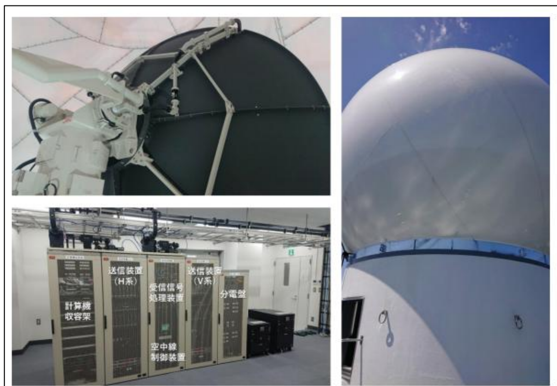
図 5-5-43 二重偏波気象ドップラーレーダー (主要装置の主な外観 日本無線株式会社製)
