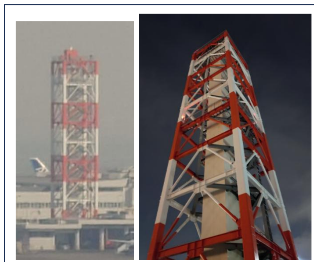
図 3-2-32 第三世代LIDAR （羽田空港1号機）
