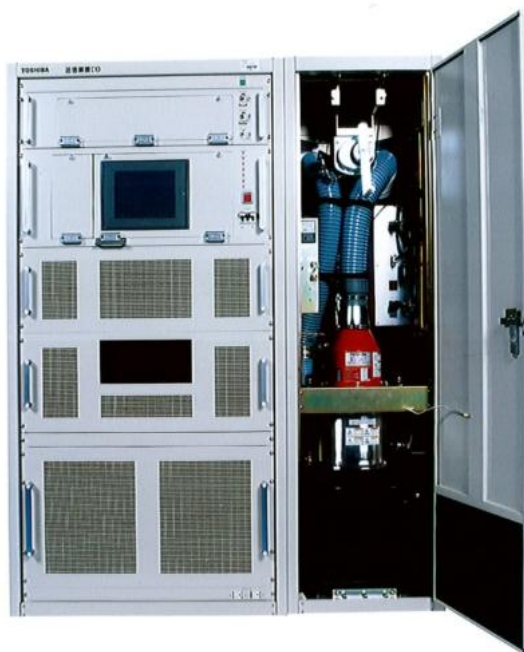
図 3-2-21 送信装置（クライストロン）
