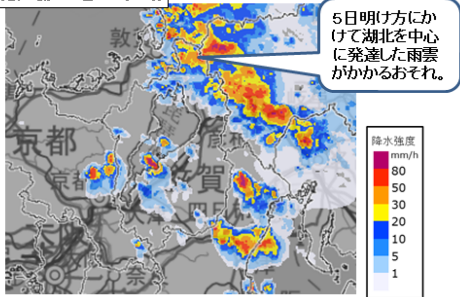
雨雲の動き 4日13時20分
