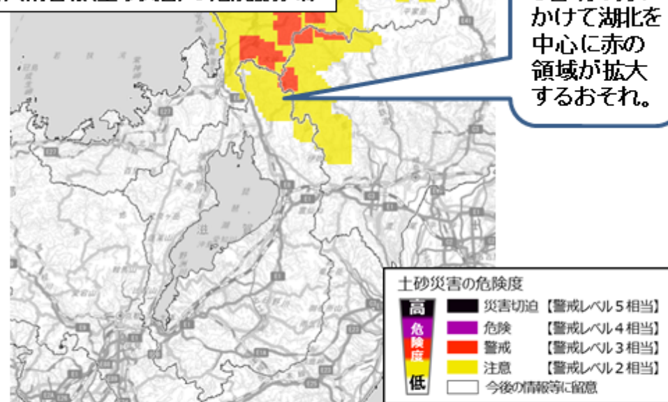
4日13時10分の土砂キキクル (大雨警報(土砂災害)の危険度分布)
