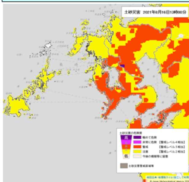
土砂キキクル 大雨警報(土砂災害)の危険度分布 16日13時00分
