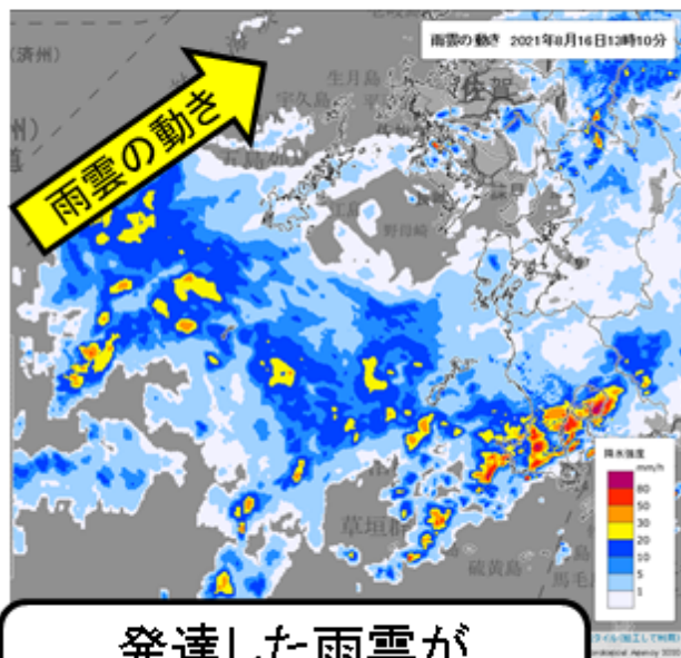
雨雲の動き 16日13時10分
